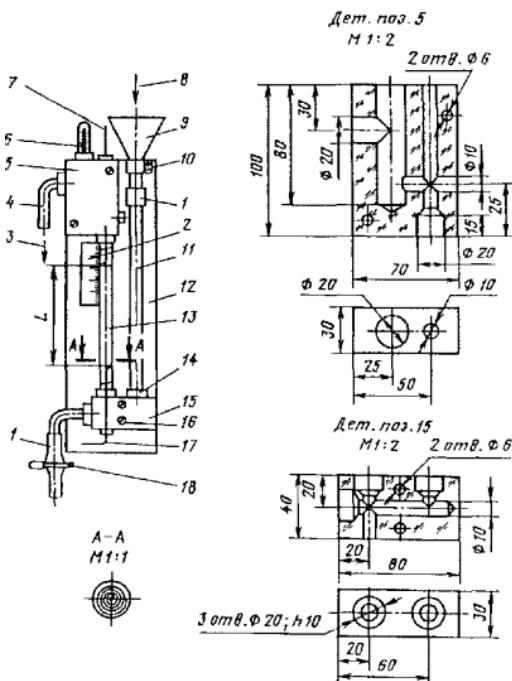
Датчик солемера:
