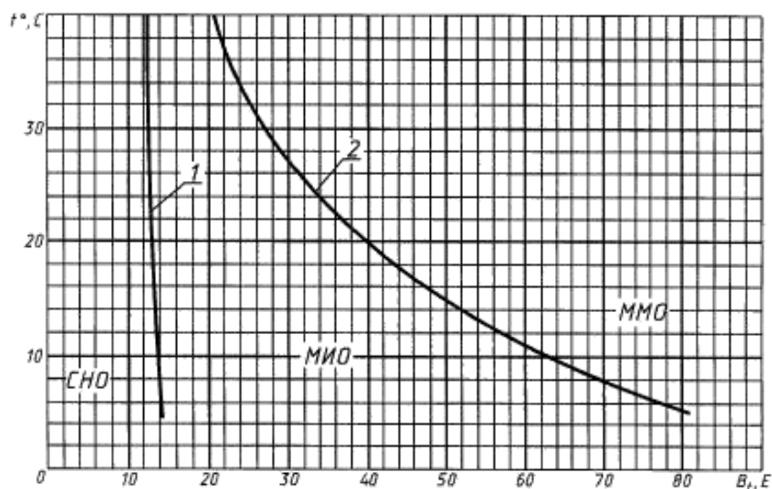
Зависимость условной вязкости от температуры
