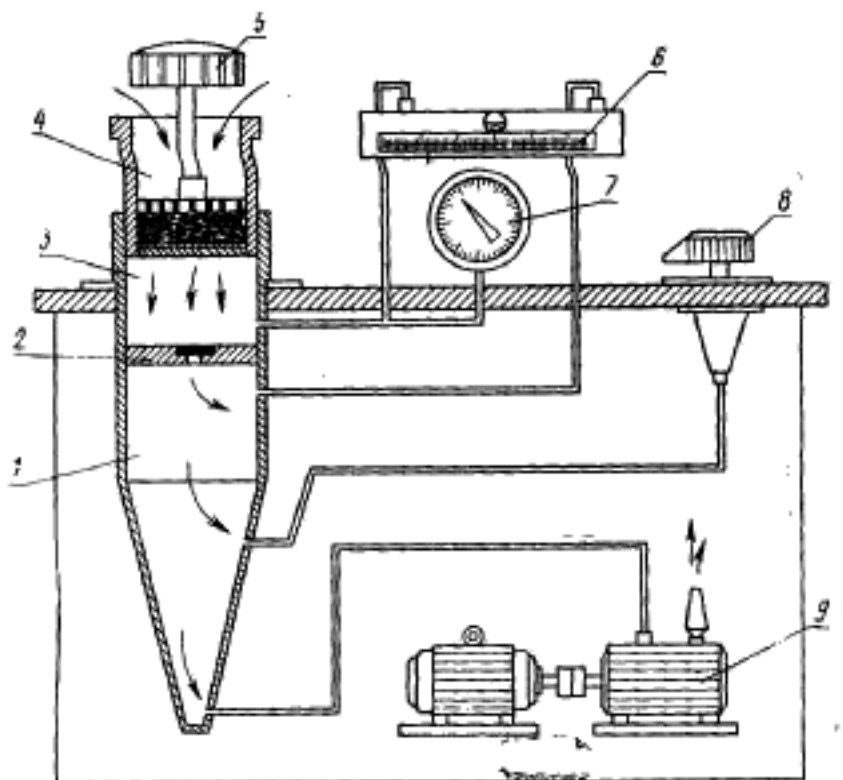
1 — камера 3; 2 — диафрагма; 3 — камера 2; 4 — камера 1; 5 — подпрессовывающее устройство; 6 — тягонапоромер; 7 — вакуумметр; 8 — дроссель; 9 — вакуум-насос
