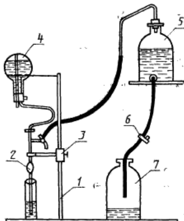
1 — штатив; 2 — пипетка вместимостью 25 \text{ см}^3 ; 3 — упор; 4 — колба для промывания пипетки; 5 — аспиратор; 6 — зажим; 7 — стаканчик
