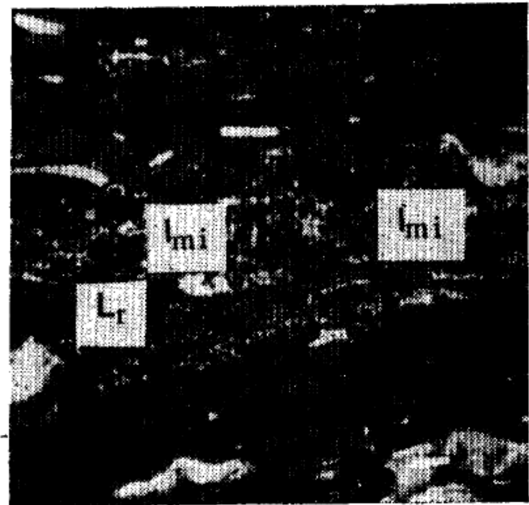
I_{mi} — микроинит; L_r — резинит
