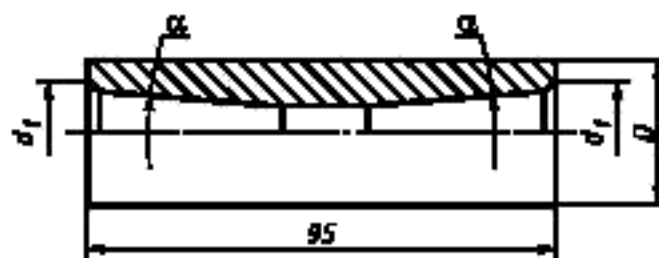
Рисунок 3 — Соединительная муфта
