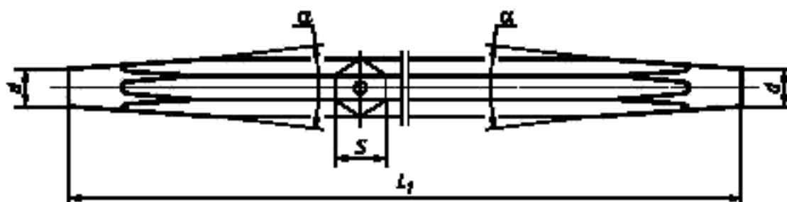
Рисунок 2 — Буровые и удлинительные штанги с конусом
