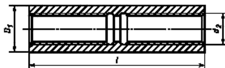
Рисунок 6 — Соединительная муфта
