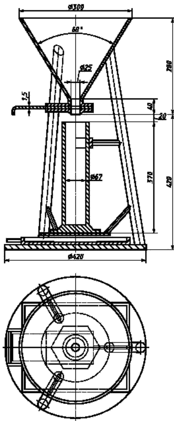
Аппарат для определения насыпной плотности удобрений
