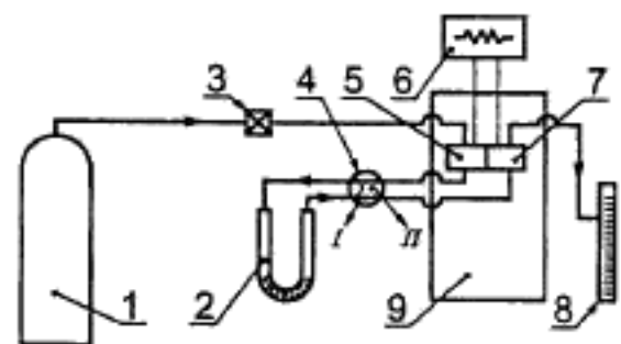
Схема установки
