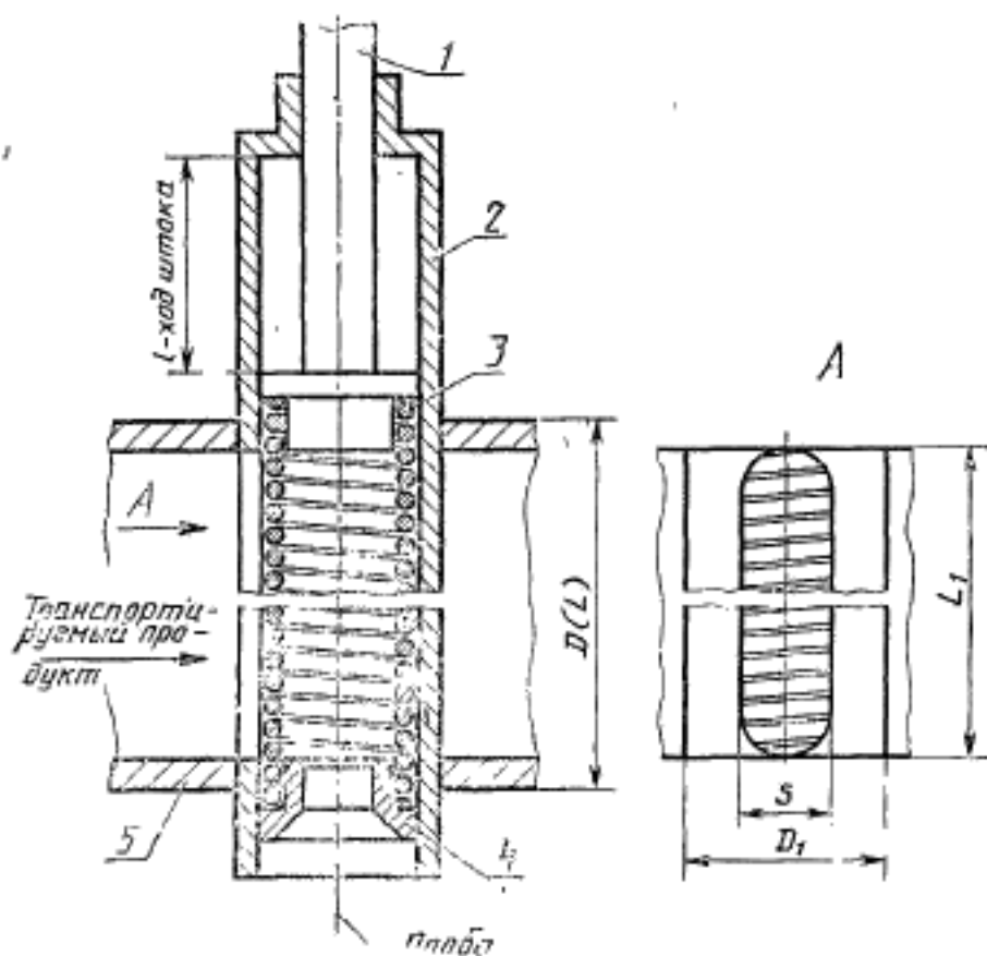
1 — шток; 2 — труба; 3 — пробоотбирающий элемент; 4 — втулка; 5 — трубопровод
