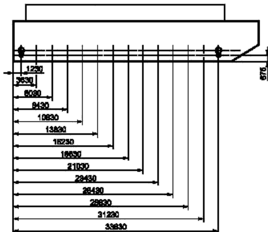
Рисунок 2 — Расположение бортовых гнезд
