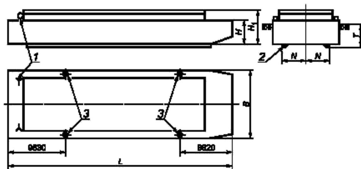
1 — присоединение шлангов подачи CO 2 , 2 — направляющий угольник размерами 200 × 200 × 12 мм; 3 — установочная тумба
