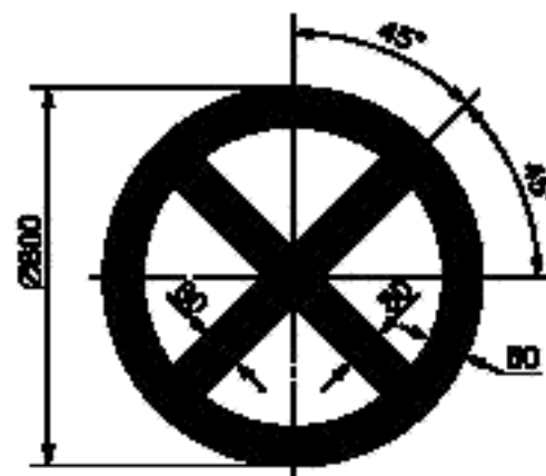
Рисунок 2 — Условное обозначение подруливающего устройства
