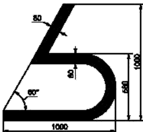
Рисунок 1 — Условное обозначение бульбообразного носа
