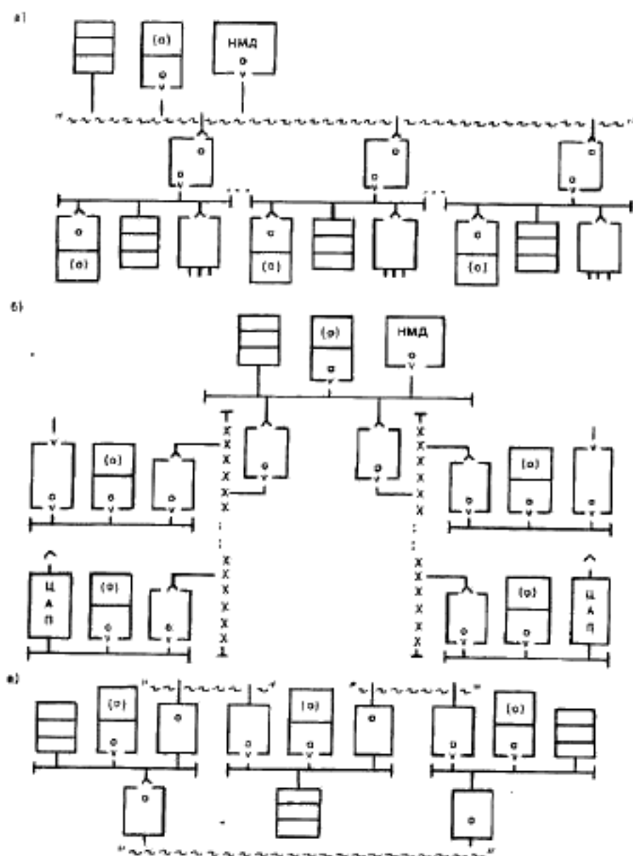
а) звездообразная линейная структура на основе кабельной межконтурной магистральной; б) трехуровневая древовидная структура; в) кольцевая структура
