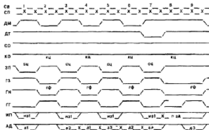
Рисунок Б.6 — Временные диаграммы расщепленных циклов чтения, проводимых одним задатчиком
