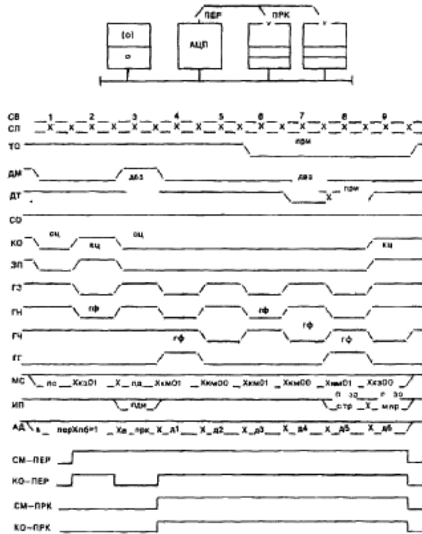
Рисунок Б.7 — Временные диаграммы сигналов в двухадресном групповом цикле передачи с расщеплением памяти, в течение которого также проходит арбитраж ЗО
