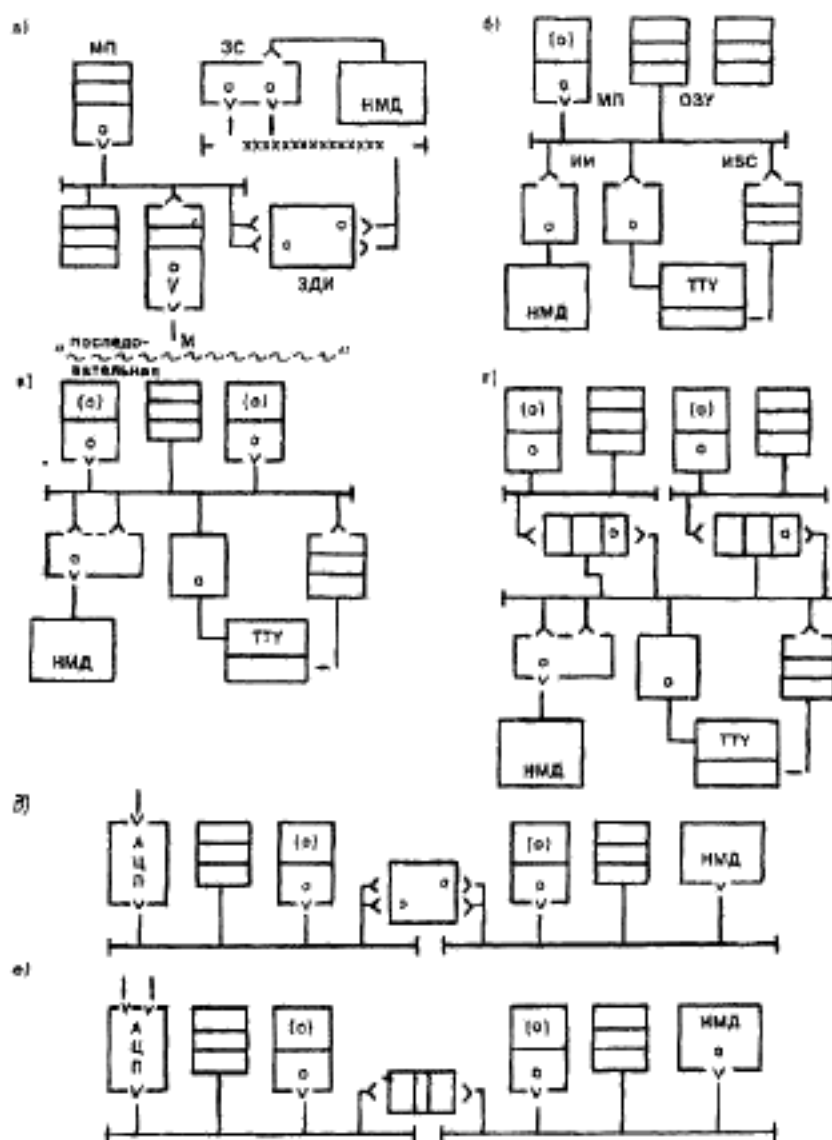
а) одноплатная микроЭВМ, подключенная через кабельную магистраль МСИ к ММД; б) персональная ЭВМ ТТУ; в) двухпроцессорная микроЭВМ; г) вычислительная система с локальными подсистемами обработки данных; д) связь двух микроЭВМ через ЗДИ (прямой доступ к памяти); е) связь двух микроЭВМ через ИС (общее ОЗУ)
