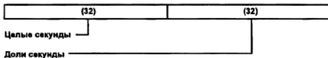
Рисунок 3—10 — Формат данных РУСов ТАЙМ-ЛУТ_РАСЩЕПЛЕНИЯ
