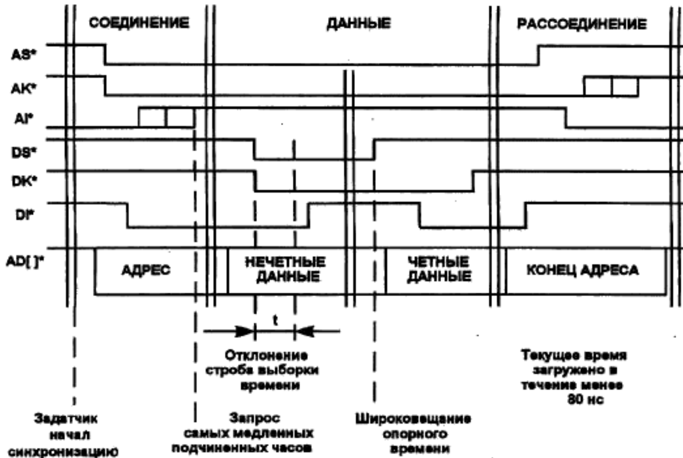
Рисунок 3—4 — Синхронизация часов
