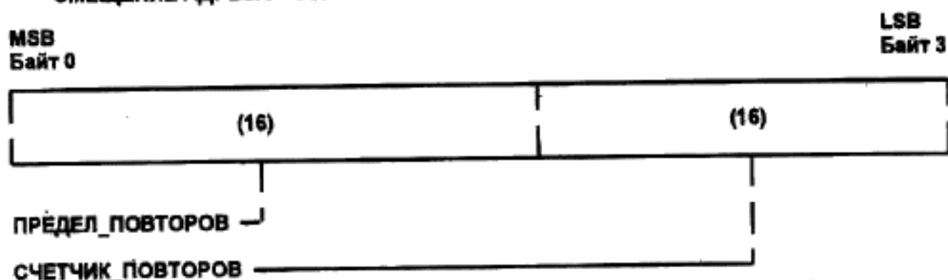
Рисунок 3—26 — Регистр СЧЕТЧИК_ПОВТОРОВ_ПРИ_ОШИБКЕ
