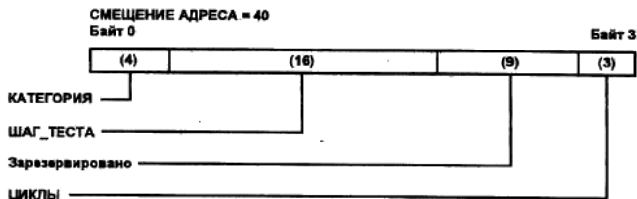
Рисунок 3—12 — Формат данных РУС СТАРТ_ТЕСТА
