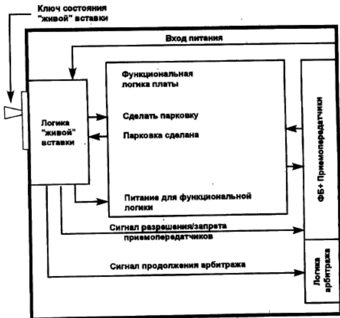
Рисунок 4—2 — Функциональное строение модуля с «живой» вставкой
