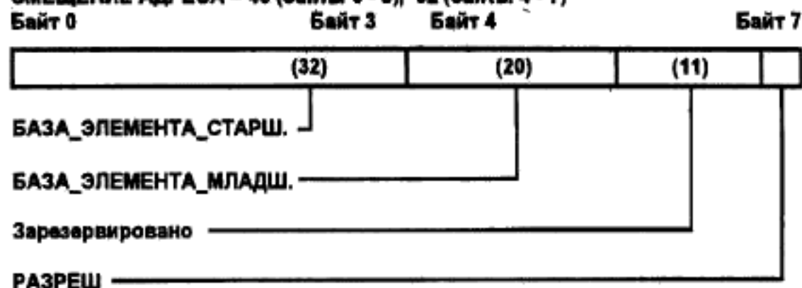
Рисунок 3—14 — Формат данных РУСа БАЗА_ЭЛЕМЕНТОВ
