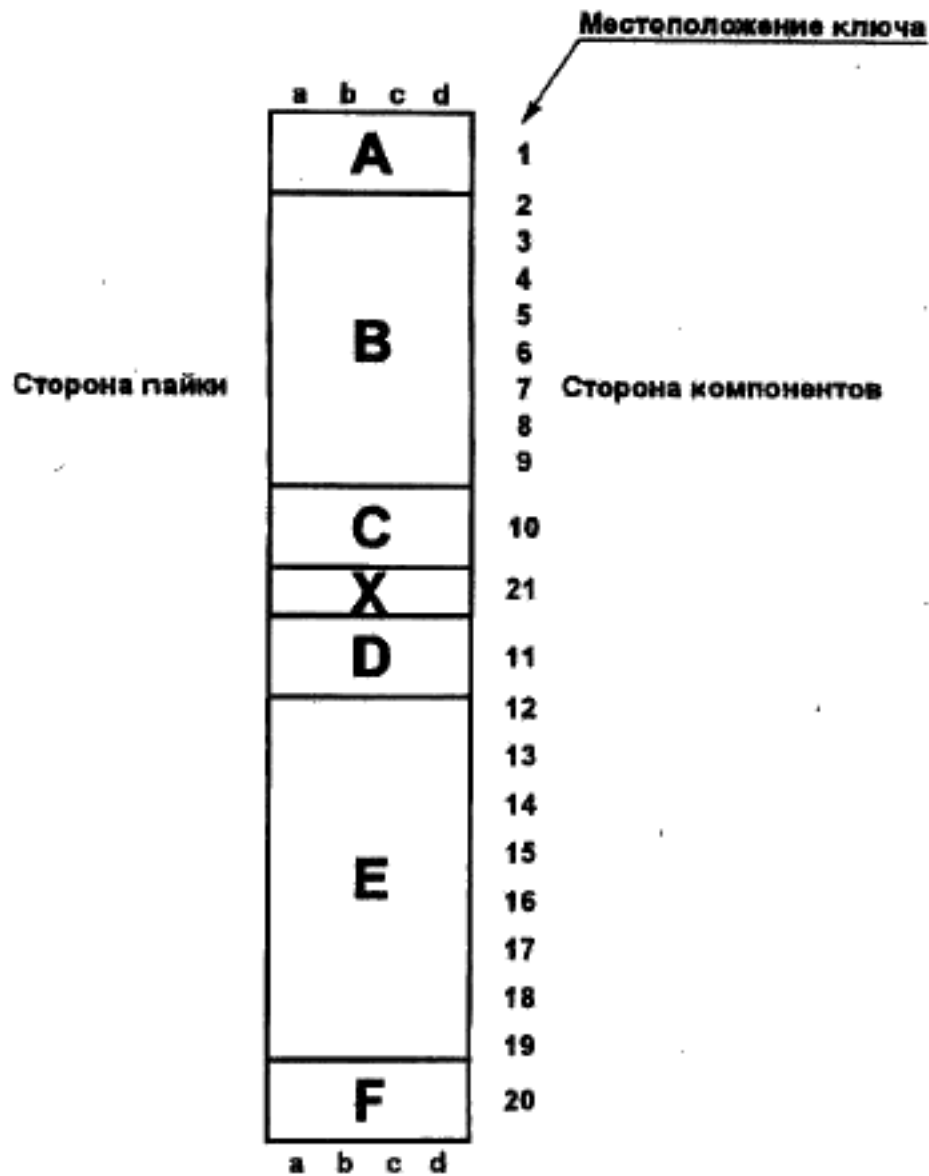
Рисунок 6—13 — Соглашения по наименованию разъемов
