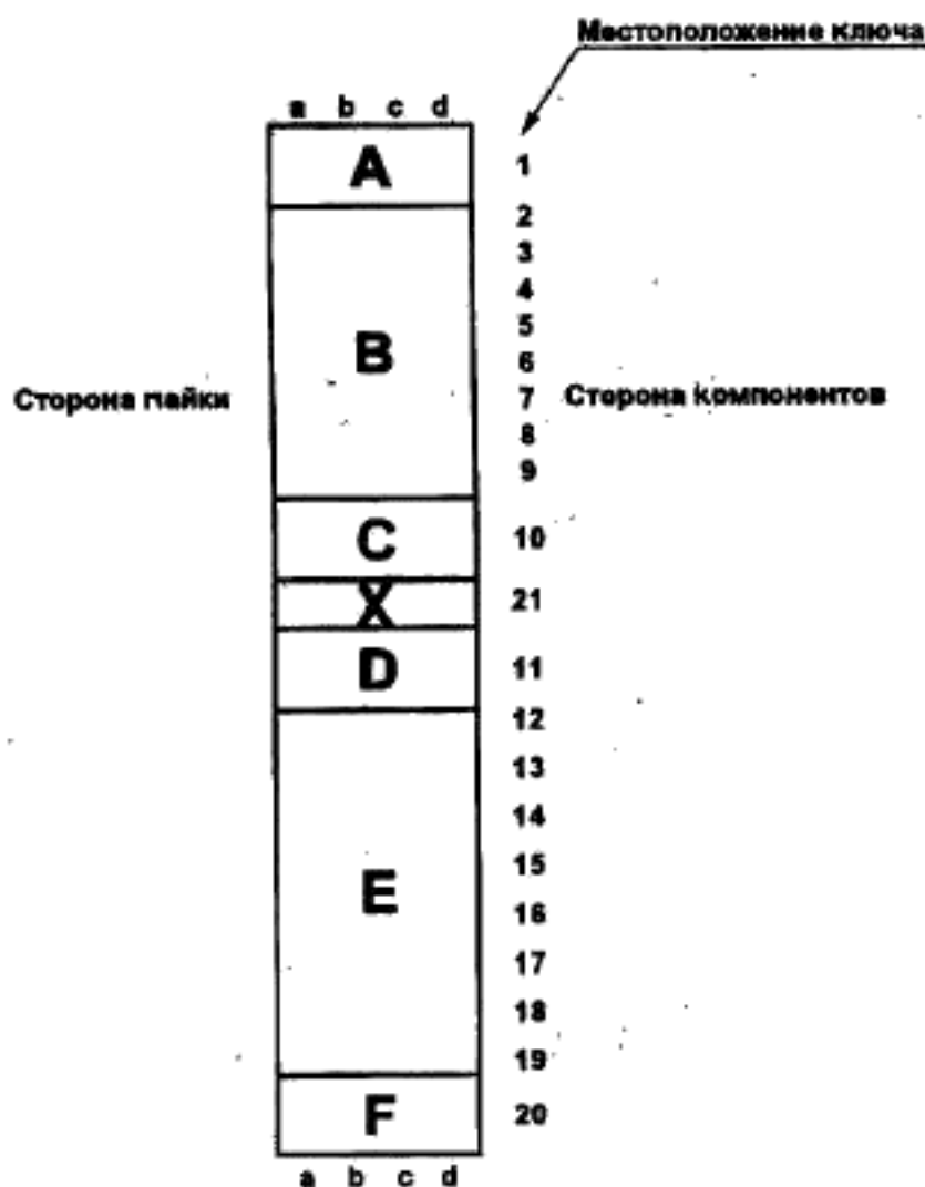
Рисунок 7—13 — Соглашения по наименованию разъемов
