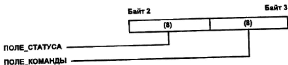
Рисунок 3—19(б) — Формат данных РУСа ОШИБКА_СТАРИШ (младшая половина)
