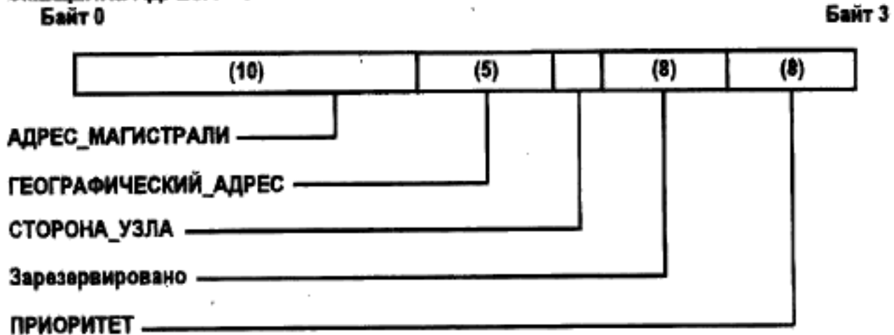
Рисунок 3—6 — Формат данных РУСа ИДЕНТИФИКАТОРЫ_УЗЛА
