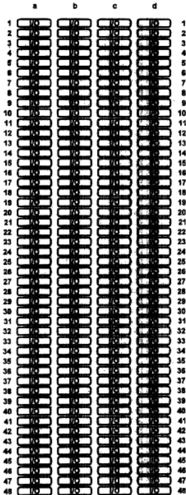
Рисунок 6—16 — Распределение контактов разъема E для 192 ввода/вывода
