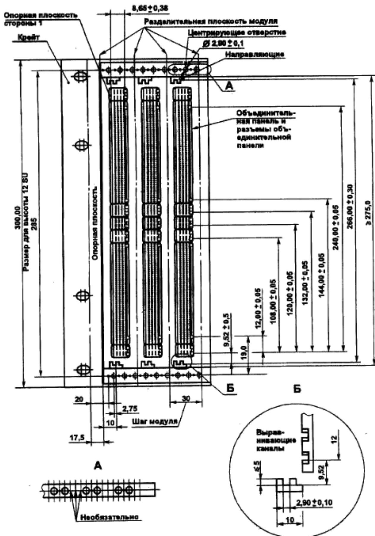
Рисунок 7-3 — X-Y вид соединения крейта и модуля
