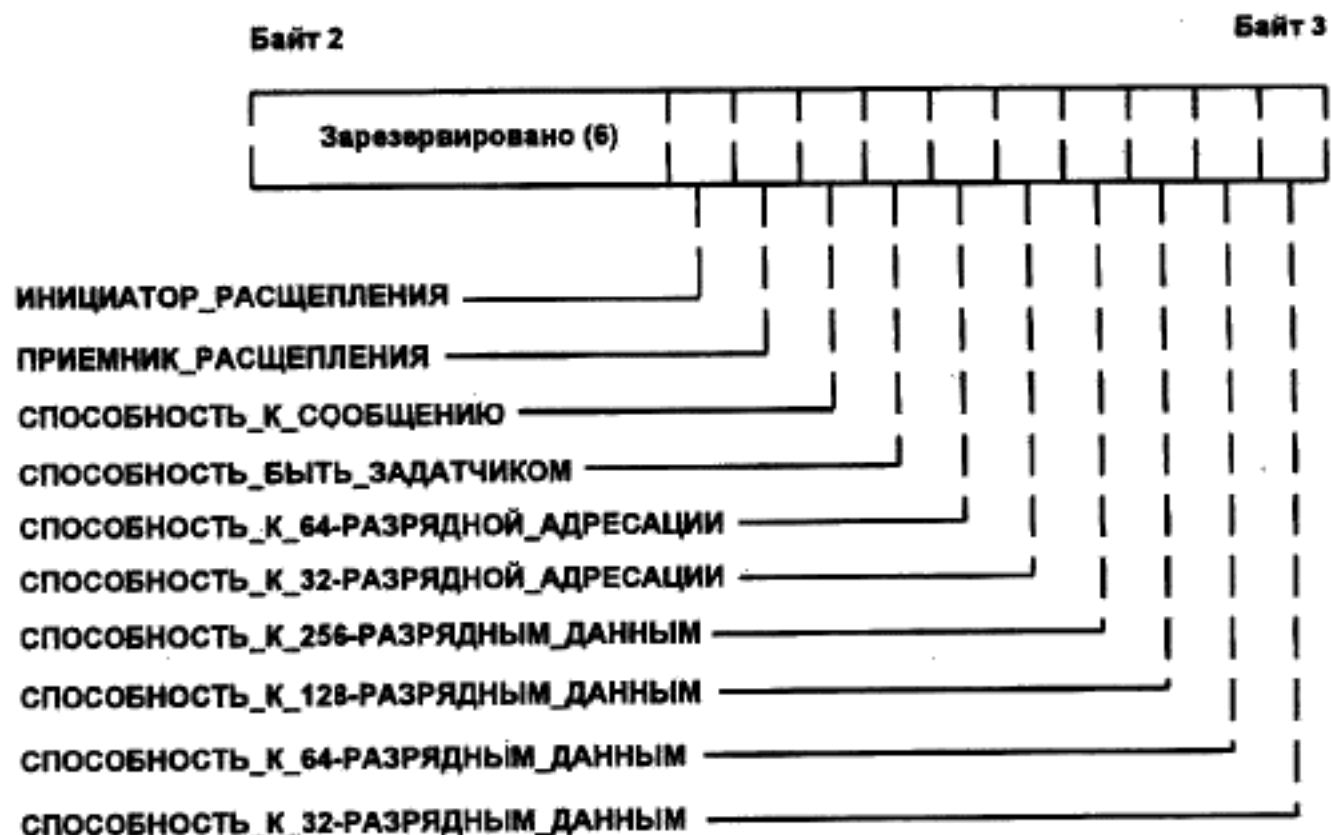
Рисунок 3—28(6) — ЛОГИЧЕСКАЯ СПОСОБНОСТЬ МОДУЛЯ (Младшая половина)
