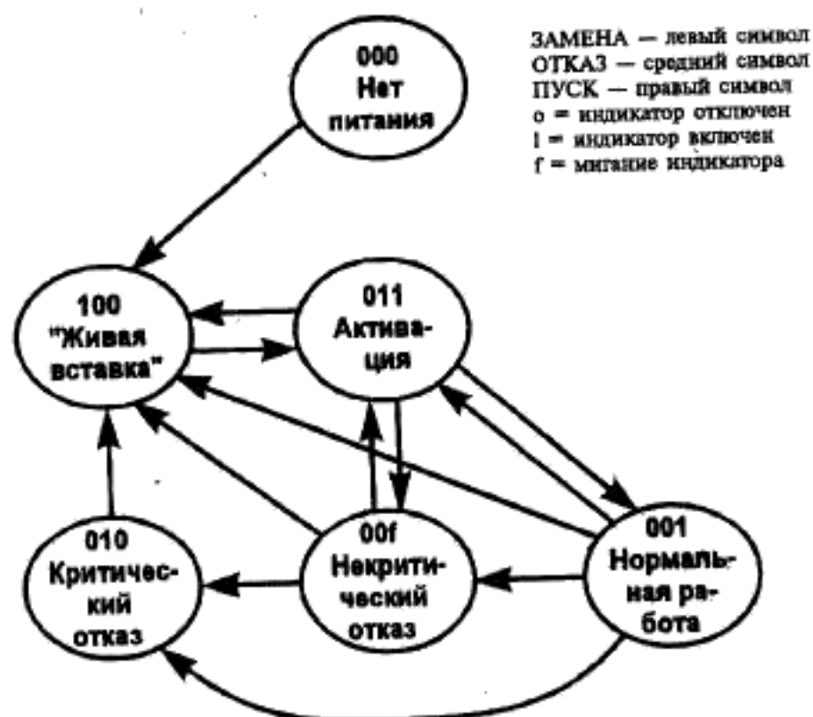
Рисунок 4—1 — Диаграмма состояний «живой» вставки модуля
