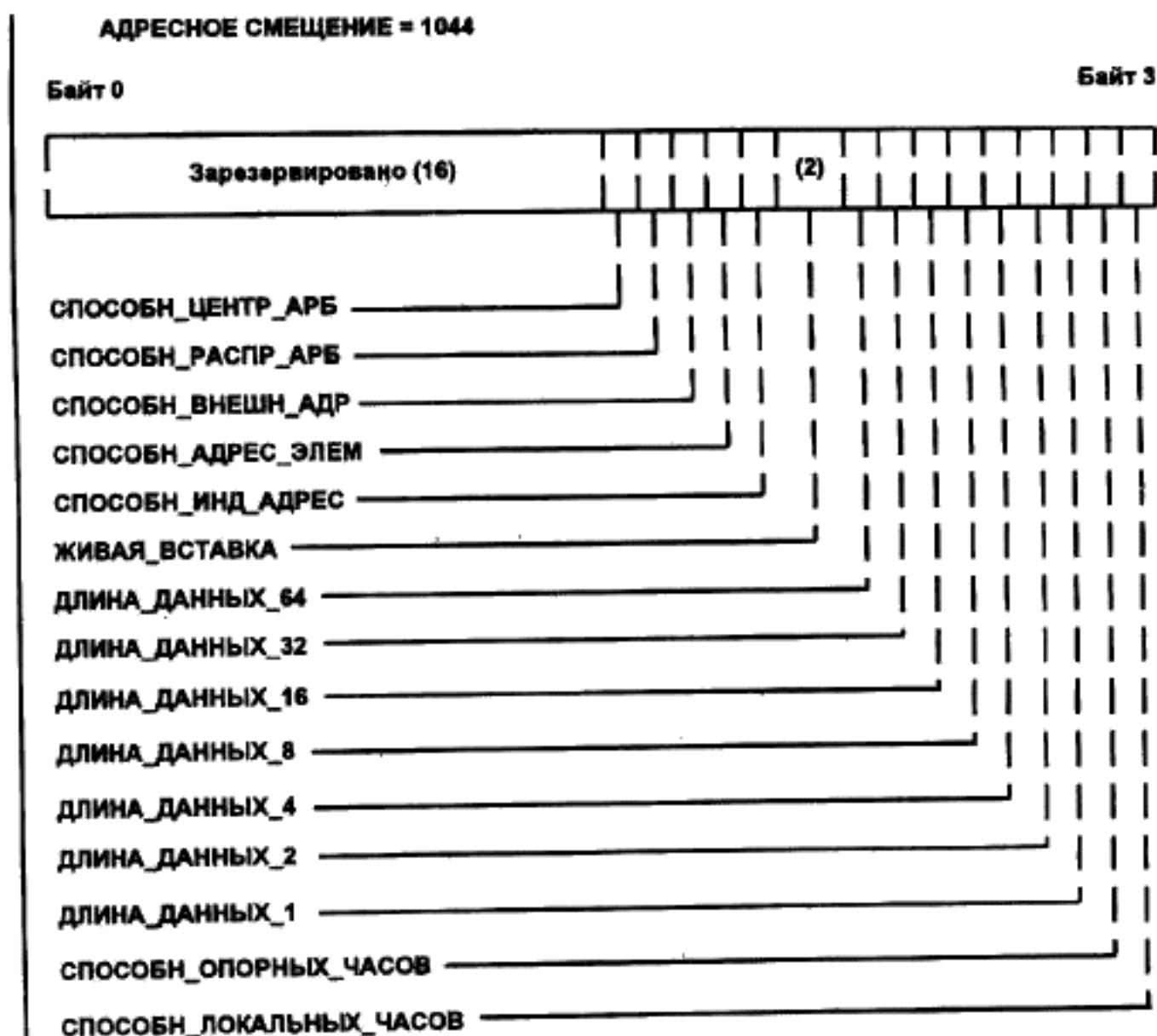
Рисунок 3—29 — Формат РУС ВНЕШНИЕ_СПОСОБНОСТИ_УЗЛА
