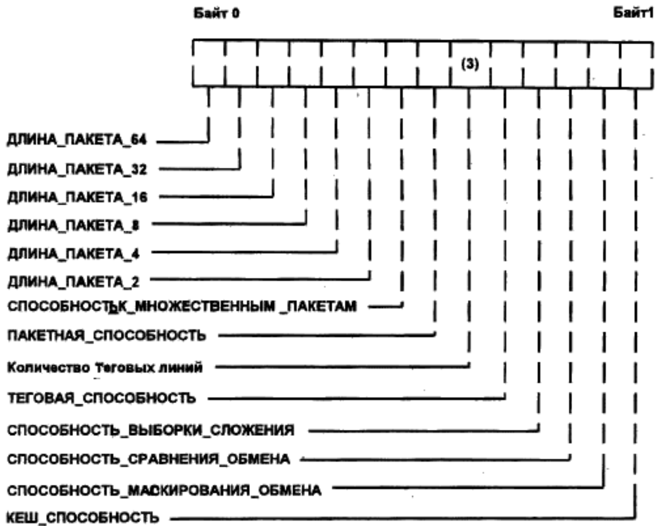
Рисунок 3—28(а) — ЛОГИЧЕСКАЯ_СПОСОБНОСТЬ_МОДУЛЯ (Старшая половина)
