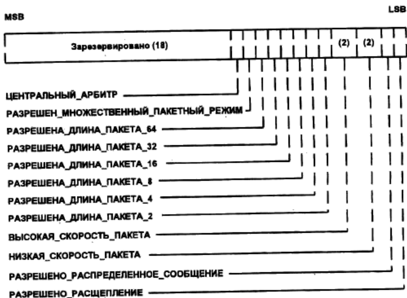
Рисунок 3—22 — Формат регистра ОБЩЕГО ЛОГИЧЕСКОГО УПРАВЛЕНИЯ
