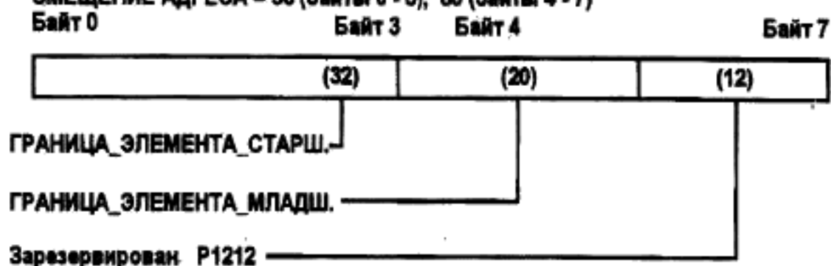
Рисунок 3—15 — Формат данных РУСа ГРАНИЦА_ЭЛЕМЕНТОВ
