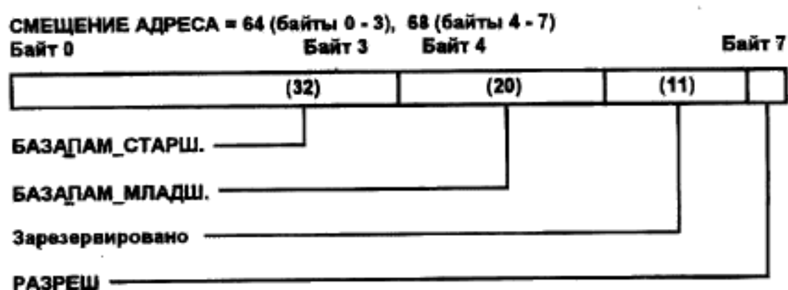
Рисунок 3—16 — Формат данных РУС БАЗА_ПАМЯТИ
