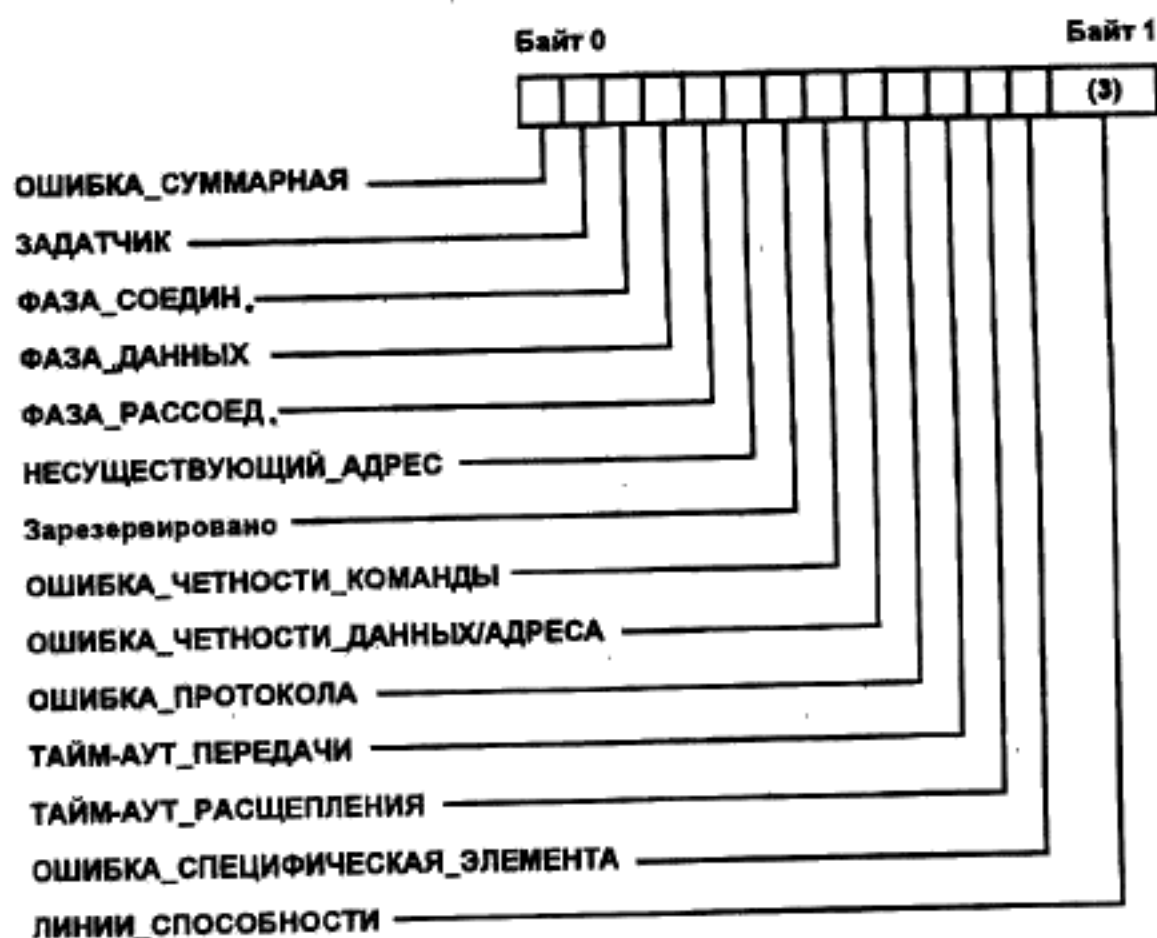
Рисунок 3—19(а) — Формат данных РУСа ОШИБКА_СТАРИШ (старшая половина)
