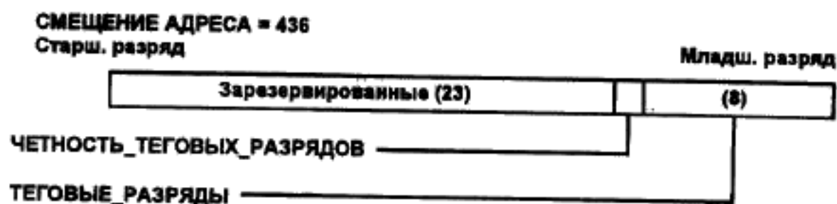
Рисунок 3—21 — Формат данных РУСа УДЕРЖАНИЕ_ТЕГОВ
