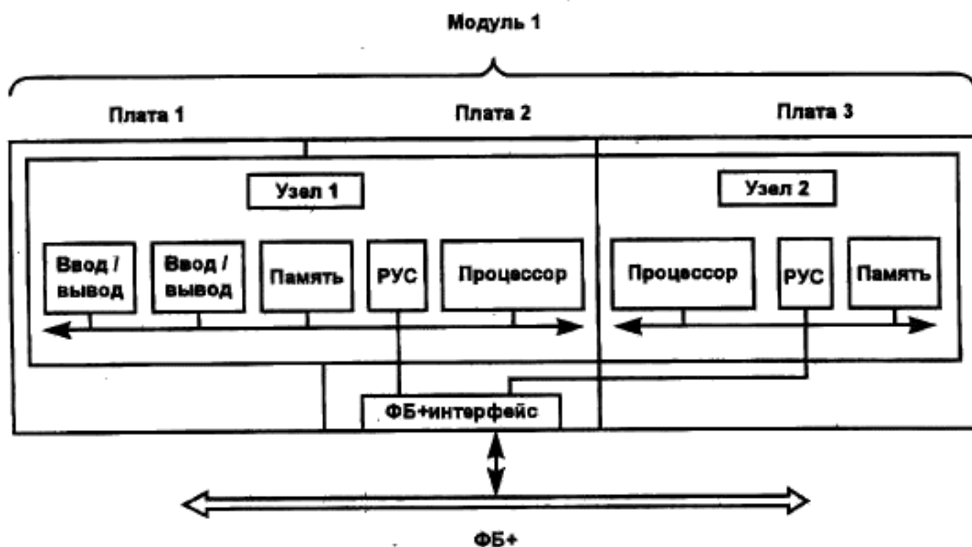
Рисунок 3—1 — ФБ+ платы, модули, узлы
