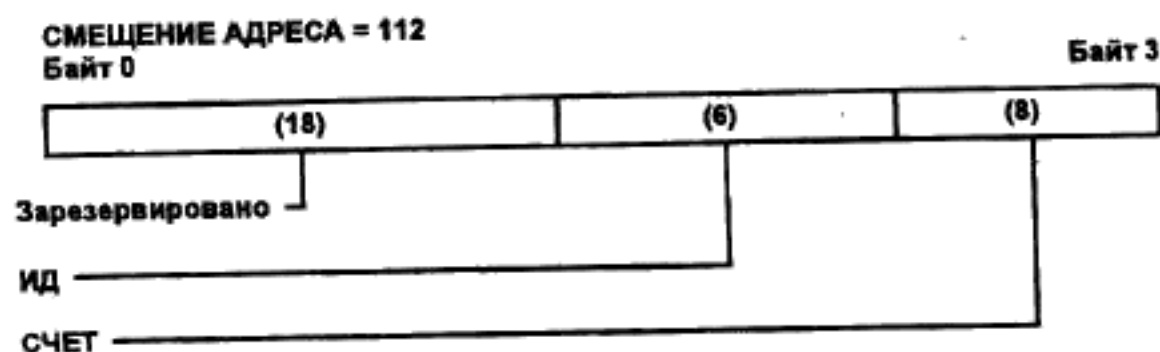
Рисунок 3—18 — Формат данных РУСа СТРОБ_ЧАСОВ
