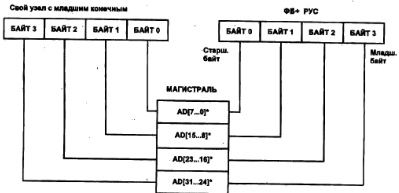
Рисунок 3—3(б) — Расположение байтов РУСа
