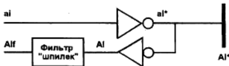
Рисунок 2.1 — Соглашения о сигналах
