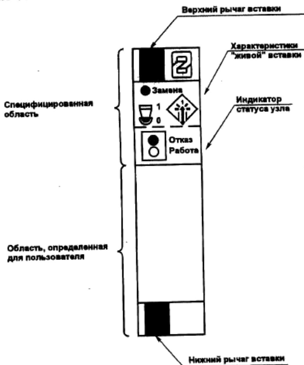
Рисунок 6—9 — Организация передней панели профиля А
