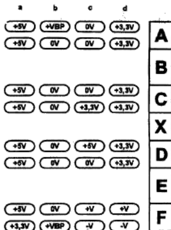
Рисунок 6—18 — Распределение контактов питания для разъемов профиля А
