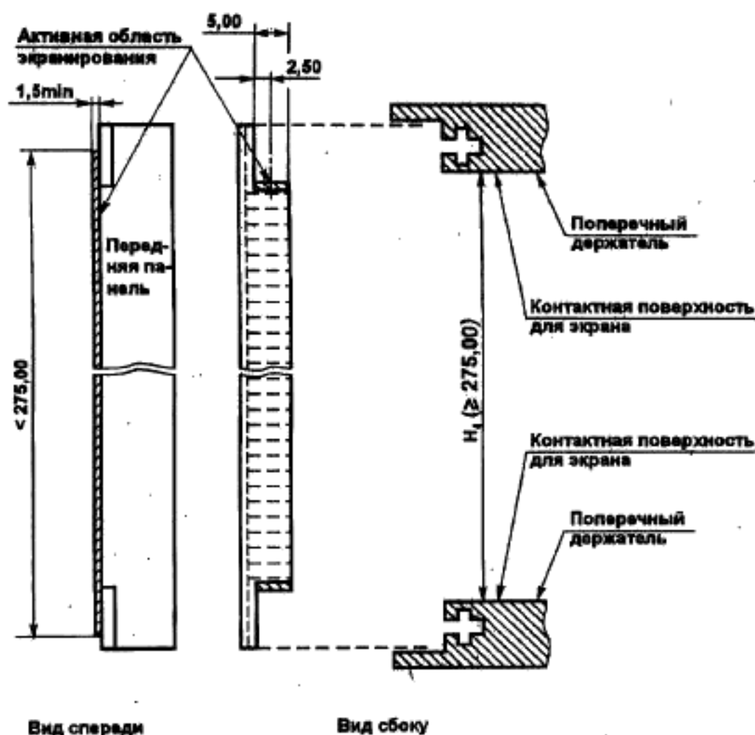
Рисунок 7—12 — Расположение EMI/RFI экранов и соединения поверхностей (альтернатива)
