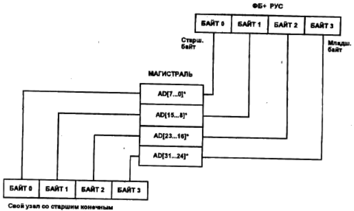
Рисунок 3—3(а) — Расположение байтов РУСа
