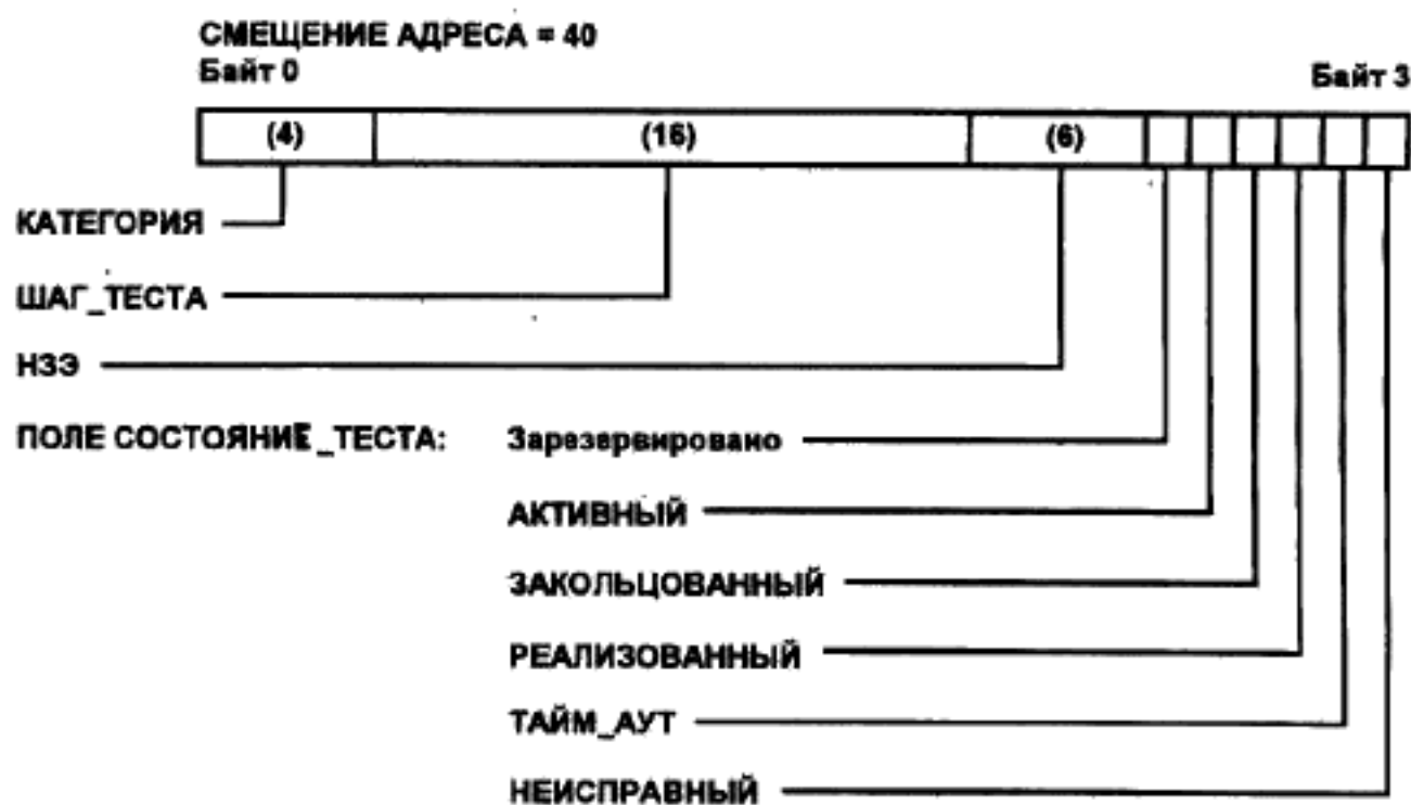
Рисунок 3—13 — Формат данных РУСа СТАТУС_ТЕСТА
