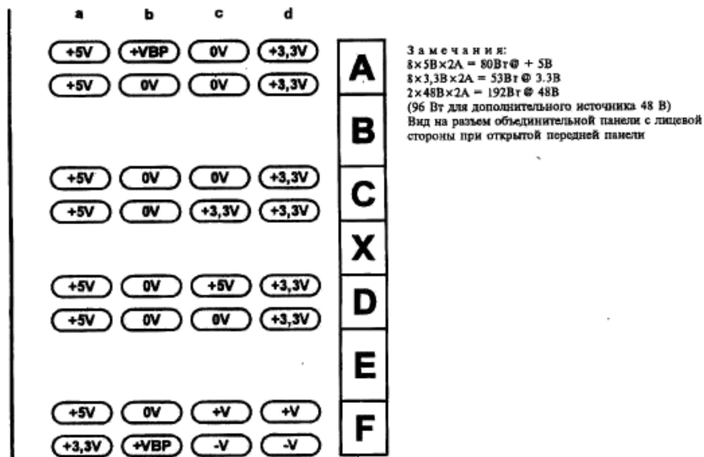
Рисунок 7—16 — Распределение контактов питания для разъемов профиля Б
