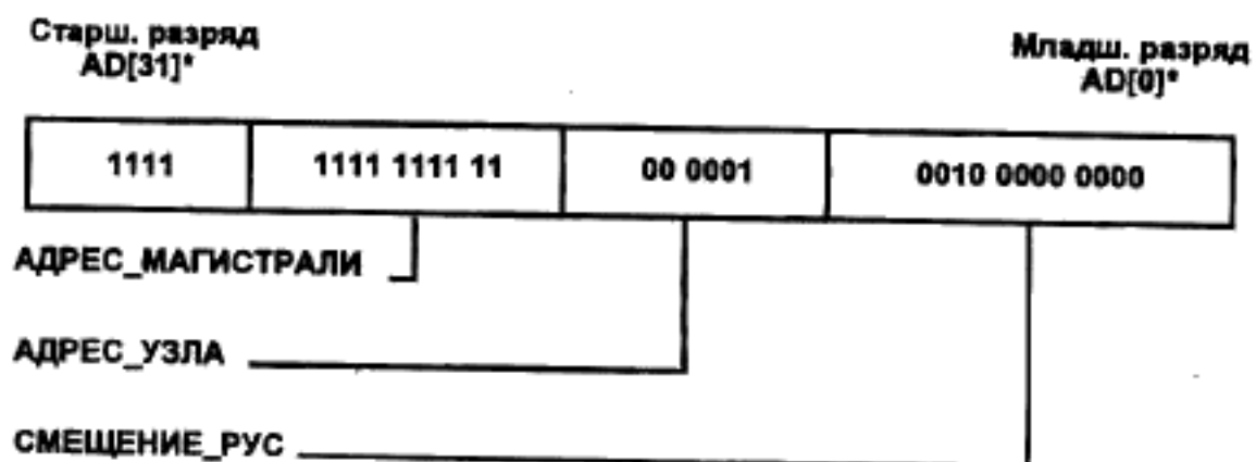
Рисунок 3-2(в) — Адресация 32-разрядных РУС
