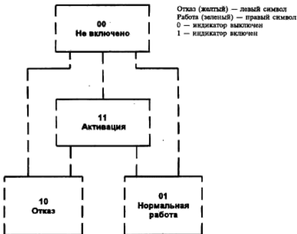
Рисунок 6—10 — Диаграмма состояний модуля
