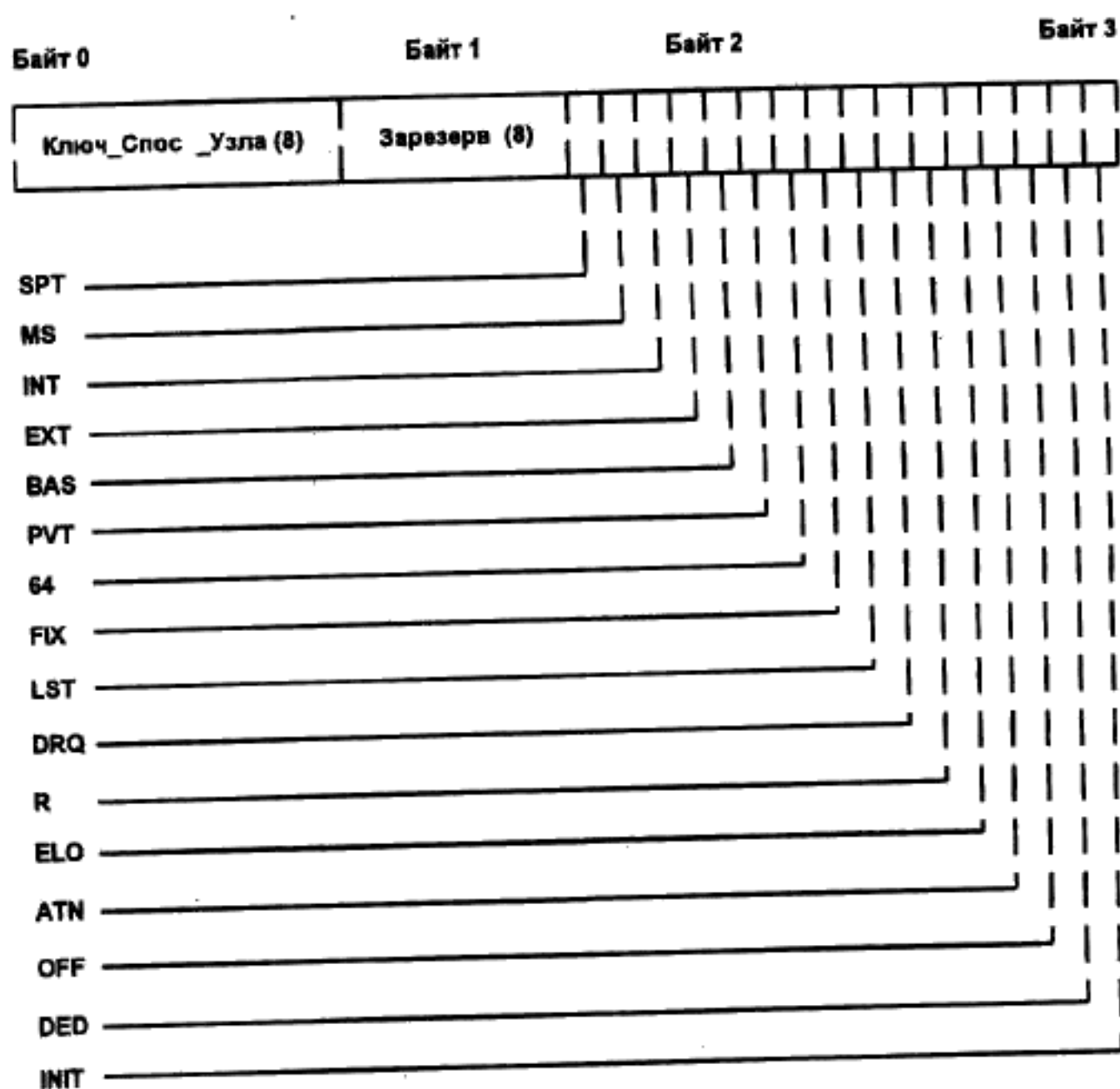
Рисунок 3—33 — Формат Входа СПОСОБНОСТИ_УЗЛА
