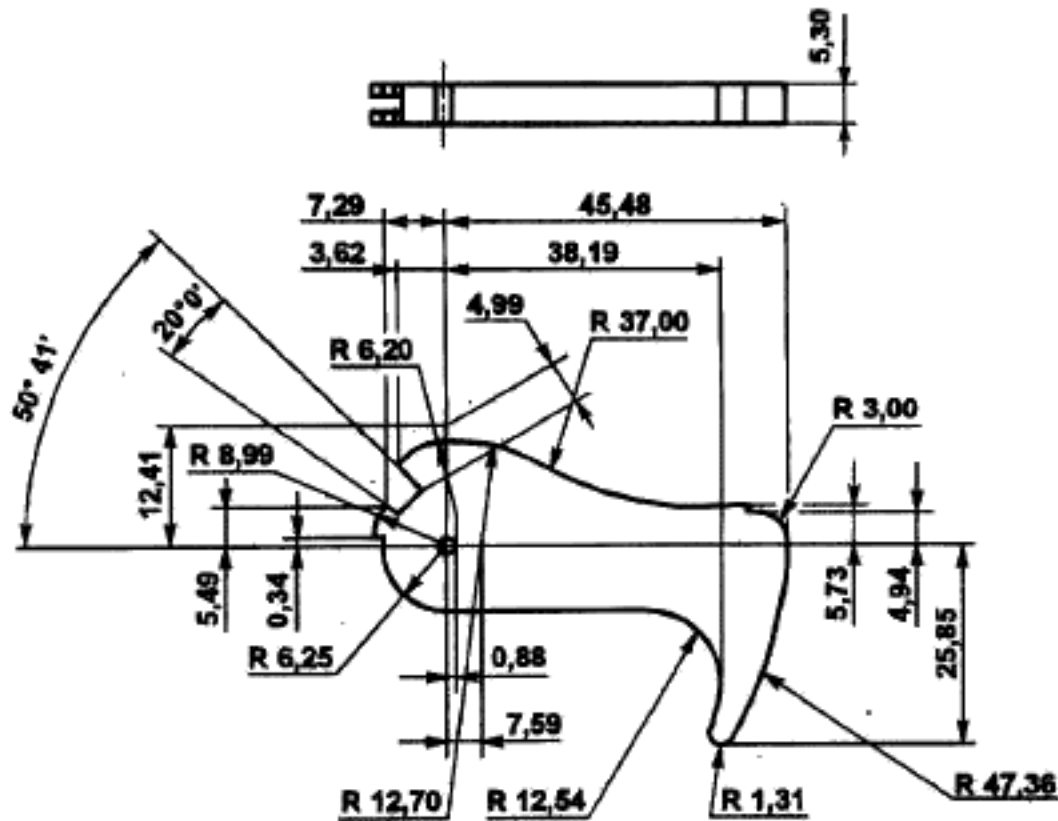
Рисунок 7—7 — рекомендуемый для Профиля Б рычаг вставки/вынимания
