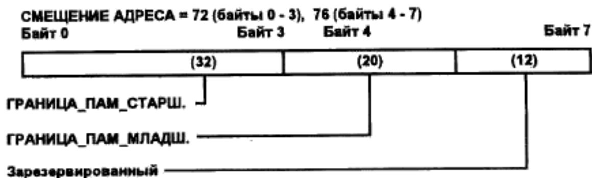
Рисунок 3—17 — Формат данных РУСа ГРАНИЦА_ПАМЯТИ
