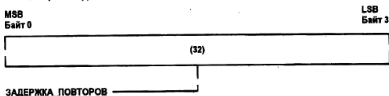
Рисунок 3—27 — Регистр ЗАДЕРЖКА_ПОВТОРОВ_ПРИ_ОШИБКЕ
