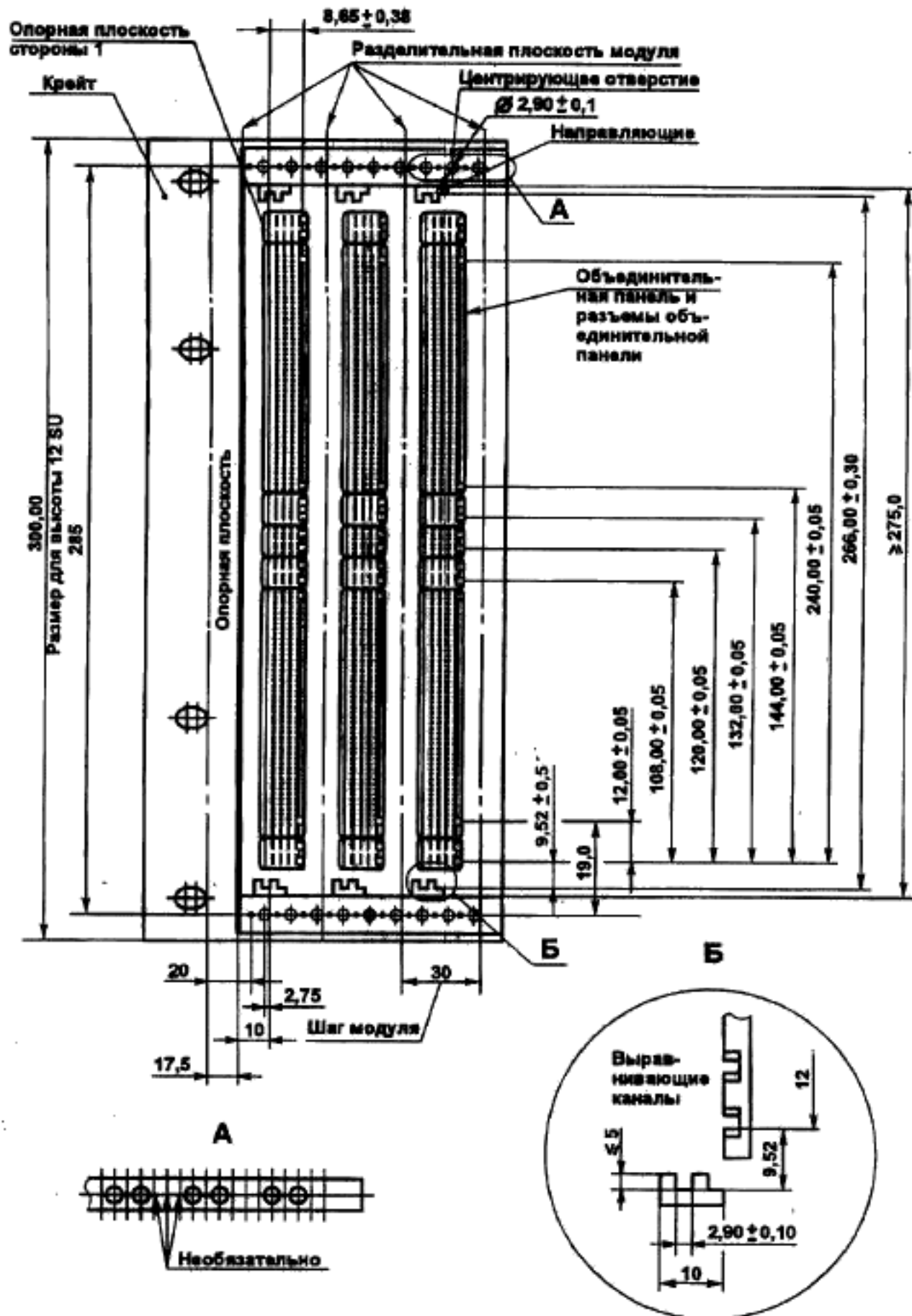
Рисунок 6—2 — Вид соединения Крейт/Объединительная плата
