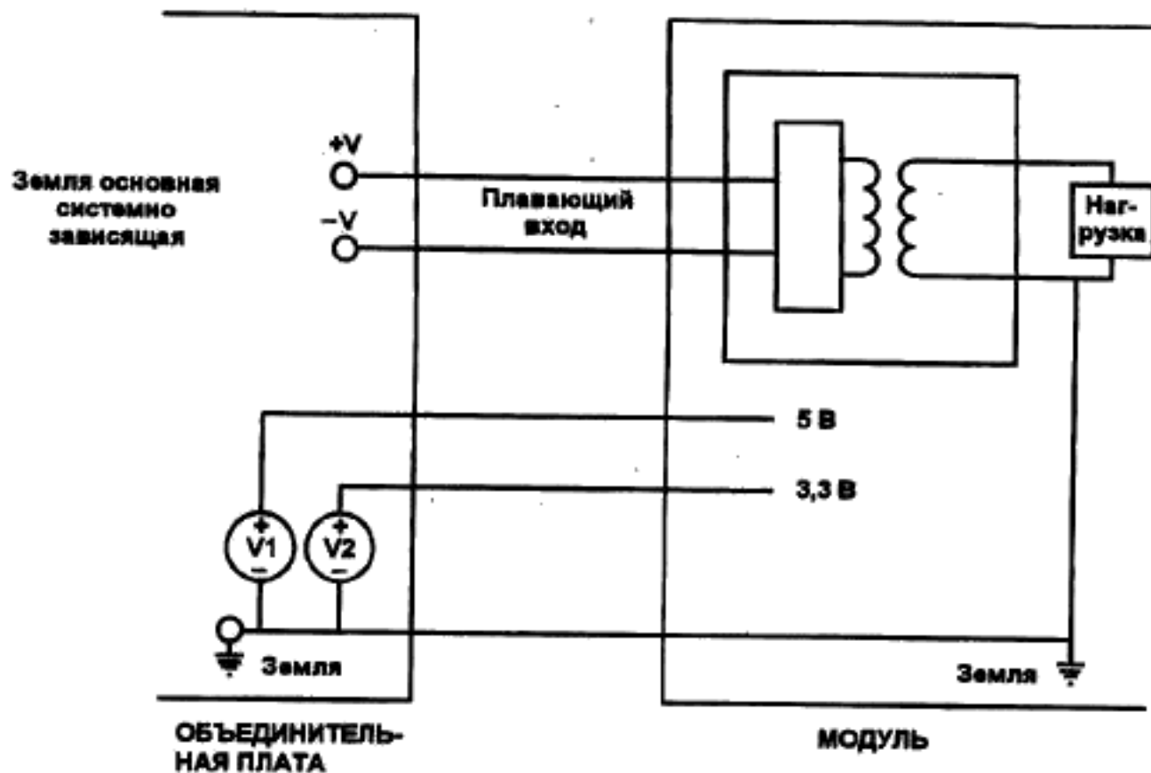
Рисунок 6—1 — Шины питания профиля А
