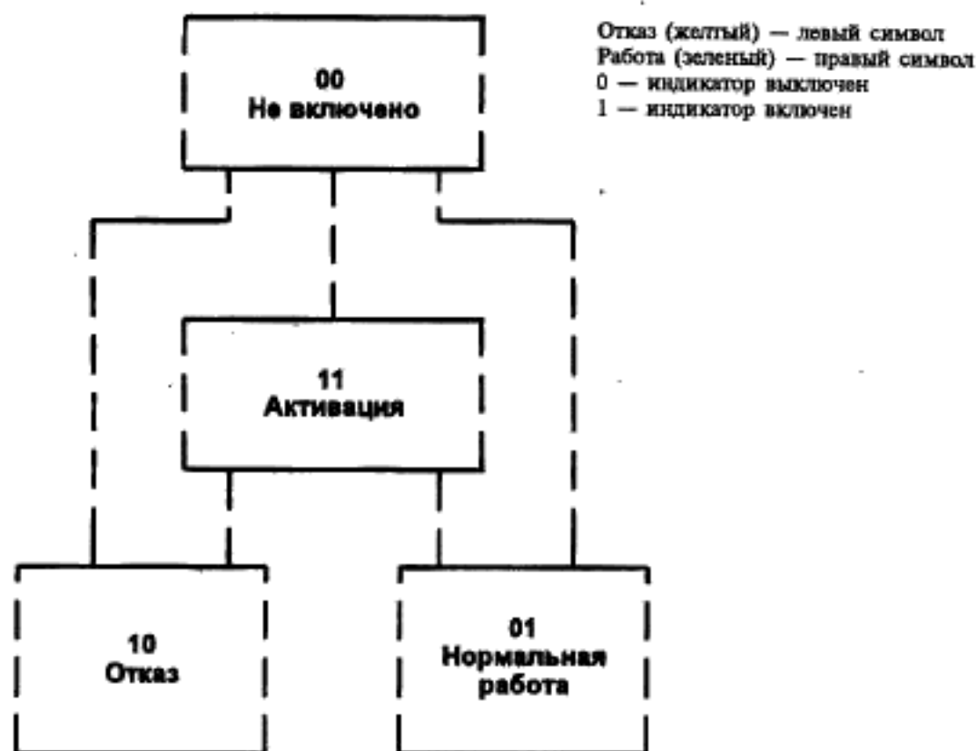
Рисунок 7—10 — Диаграмма состояний модуля
