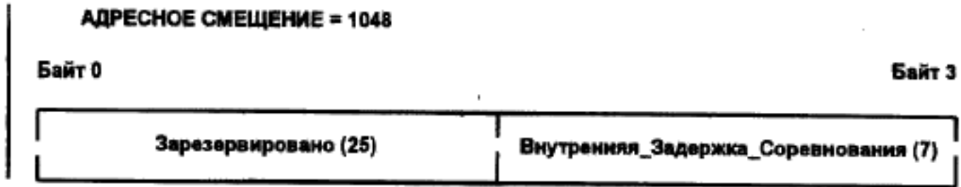
Рисунок 3—30 — Формат РУС ВНУТРЕННЯЯ_ЗАДЕРЖКА_СОРЕВНОВАНИЯ
