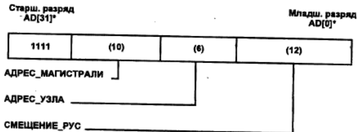
Рисунок 3-2(б) — Адресация 32-разрядных РУС
