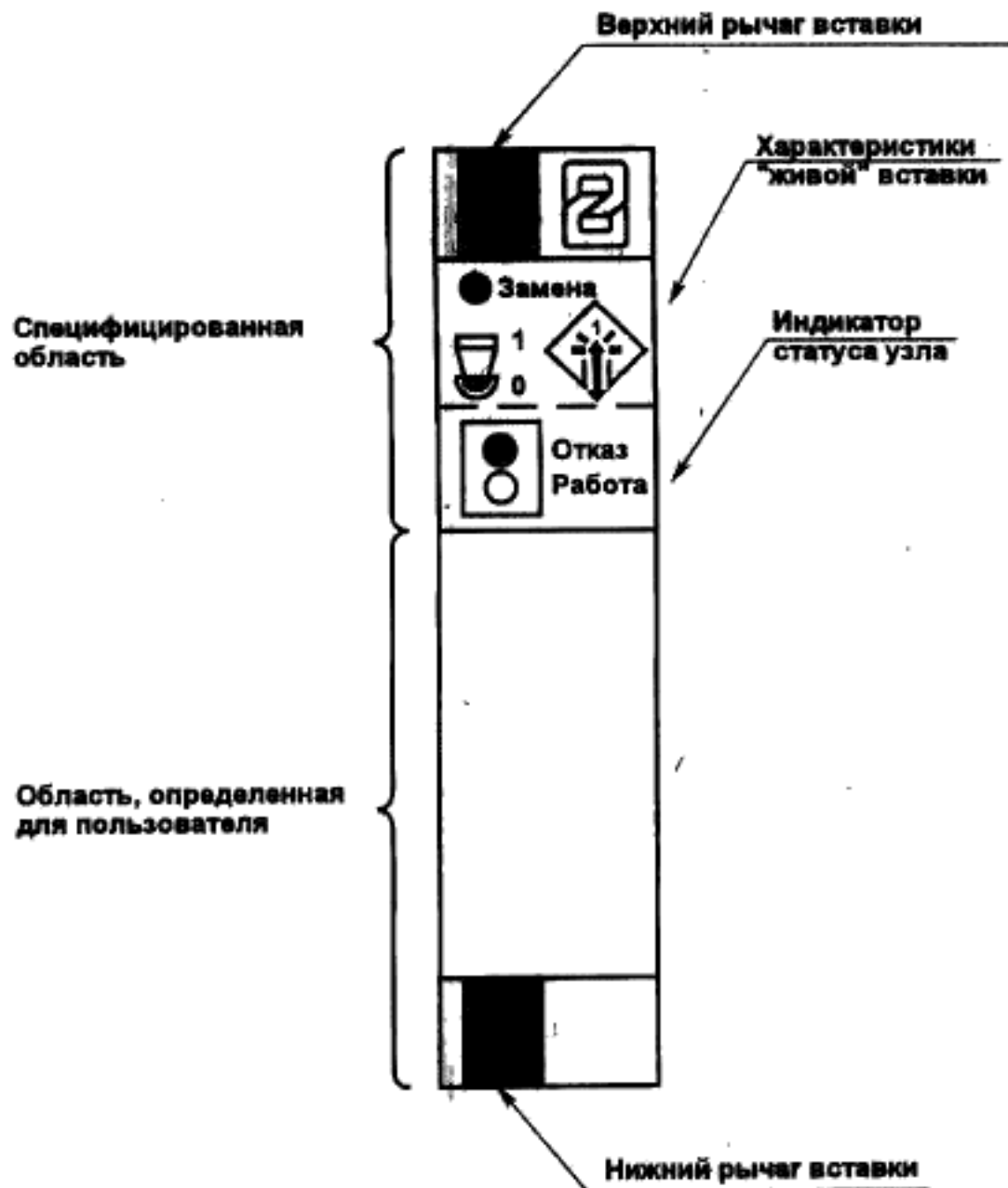
Рисунок 7—9 — Организация передней панели профиля Б
