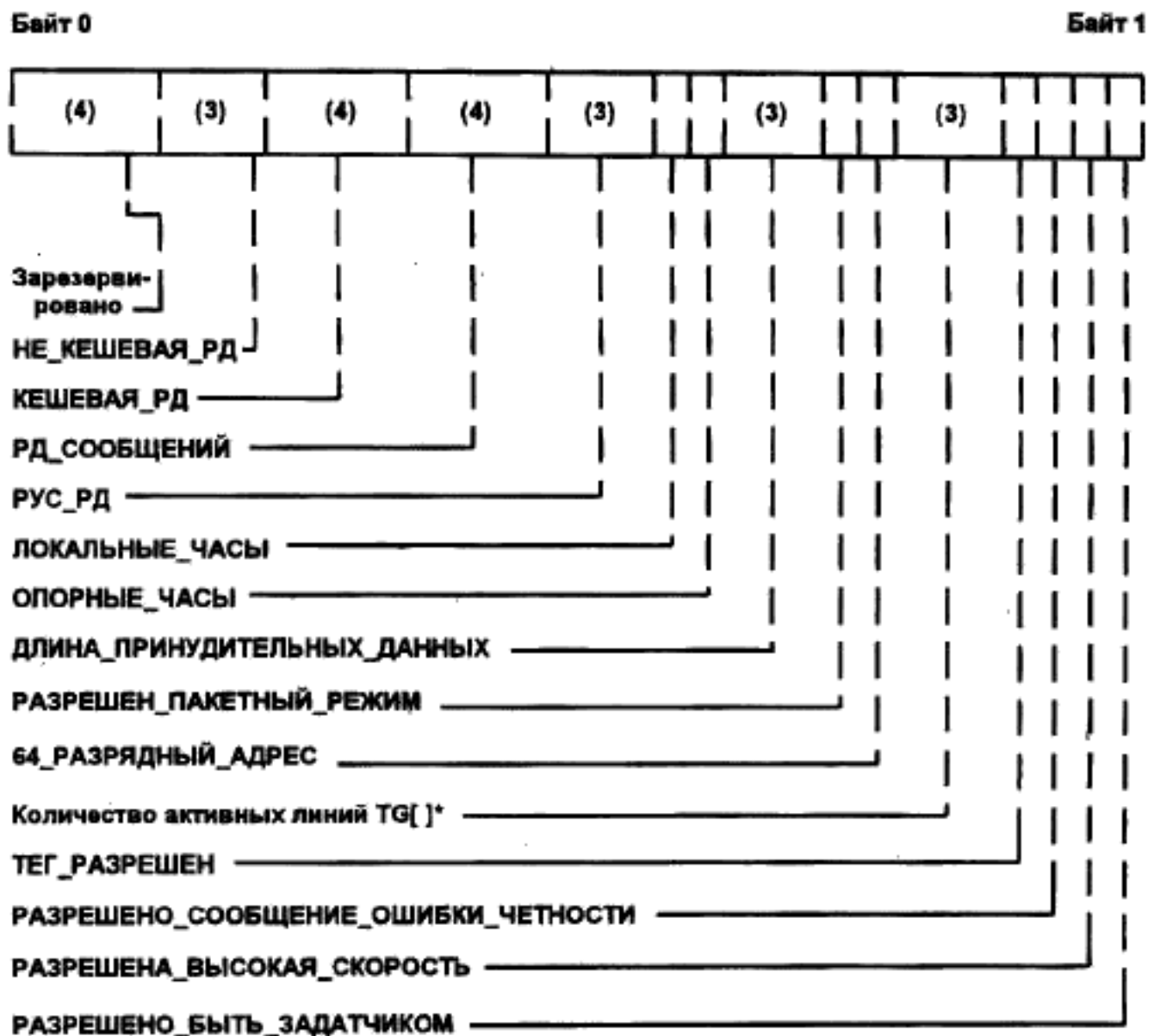
Рисунок 3—23 — Формат регистра ЛОГИЧЕСКОГО_УПРАВЛЕНИЯ_МОДУЛЯ
