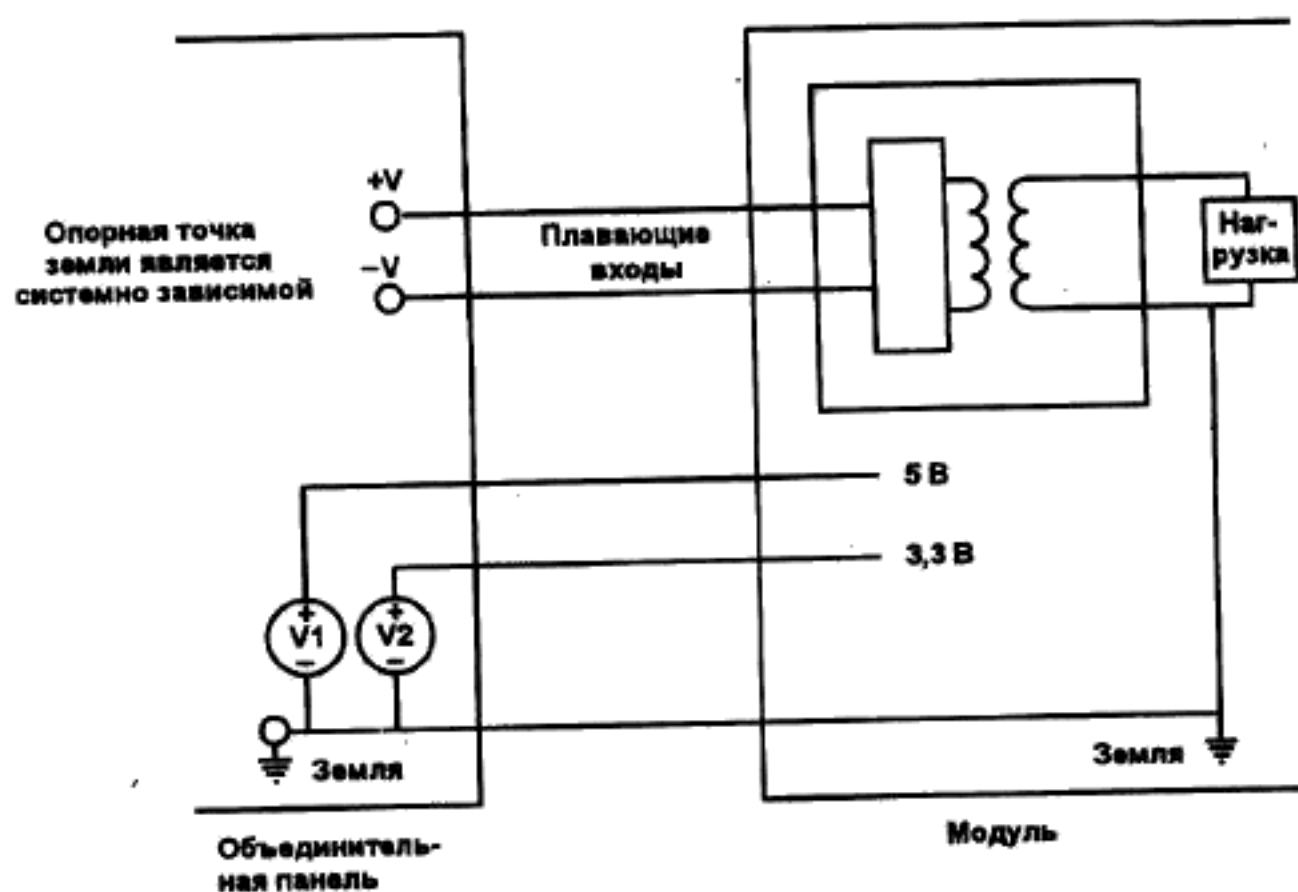
Рисунок 7-1 — Шины питания Профиля Б
