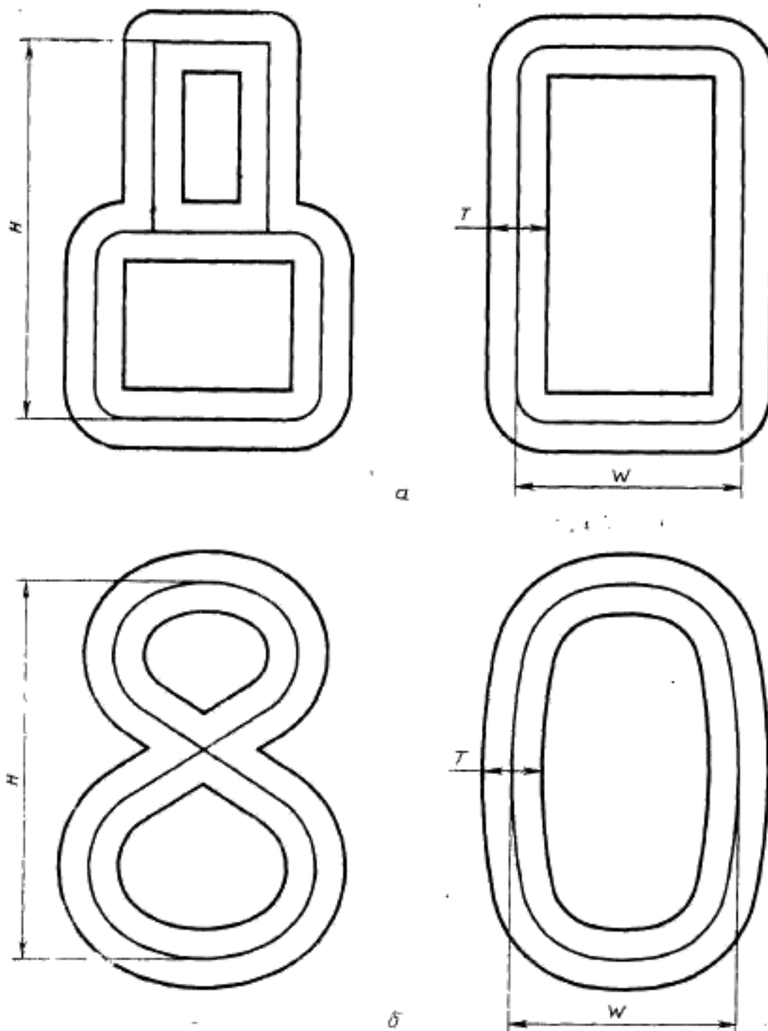
а—шрифт РОС-А; б—шрифт РОС-Б Черт. 1
