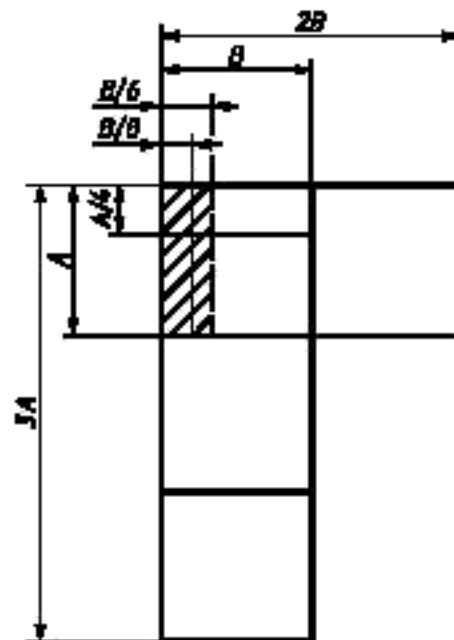
Размеры посадочных окон для панелей, устройств нестойкого типа, блочных каркасов и блоков различного назначения
