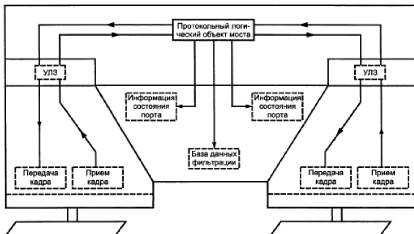
Рисунок 3.6 — Операции межмостового протокола
