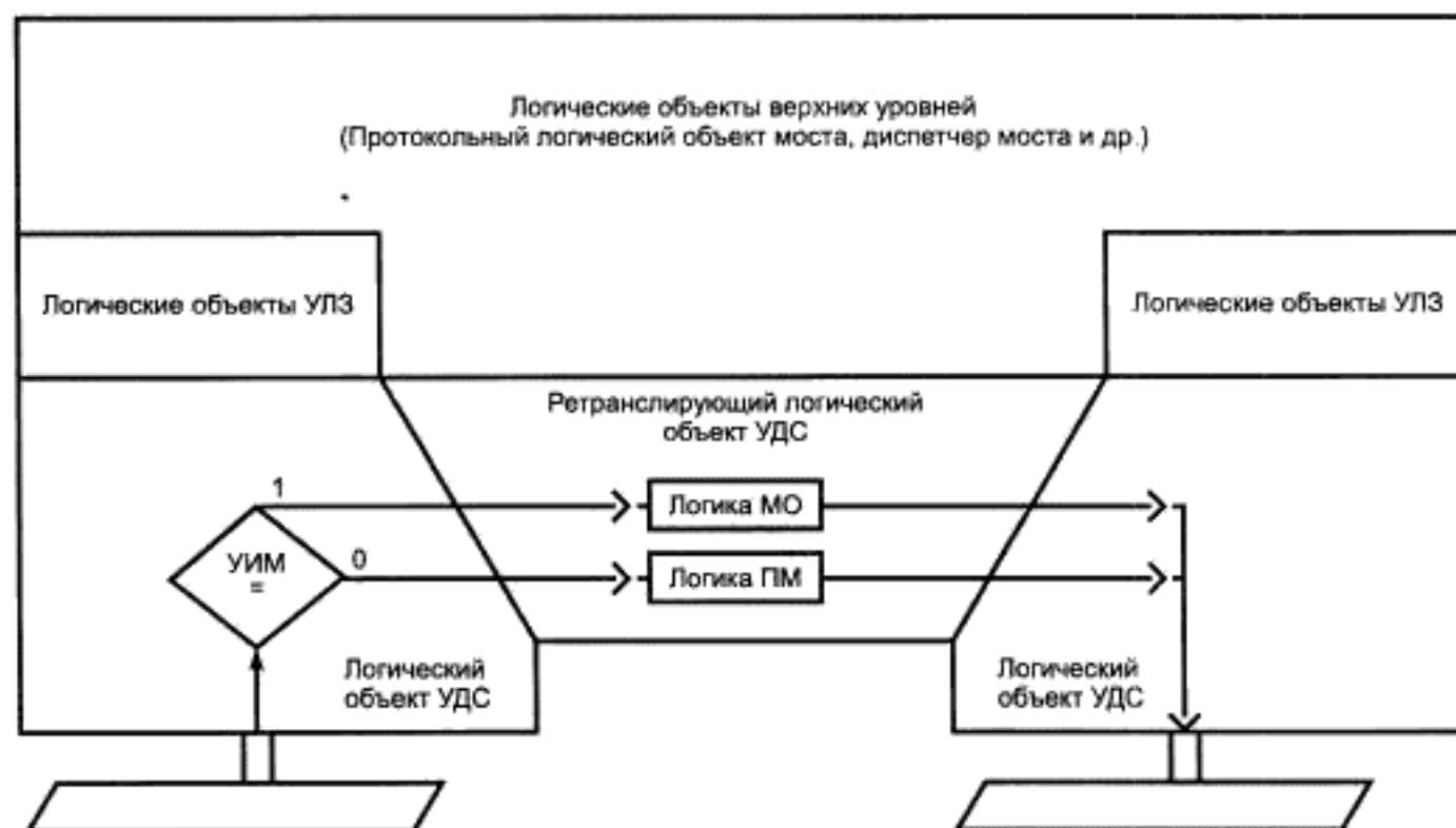
Рисунок С.1 — Логика операций моста ПМСО
