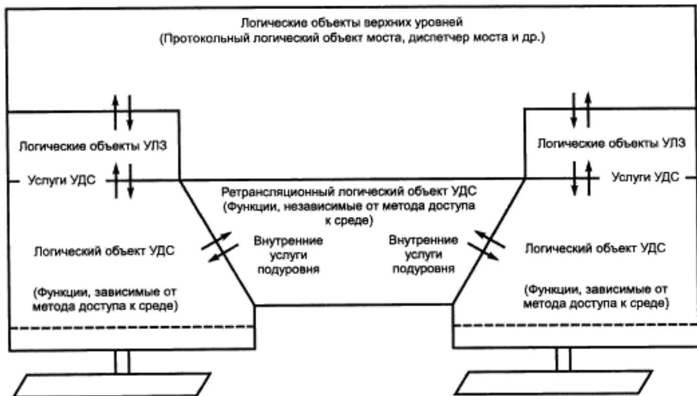
Рисунок 3.3 — Архитектура моста
