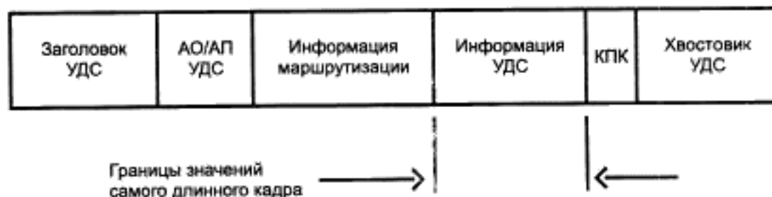
Рисунок С.6 — Границы значений самого длинного кадра
