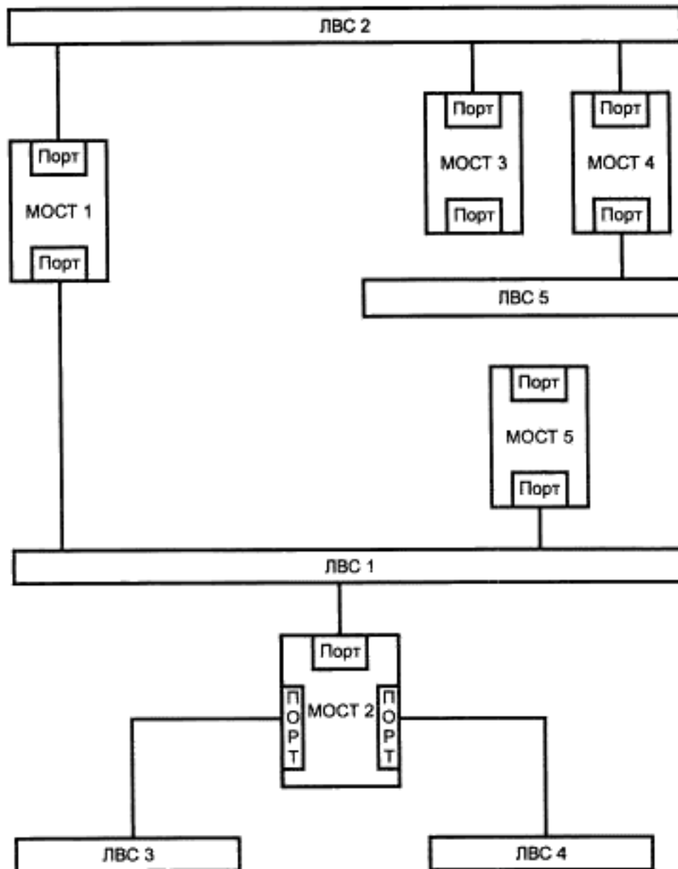
Рисунок 4.1 — Активная топология
