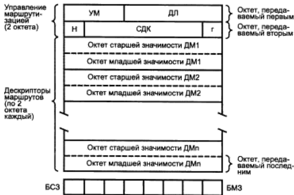
Рисунок С.3 — Поле информации маршрутизации
