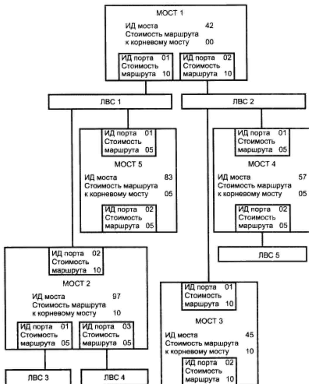
Рисунок 4.2 — Связующее дерево
