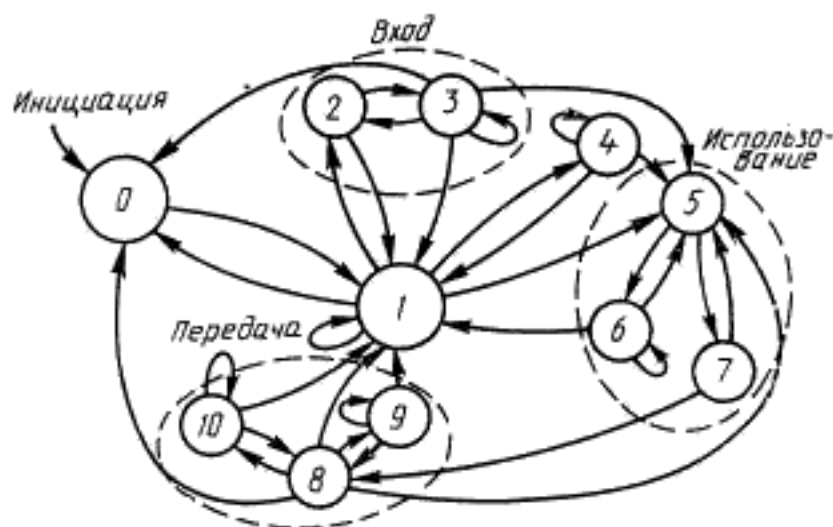
Диаграмма состояний конечного автомата управления доступом
