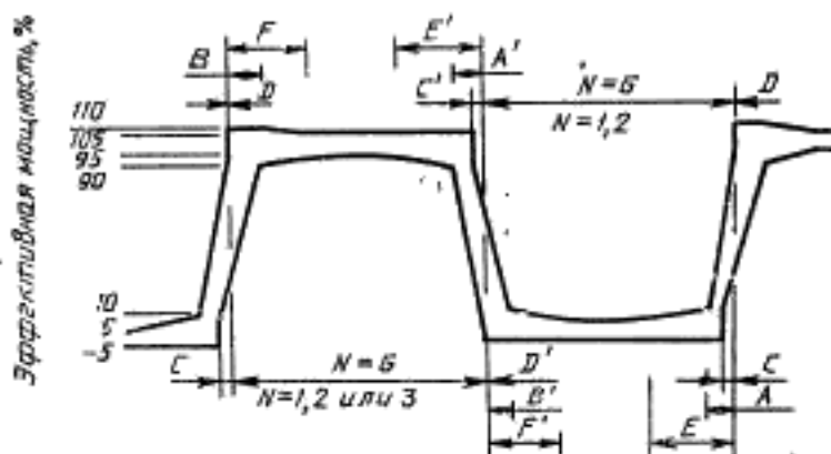
Форма оптического волнового сигнала
