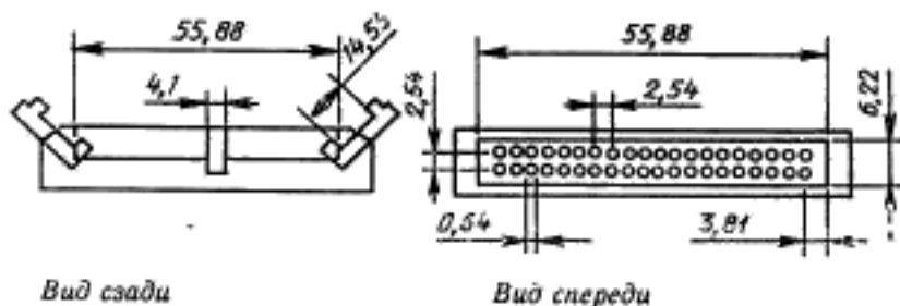
Розетка одинарного интерфейсного соединителя
