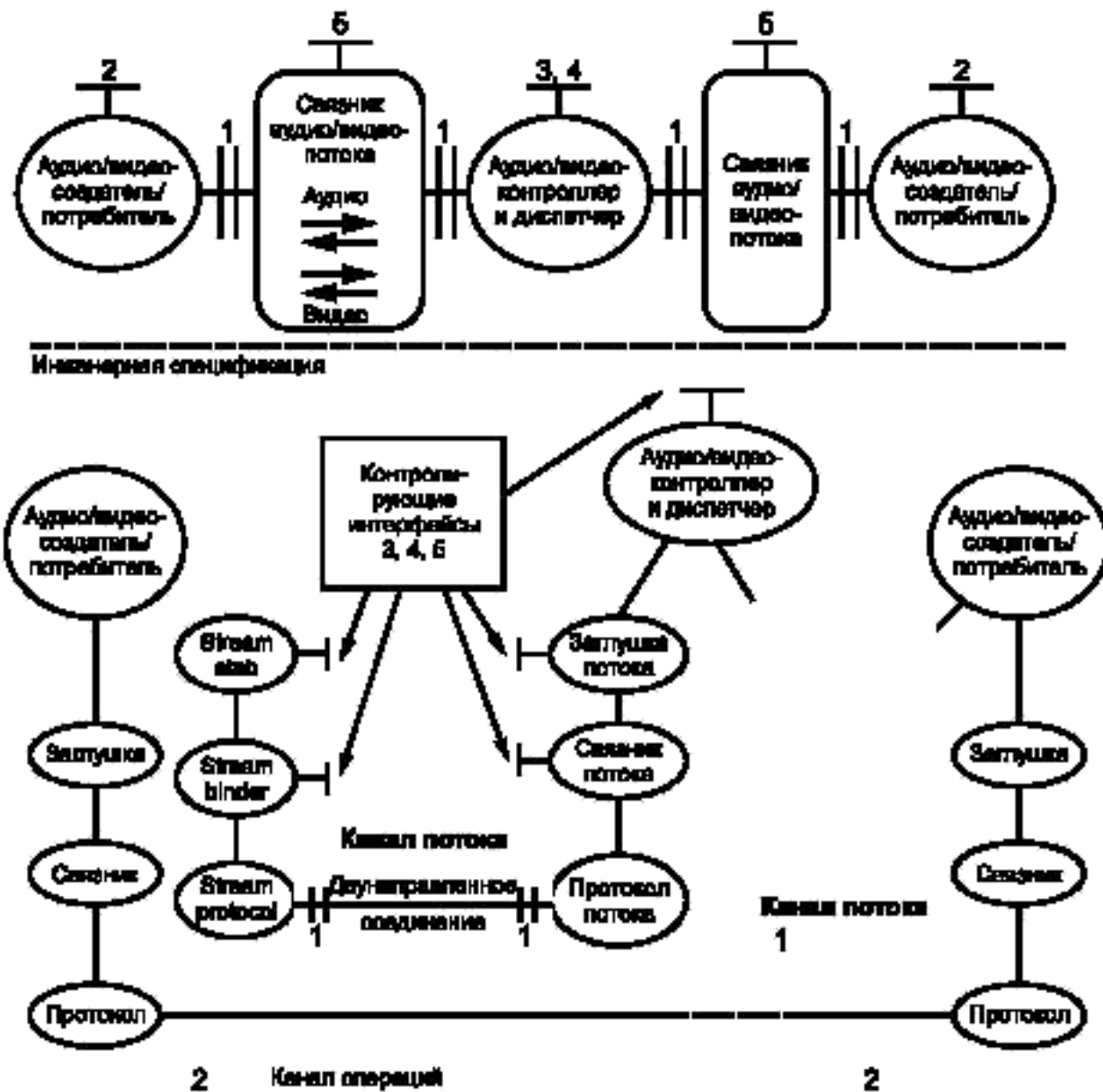
Рисунок 35 — Отображение вычислительной спецификации в инженерную
