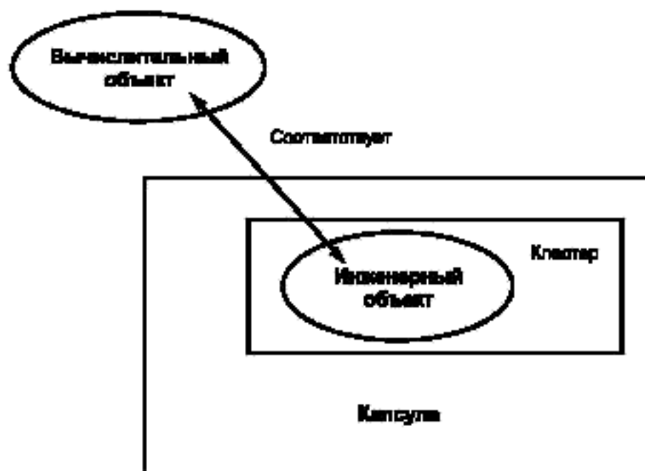
Рисунок 14 — Соответствие один-к-одному
