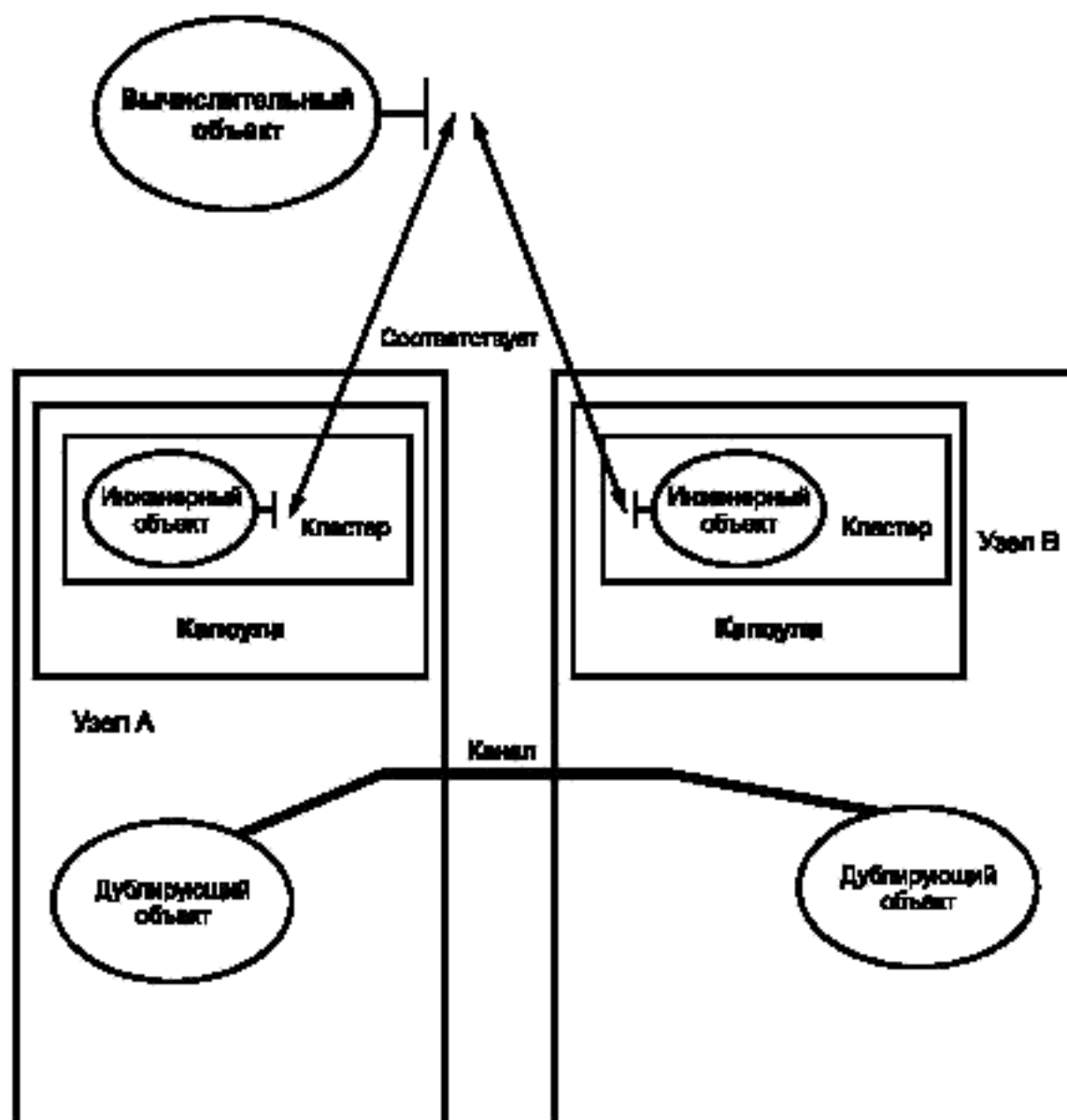
Рисунок 15 — Соответствие многие-одному
