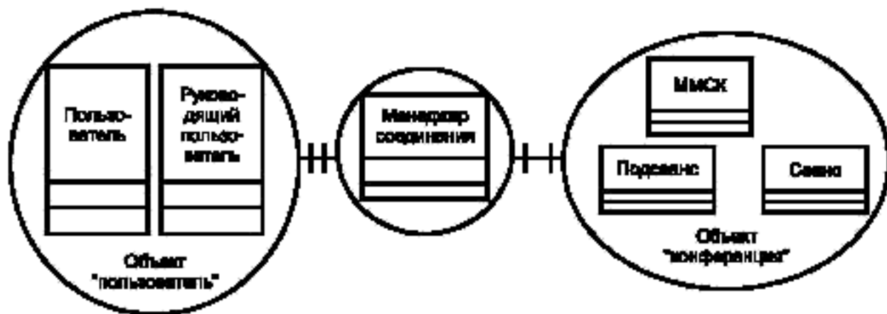
Рисунок 24 — Вычислительная конфигурация ММСК
