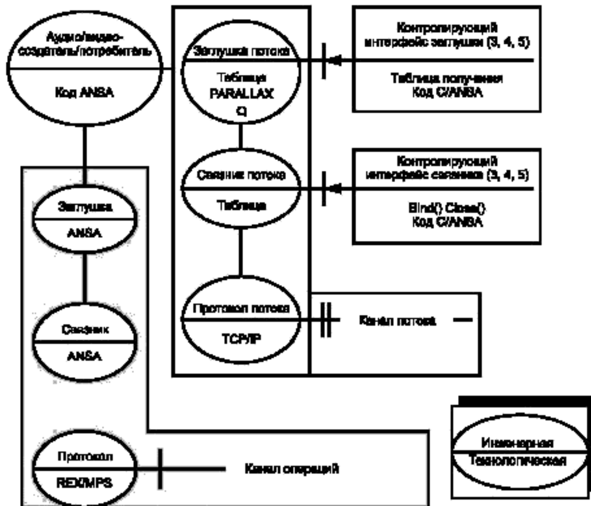
Рисунок 36 — Отображение инженерной спецификации в технологическую
