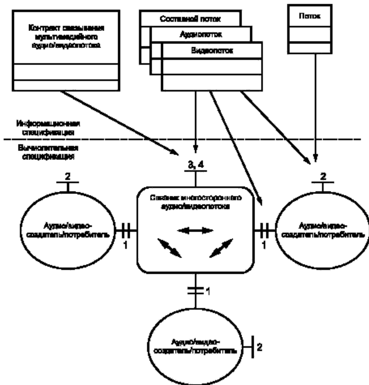
Рисунок 33 — Отображение информационной спецификации в вычислительную
