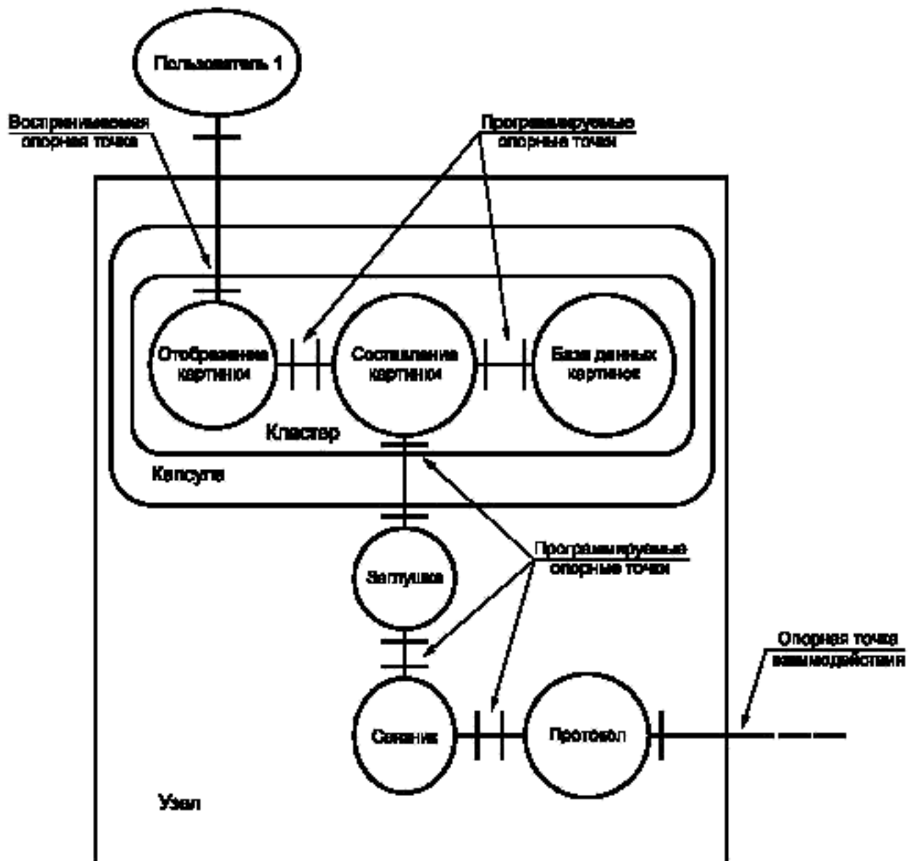
Рисунок 19 — Инженерная точка зрения (часть)
