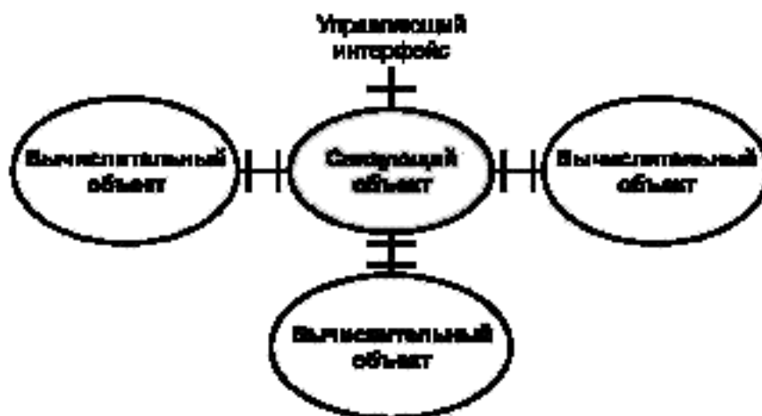
Рисунок 2 — Составное связывание
