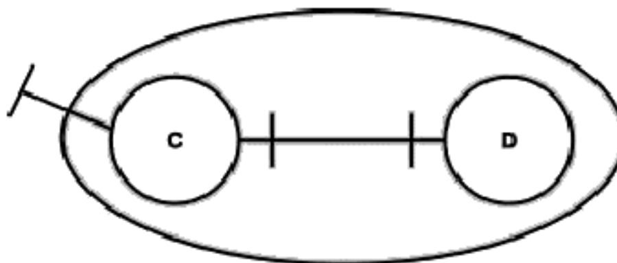
Рисунок 1 — Композиция объектов
