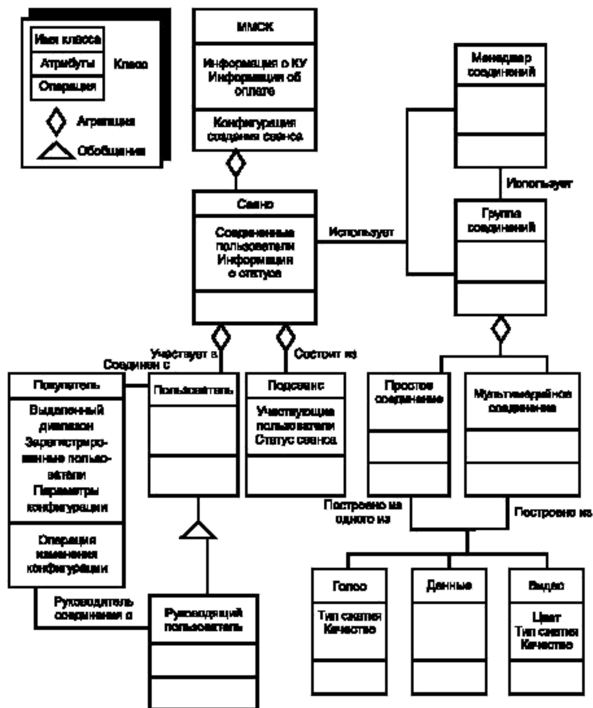
Рисунок 23 — Информационная спецификация
