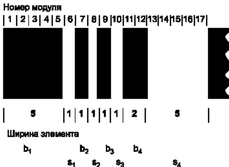
Рисунок 3 — Знак символа PDF417.
