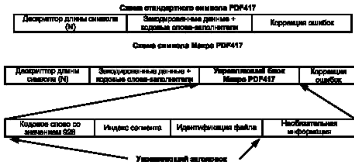
Рисунок Н.1 — Схемы символов PDF417
