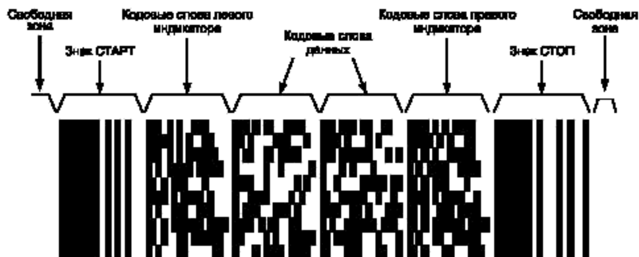
Рисунок 1 — Структура символа PDF417.
