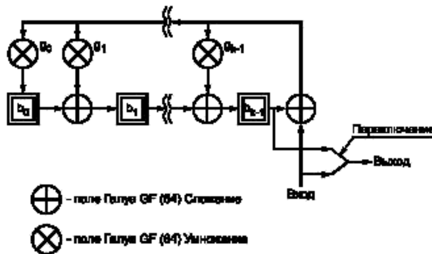
Рисунок 7 — Схема кодирования кодовых слов коррекции ошибок
