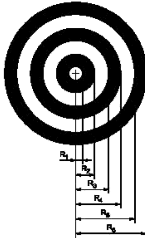
Рисунок 9 — Размеры шаблона поиска MaxiCode
