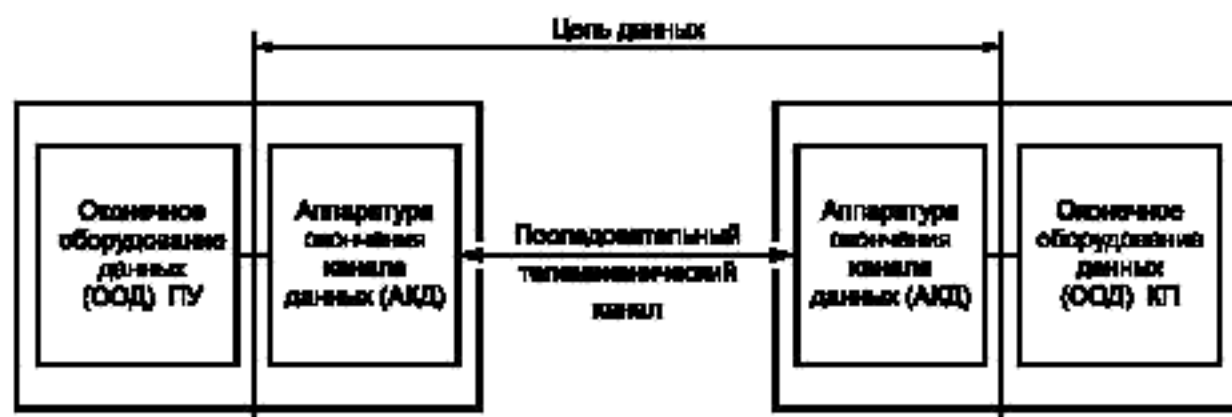
Рисунок 2 — Интерфейсы и соединения между ПУ и КП
