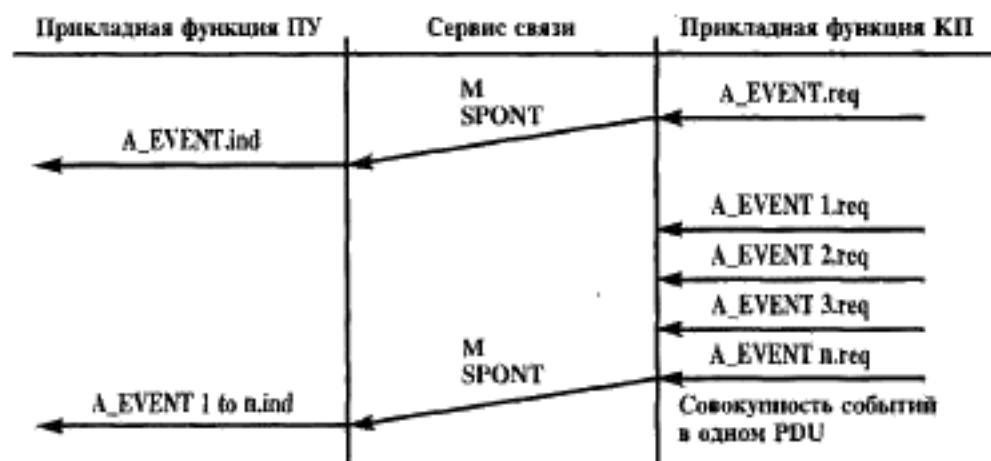
Рисунок 12 — Последовательная процедура сбора данных о событиях
