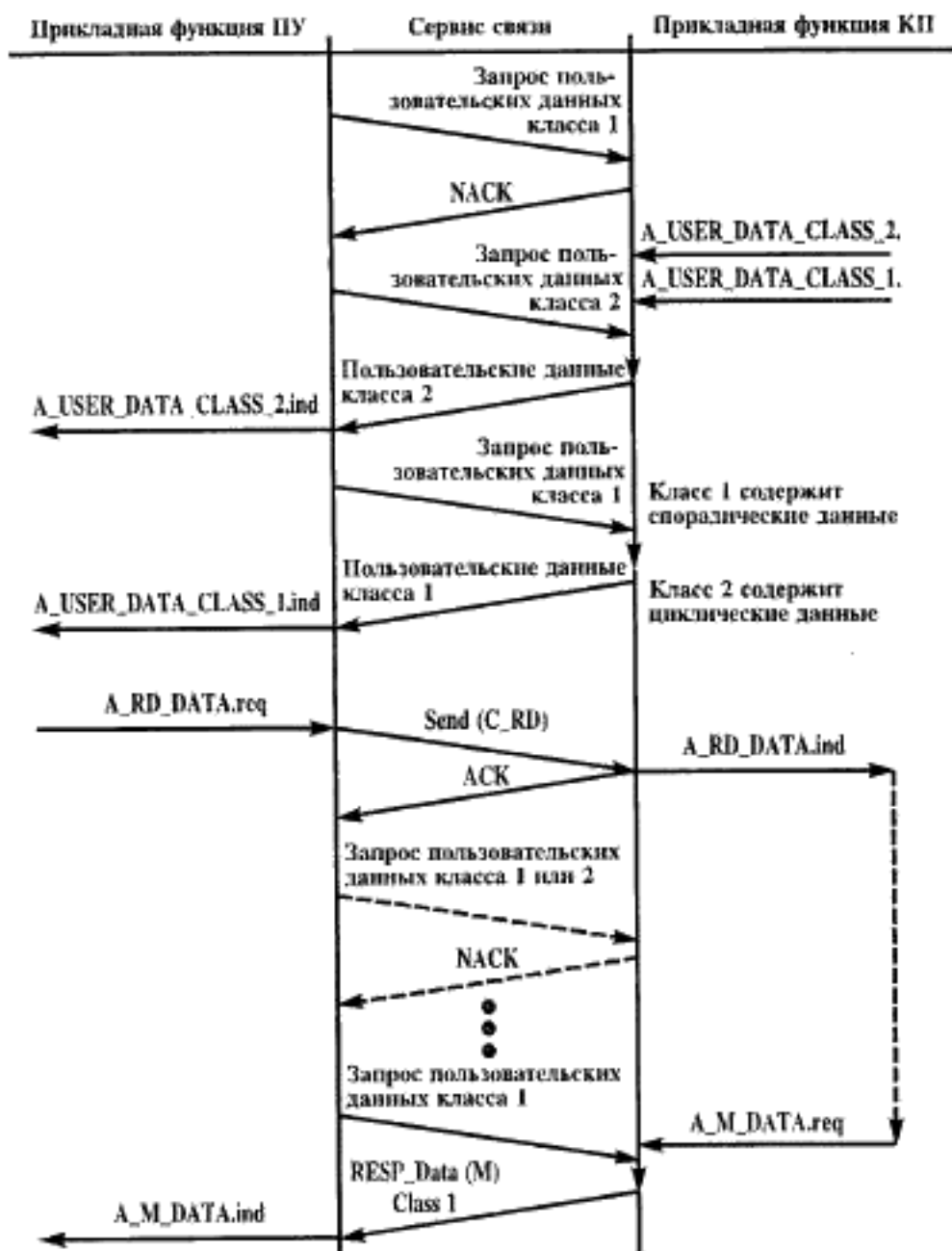
Рисунок 10 — Последовательная процедура — процедура опроса
