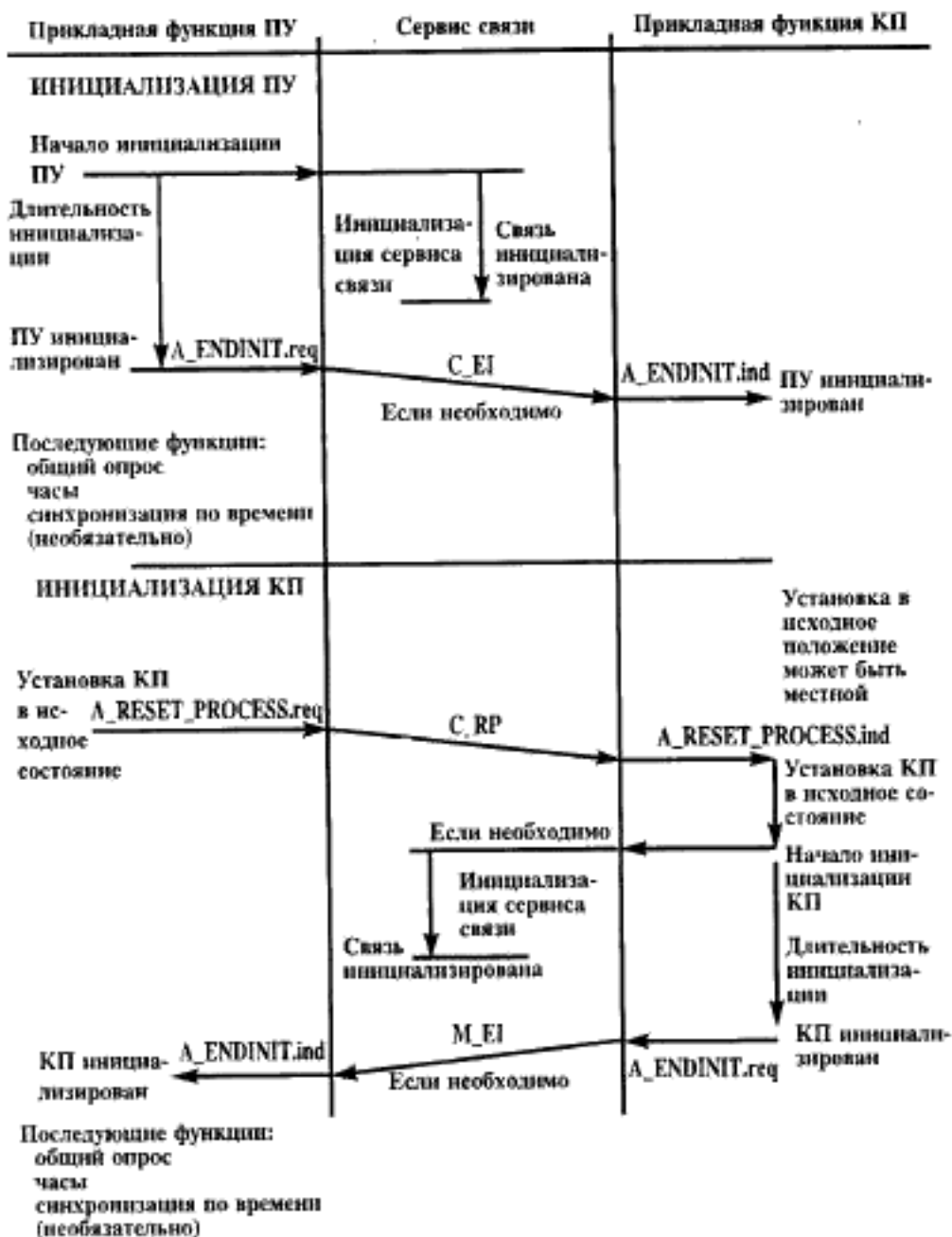
Рисунок 3 — Последовательная процедура — основная процедура инициализации
