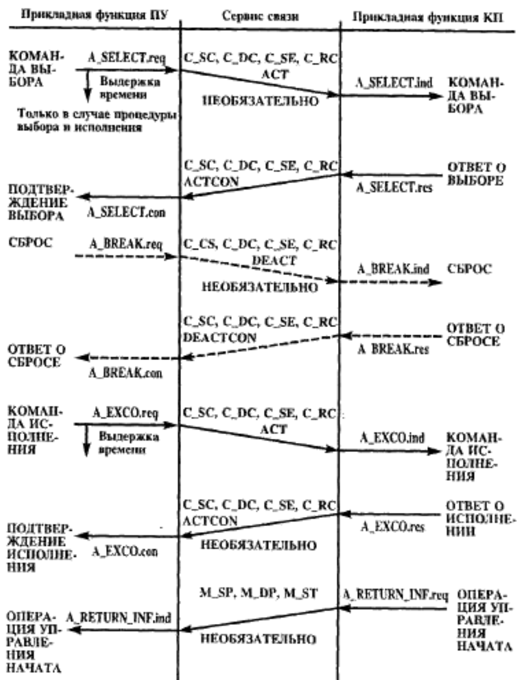
Рисунок 16 — Последовательная процедура — процедура передачи команда, лист 1
