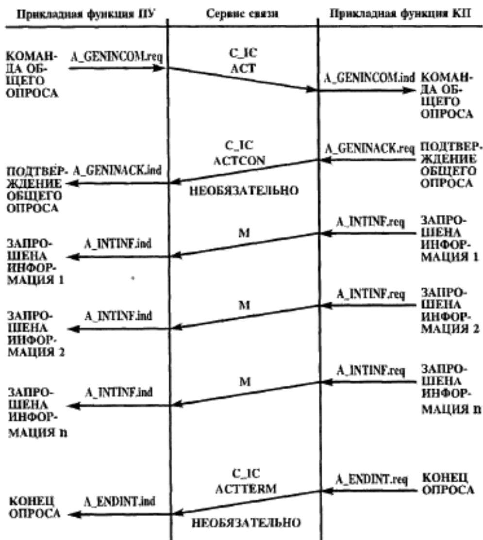
Рисунок 14 — Последовательная процедура — процедура опроса подстанций
