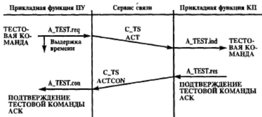
Рисунок 19 — Последовательная процедура — тестовая процедура
