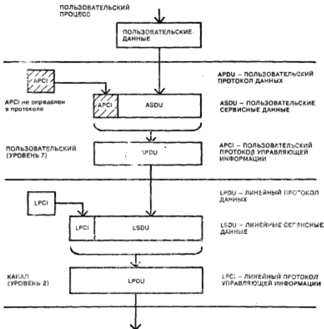
Рисунок 4 — Связи между блоками данных
