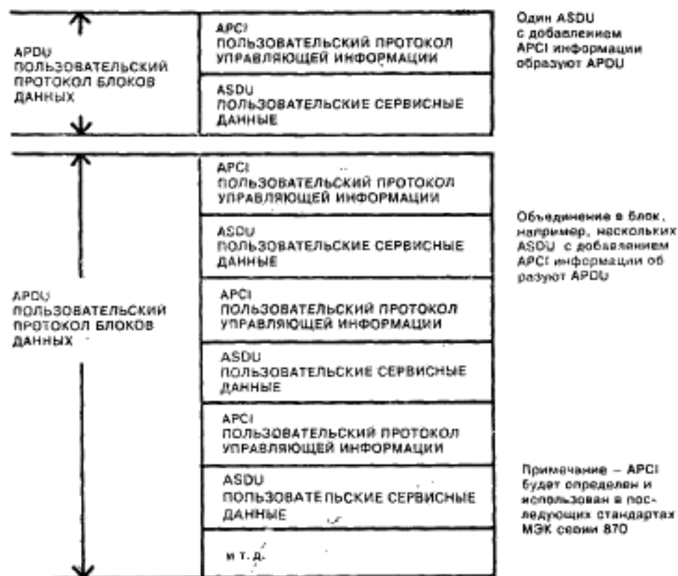
Рисунок 5 — Общая структура ПОЛЬЗОВАТЕЛЬСКОГО ПРОТОКОЛА БЛОКОВ ДАННЫХ
