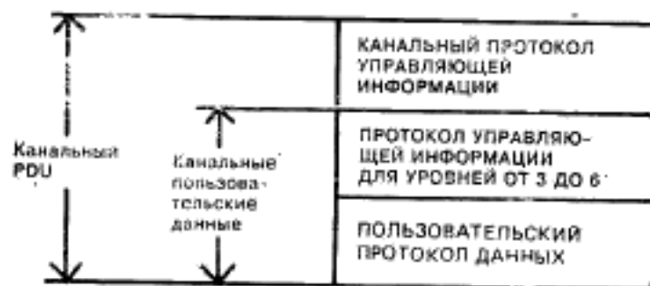
Рисунок 2 — Структура кадра для модели 1
