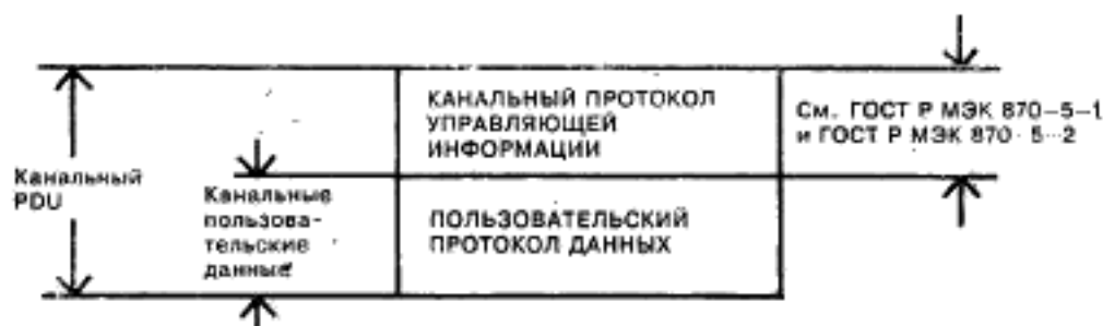
Рисунок 3 — Структура кадра для модели 2
