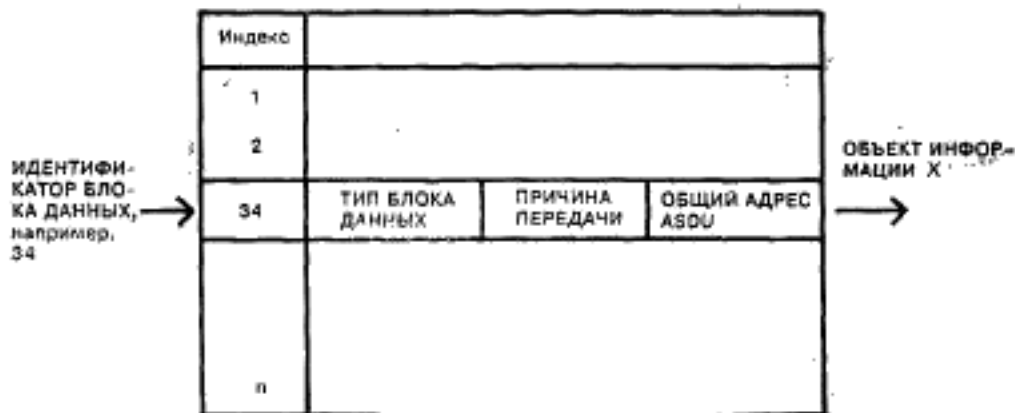
Рисунок 9 — Пример компактной идентификации ОБЪЕКТОВ ИНФОРМАЦИИ
