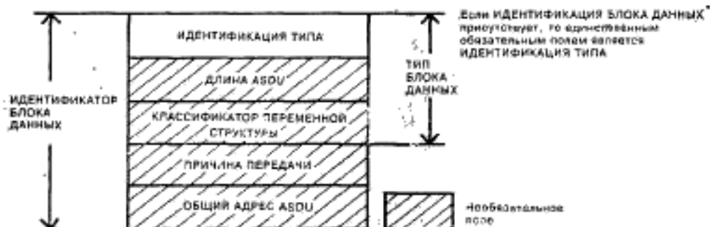
Рисунок 7 — Основная структура ИДЕНТИФИКАТОРА БЛОКА ДАННЫХ
