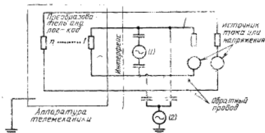
Схема для аналоговых входных сигналов
