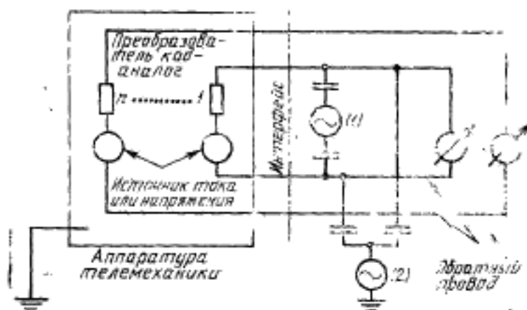
Схема для аналоговых выходных сигналов
