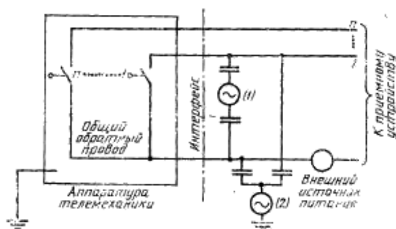
а) схема для пассивных двоичных выходных сигналов
