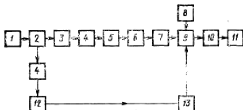
Схема установки для определения временного разрешения
