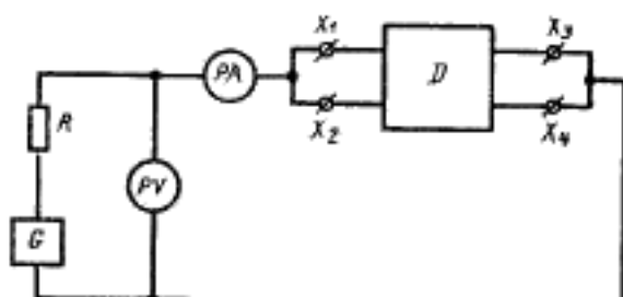
PA —измеритель тока; X 1 , X 2 —входные контакты; D —измерительный прибор; X 3 , X 4 —выходные контакты; R —защитный резистор; PV —измеритель напряжения; G —генератор тока
