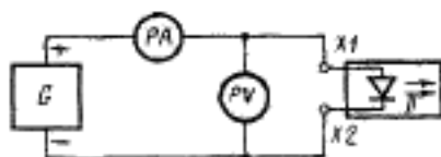
PA—измеритель тока; G—генератор тока; PV—измеритель напряжения; X1, X2—контакты подключения измеряемого прибора; D—измеряемый прибор.
