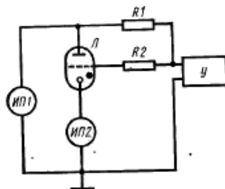
R1, R2 — резисторы; ИП1 — измеритель напряжения; ИП2 — измеритель тока; L — испытываемый тиратрон; U — регулируемый источник постоянного напряжения.
