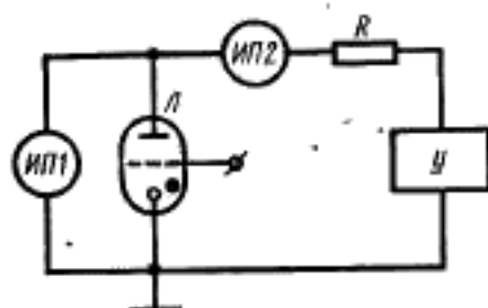
R — резистор; ИП1 — измеритель напряжения; ИП2 — измеритель тока; L — испытуемый тиратрон (газотрон); U — регулируемый источник постоянного напряжения
