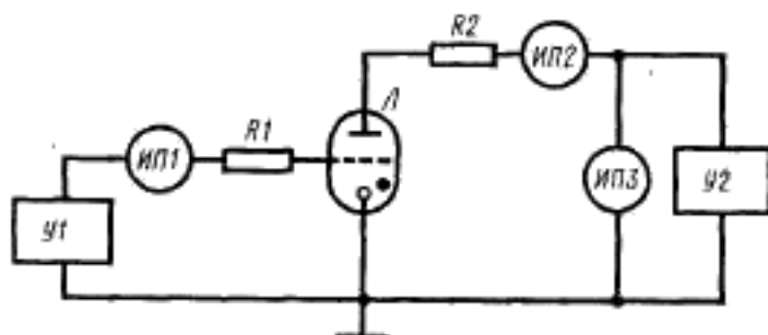
R1, R2 — резисторы; ИП1, ИП2 — измерители тока; ИП3 — измеритель напряжения; L — испытываемый тиратрон; У1, У2 — регулируемые источники постоянного напряжения
