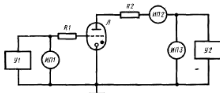
R1 , R2 —резисторы; ИП1 , ИП3 —измерители напряжения; ИП2 —измеритель тока; Л —испытываемый тириатрон; У1 , У2 —регулируемые источники постоянного напряжения
