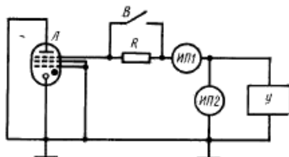
R — резистор; B — выключатель; ИП1 — измеритель тока; ИП2 — измеритель напряжения; L — испытываемый тиратрон; У — регулируемый источник постоянного напряжения
