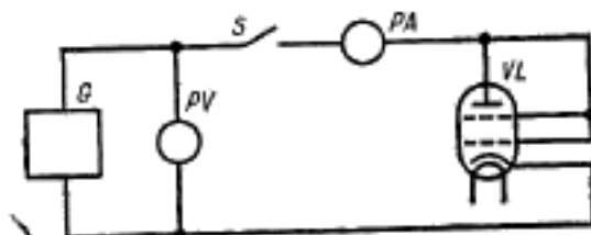
PV —вольтметр постоянного тока; PA —миллиамперметр постоянного тока; S —выключатель; VL —испытываемая лампа; G —источник напряжения постоянного тока.
