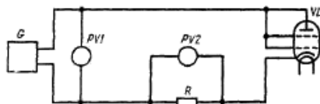
PV1—PV2—электронные импульсные вольтметры; G—генератор импульсного напряжения; R—резистор; VL—испытываемая лампа.
