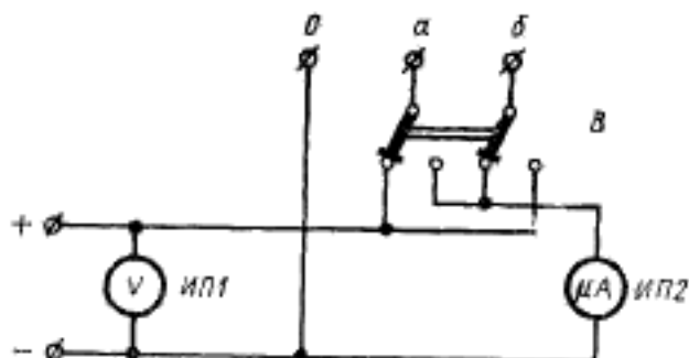
ИП1 — вольтметр постоянного тока; В — переключатель полярности напряжения; а и б — контакты, предназначенные для присоединения электродов, металлического баллона или подогревателя, между которыми измеряют сопротивление изоляции; в — контакт, являющийся общей точкой схемы; ИП2 — электронный или магнитоэлектрический микроамперметр постоянного тока
