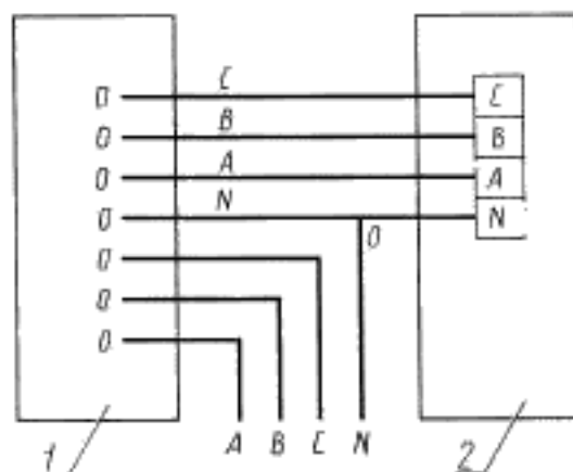
1 — автотрансформатор; 2 — испытуемое оборудование
