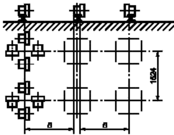
Рисунок Г.2 — Трансформаторы массой от 200 до 255 т
