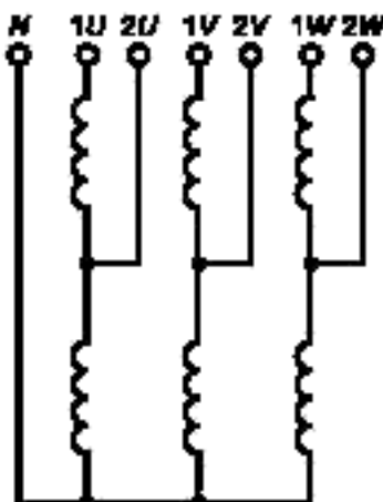
Рисунок Ж.7 — Маркировка трехфазного автотрансформатора ( Y_N авто/D-0)
