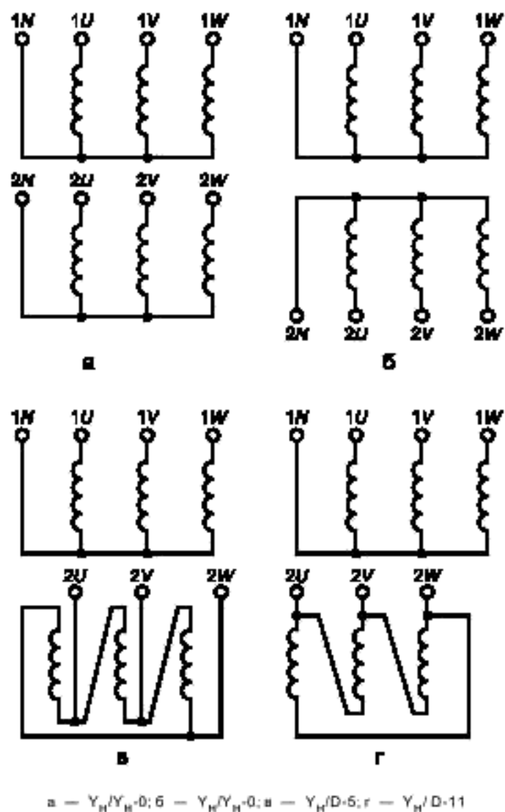
Рисунок Ж.4 — Маркировка трехфазных двухобмоточных трансформаторов
