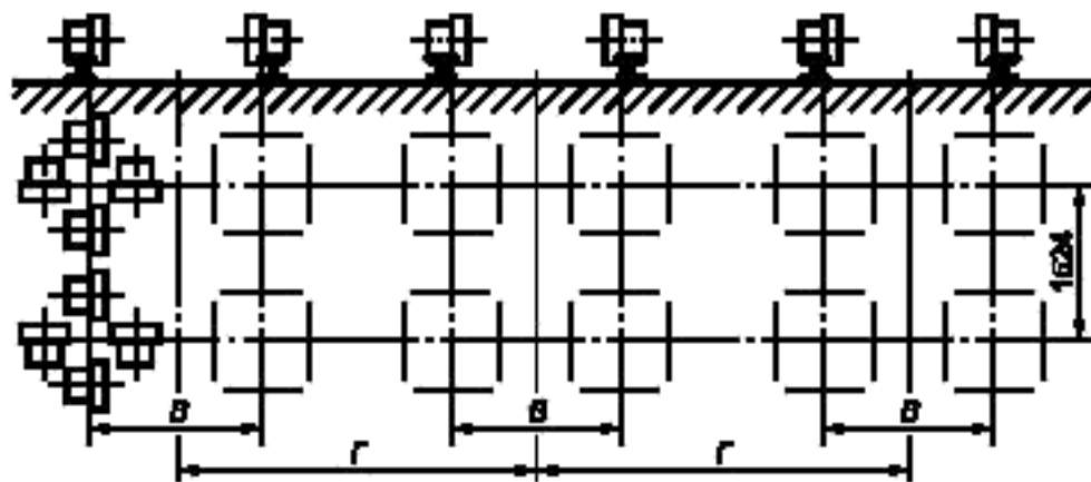
Рисунок Г.4 — Трансформаторы массой от 300 до 700 т
