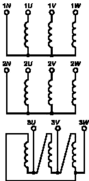
Рисунок Ж.5 — Маркировка трехфазного трехобмоточного трансформатора ( Y_N/Y_N/D-0-5 )
