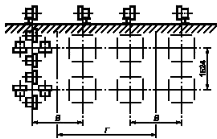
Рисунок Г.3 — Трансформаторы массой от 255 до 300 т
