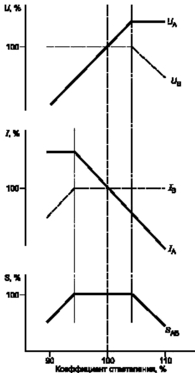
Рисунок 3 — Комбинированное регулирование напряжения (режим a )
