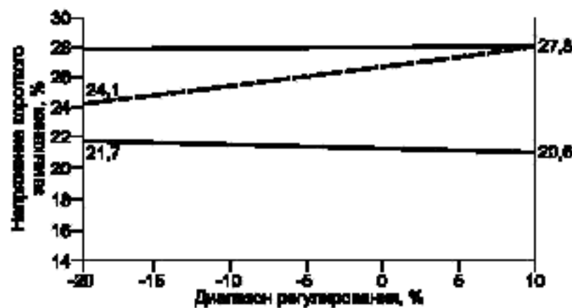
Рисунок В.1 — Диапазон изменения напряжения короткого замыкания
