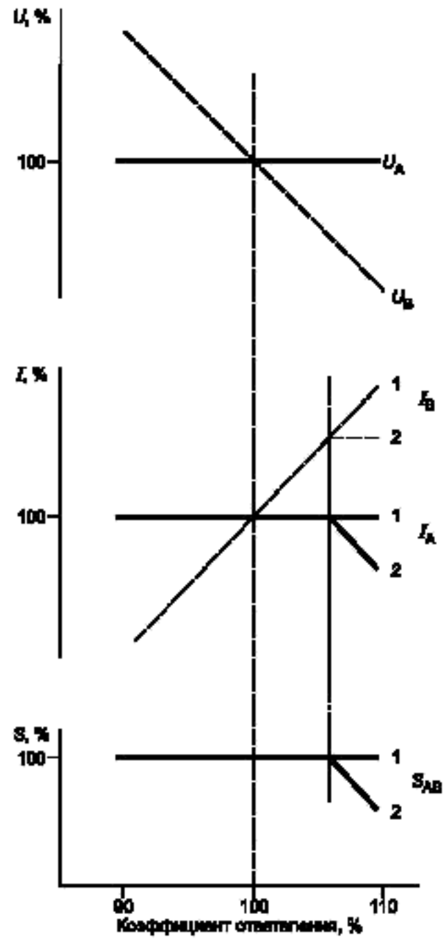
Рисунок 2 — Регулирование напряжения при переменном магнитном потоке (режим b )
