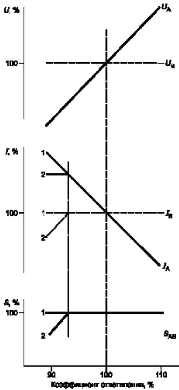
Рисунок 1 — Регулирование напряжения при постоянном магнитном потоке (режим a )
