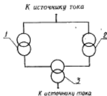
1 — испытуемый трансформатор; 2 — вспомогательный трансформатор; 3 — промежуточный трансформатор
