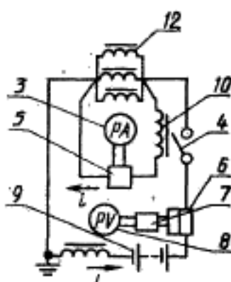
1 — питающий трансформатор; 2 — измеряемая обмотка (первичная); 3 — микроамперметр; 4 — выключатель; 5 — фильтр; 6 — шунт; 7 — фильтр; 8 — милливольтметр; 9 — аккумуляторная батарея; 10 — дроссель; 11 — индуктивность; 12 — измеряемая обмотка (вторичная)
