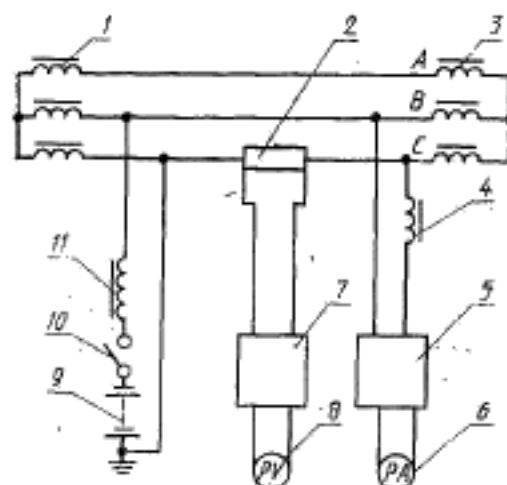
1 — питающий трансформатор; 2 — шунт; 3 — измеряемая обмотка; 4 — индуктивность; 5 — фильтр; 6 — микроамперметр; 7 — фильтр; 8 — милливольтметр; 9 — аккумуляторная батарея; 10 — выключатель; 11 — дроссель
