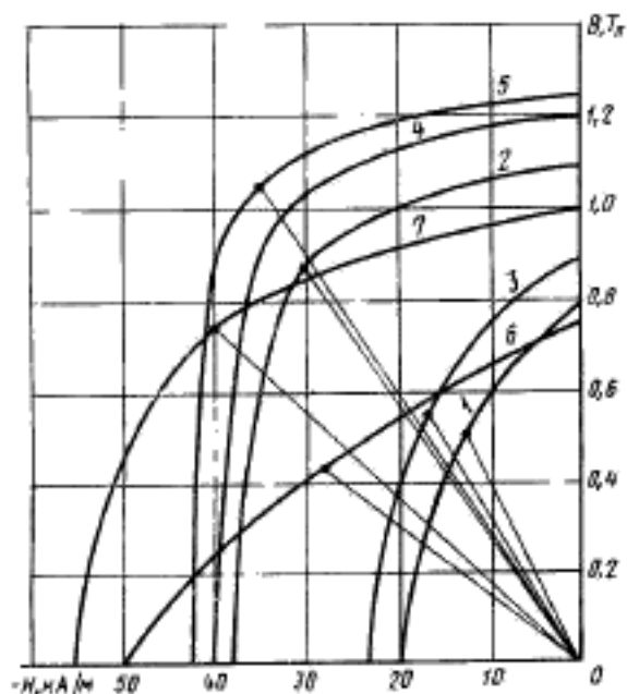
1—28Х10К; 2—28Х10КА; 3—25Х15К; 4—25Х15КА; 5—23Х15К5ФА; 6—30Х23К; 7—30Х23КА
