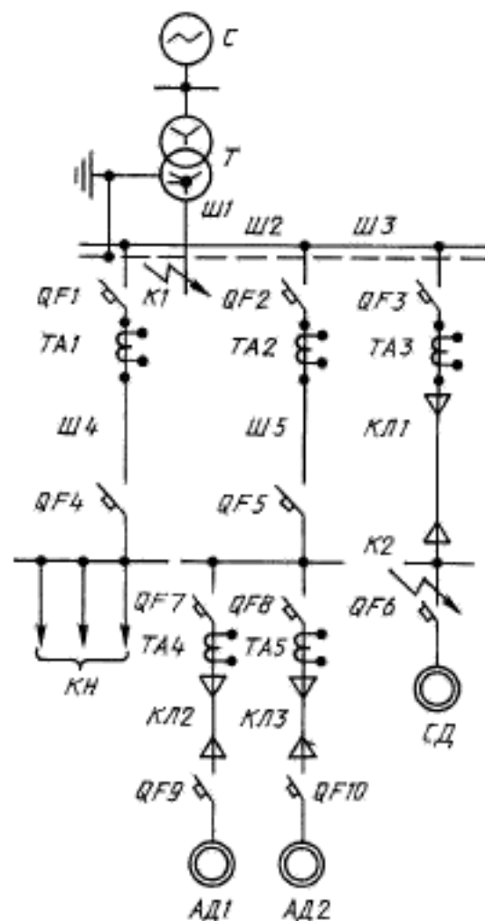
Расчетная схема к примеру 2
