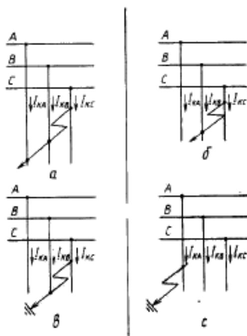
а—трехфазное КЗ K^{(3)} ; б—двухфазное КЗ— K^{(2)} , в—двухфазное КЗ на землю— K^{(1,1)} ; с—однофазное КЗ на землю— K^{(1)}
