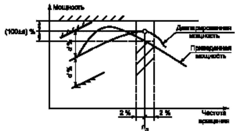
Рисунок 2 — График для декларируемого значения частоты вращения с максимальной мощностью
