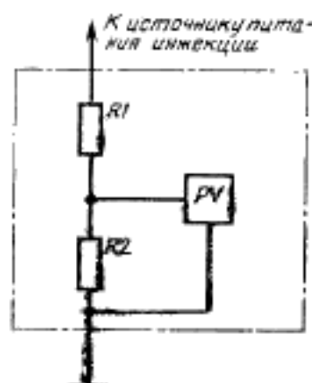
R1, R2 — резисторы делителя; PV — импульсный вольтметр
