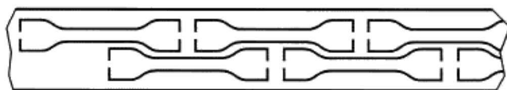
Рисунок 15 — Образцы, вырубленные ножом с выемкой
