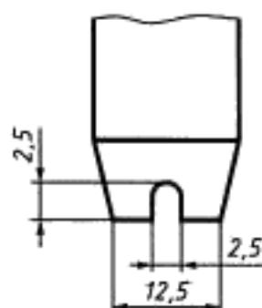
Рисунок 14 — Конеч вырубного ножа с выемкой
