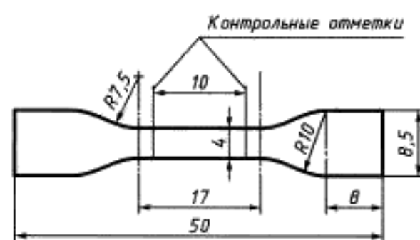
Рисунок 13 — Образец в виде двусторонней лопатки уменьшенного размера
