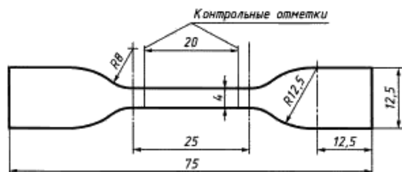
Рисунок 12 — Образец в виде двусторонней лопатки
