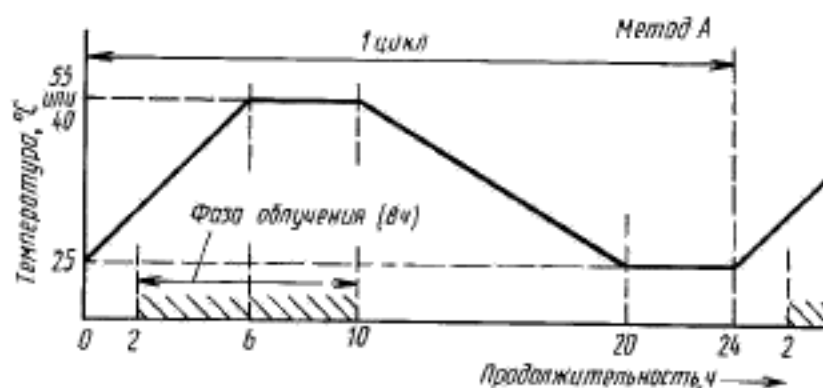
Режим облучения и зависимость температуры от времени
