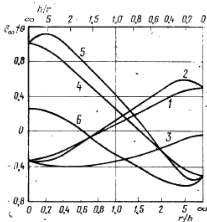
Зависимость отношения \delta_{\infty} \cdot \theta от формы цилиндрического детектора радиуса r и полувысоты h для случаев 1–6 таблицы приложения 6
