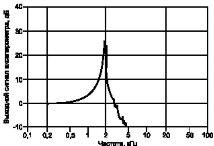
Рисунок 8 — Типичная частотная характеристика акселерометра с щупом
