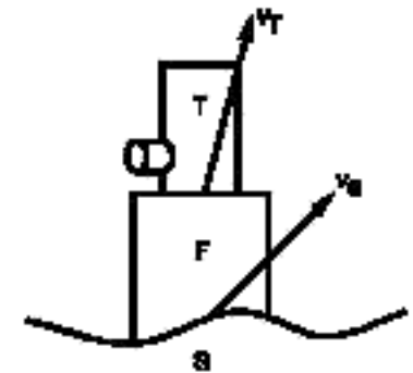
Рисунок 1 — Схематическое изображение установки акселерометра
