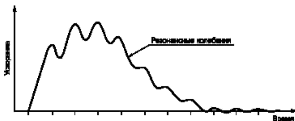
Рисунок 4 — Отклик акселерометра на удар
