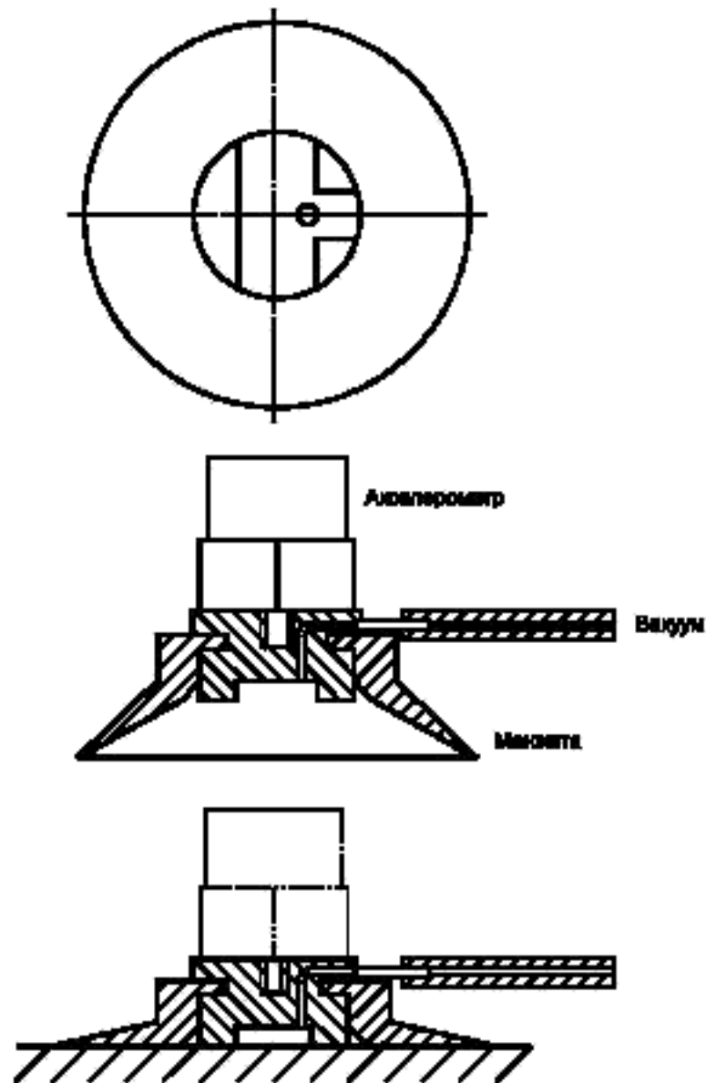
Рисунок 11 — Вакуумное крепление
