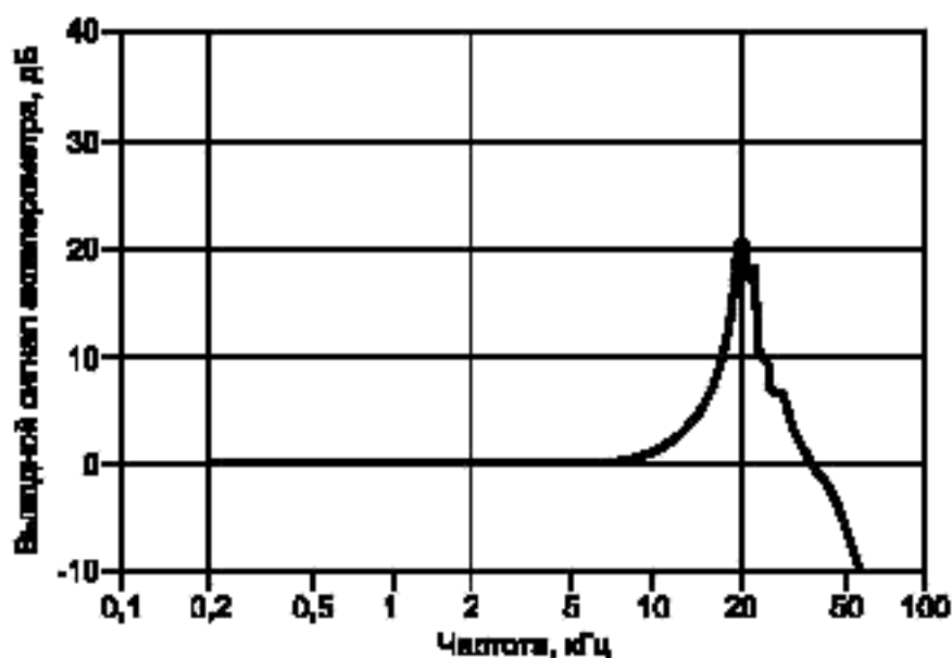
Рисунок 9 — Типичная частотная характеристика акселерометра на магните
