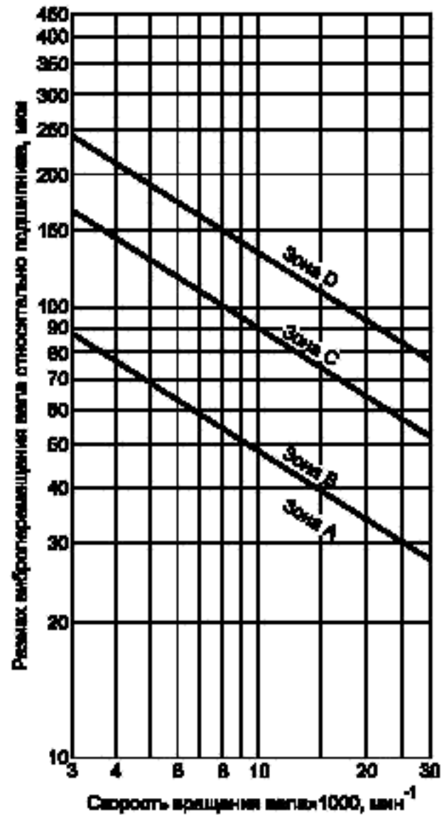
Рисунок А.1 — Рекомендуемые значения максимальной относительной перемещения вала в зависимости от максимальной рабочей скорости вращения вала агрегата
