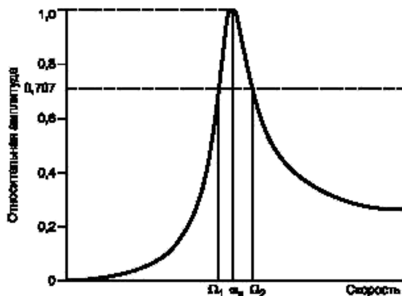
Рисунок 5 — Диаграмма Бодe для оценки модальной чувствительности
