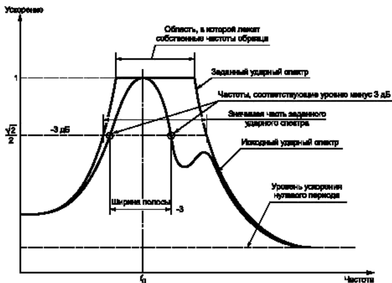
Рисунок 3 — Типичная огибающая спектра ответа
