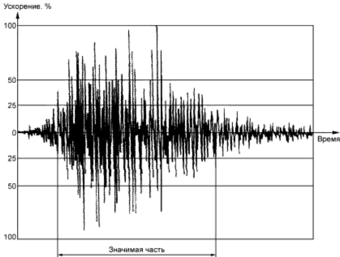
Рисунок 4 — Типичная форма акселерограммы
