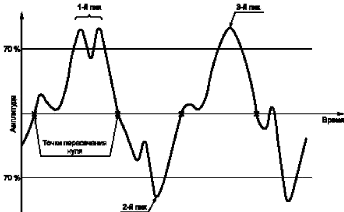
Рисунок 2 — Пример обнаружения пиков отклика, превышающих пороговое значение (70 %)
