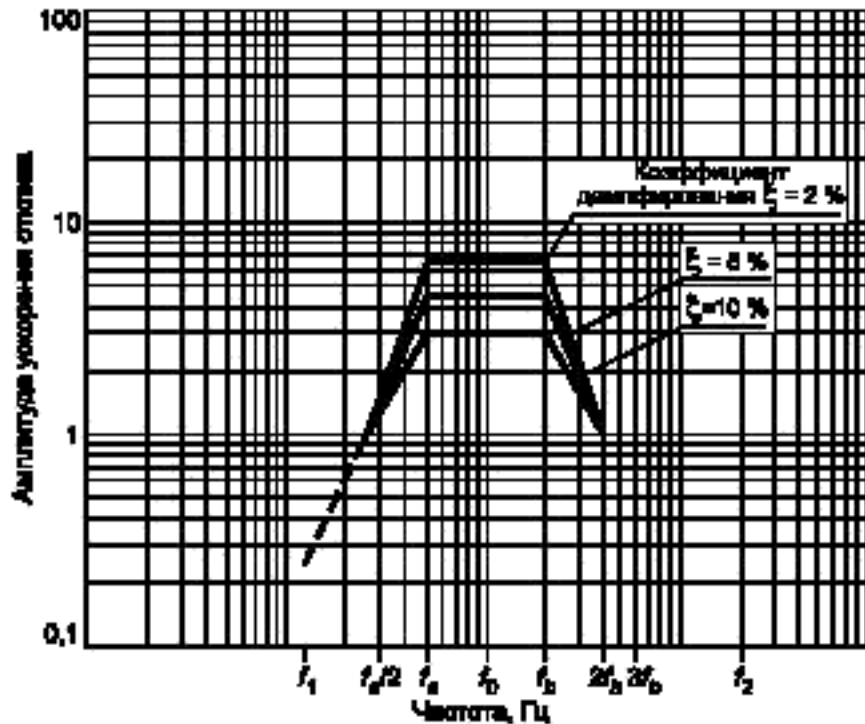
Рисунок — Категория 2. Рекомендуемый вид заданного спектра ответа
