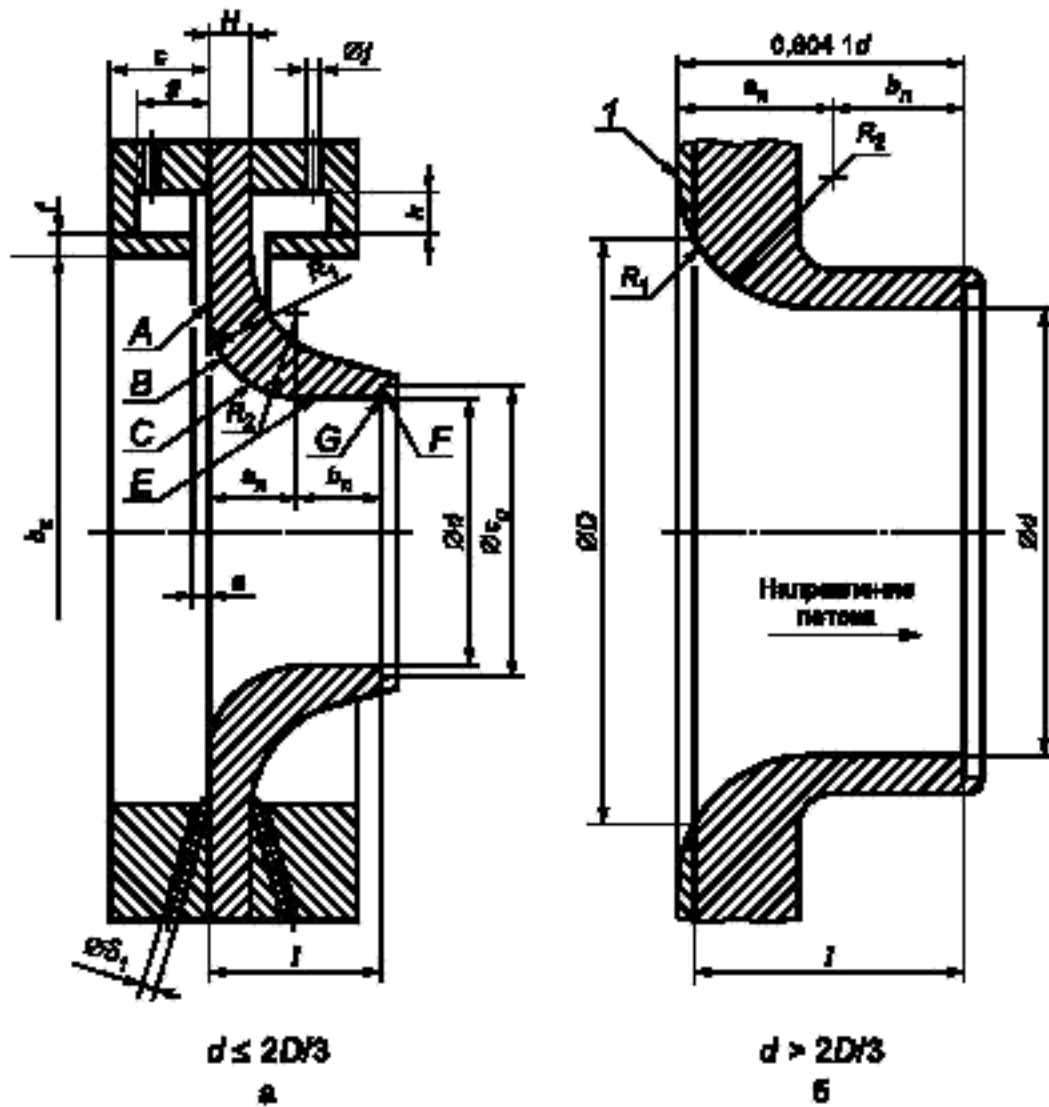
Рисунок 1 — Сопло ИСА 1932
