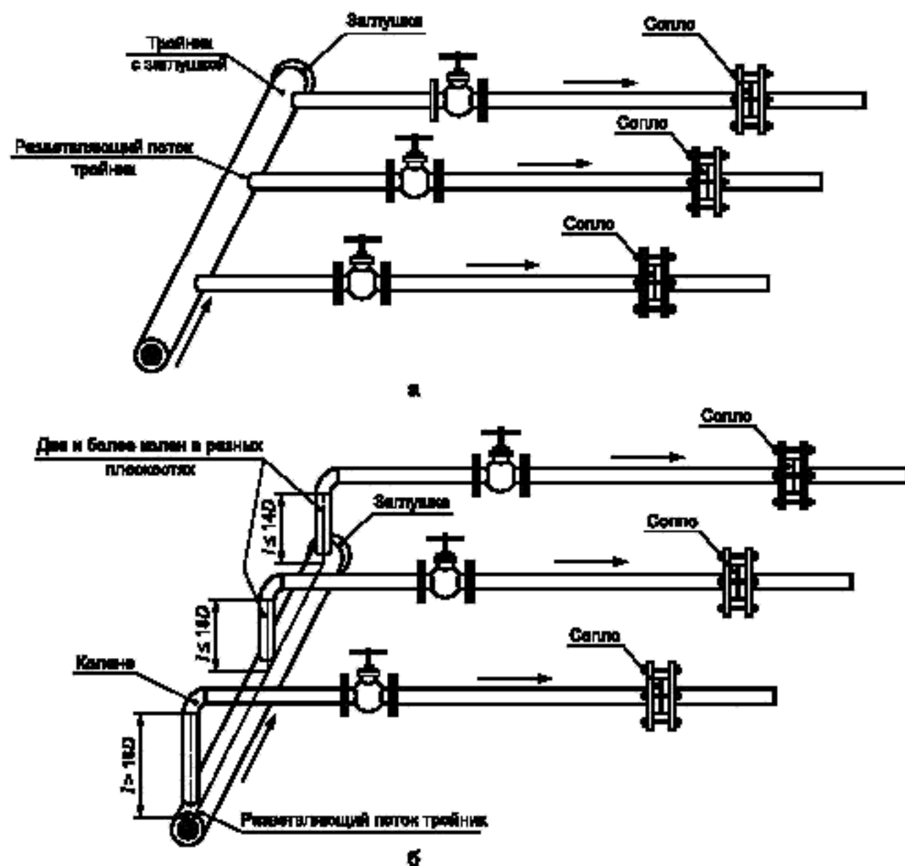
Рисунок 5 — Схемы коллектора
