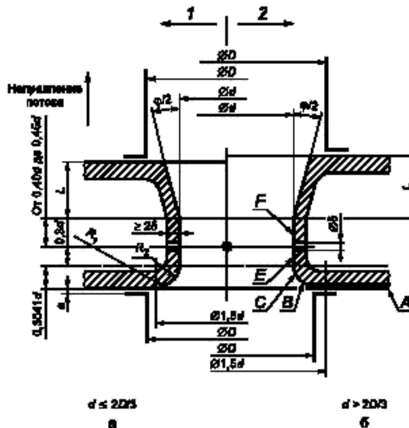
1 — укороченное сопло Вентури; 2 — неукороченное сопло Вентури
