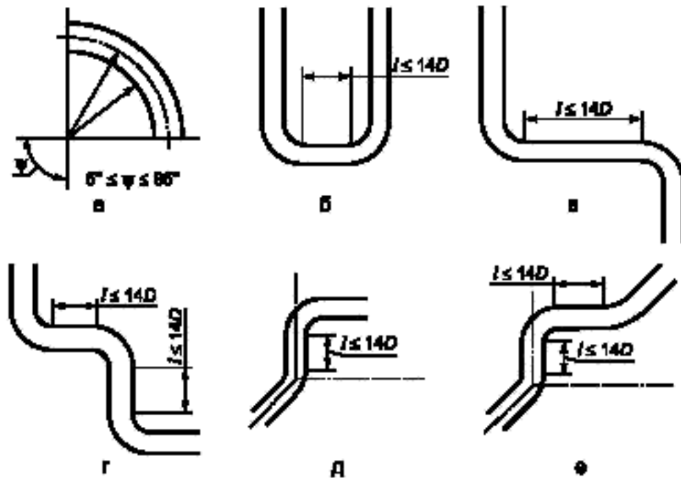
Рисунок А.1 — Колено и группы колен
