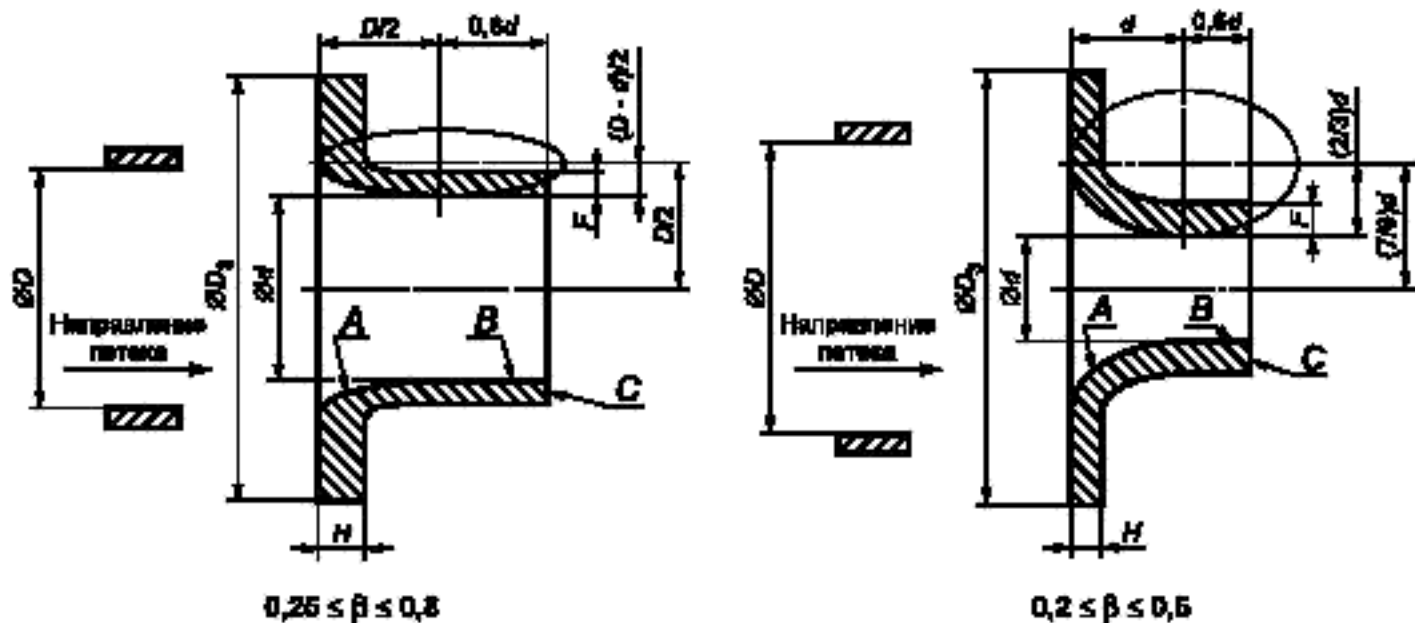
Рисунок 2 — Эллипсное сопло
