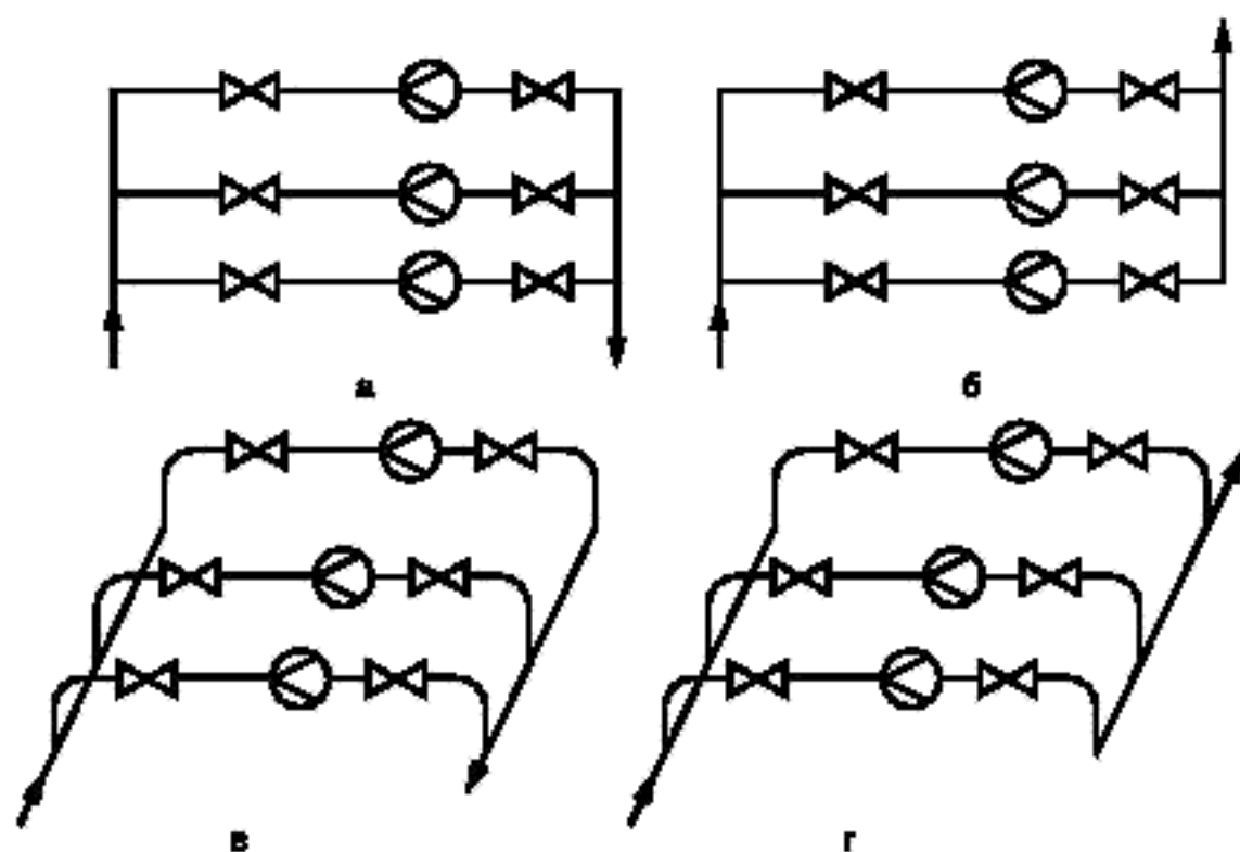
Рисунок А.4 — Схемы коллекторных систем
