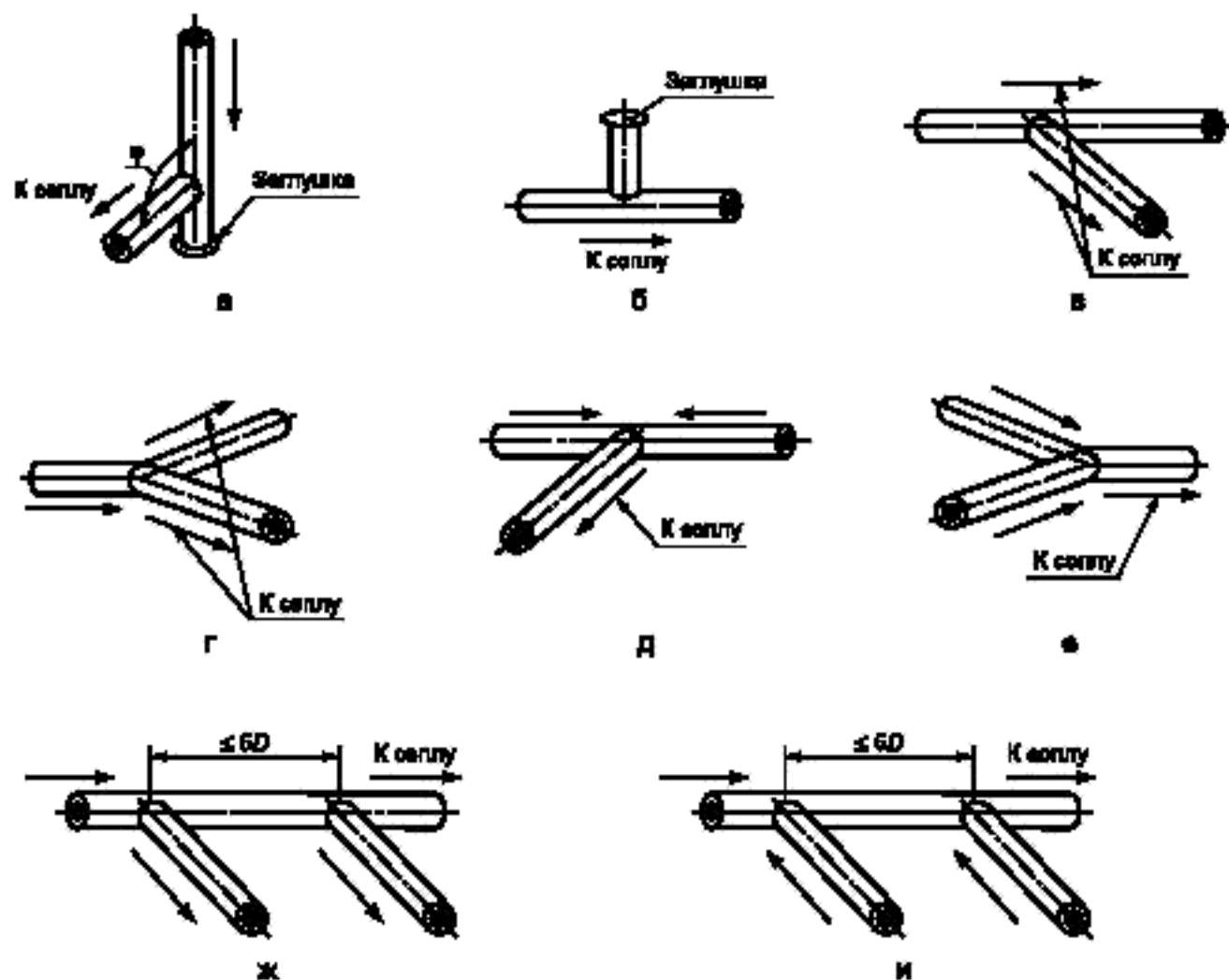
Рисунок А.2 — Тройники
