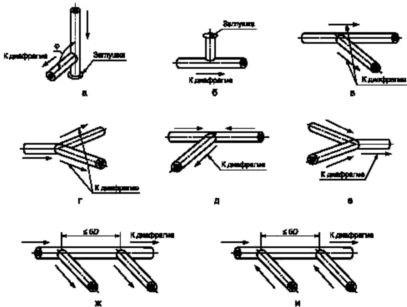
Рисунок А.2 — Тройники
