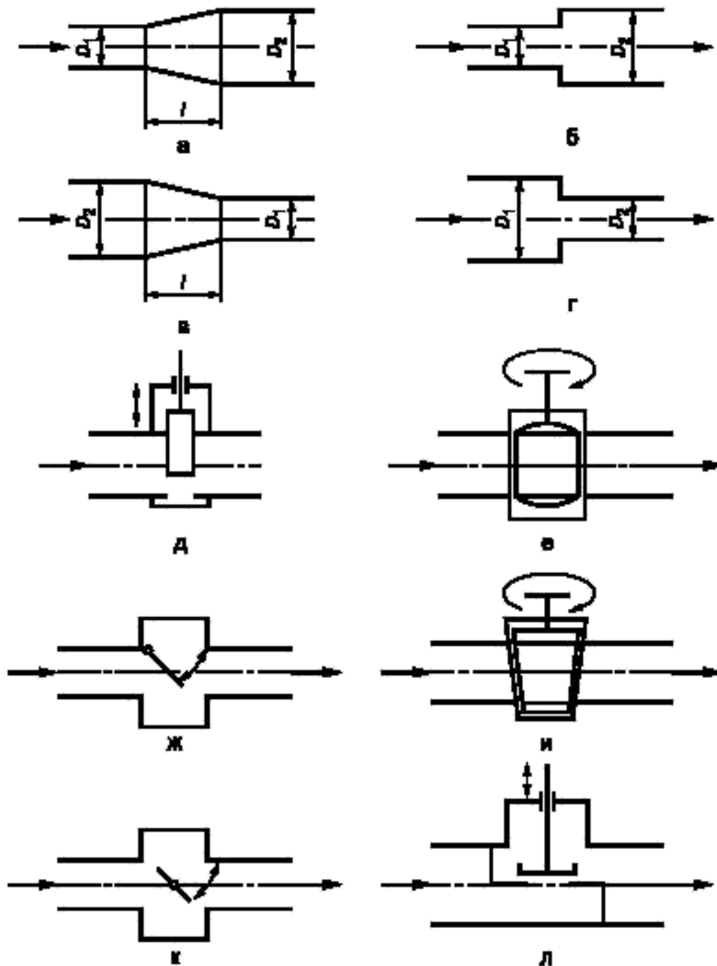
Рисунок А.3 — Переходные участки и запорная арматура
