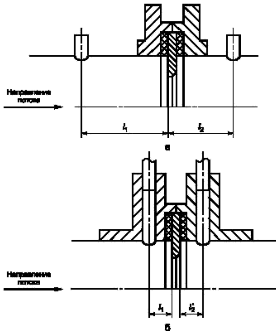
а — трехрадиусный отбор; б — фланцевый отбор
