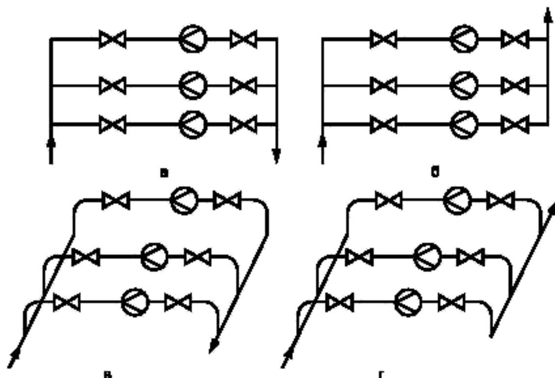
Рисунок А.4 — Схемы коллекторных систем
