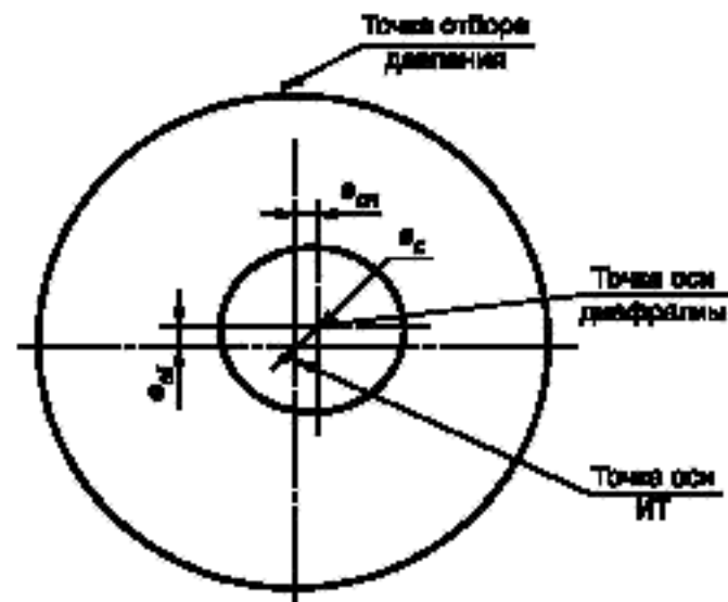
Рисунок 10 — Параметры эксцентриситета установки диафрагмы
