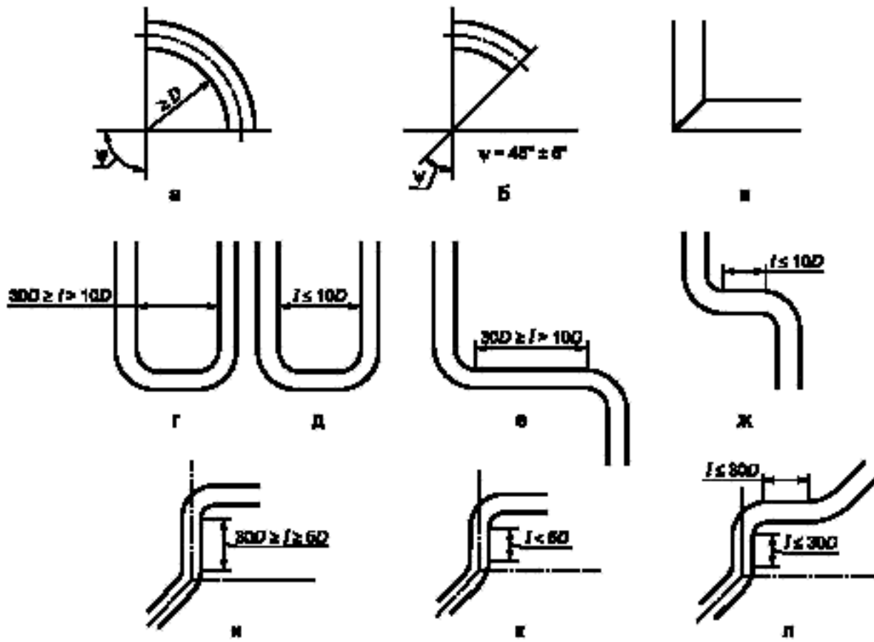
Рисунок А.1 — Колено и группы колен
