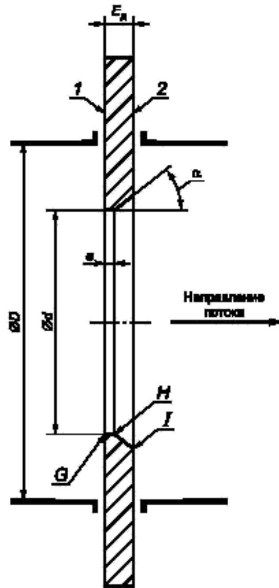
1 — входной торец диафрагмы; 2 — выходной торец диафрагмы
