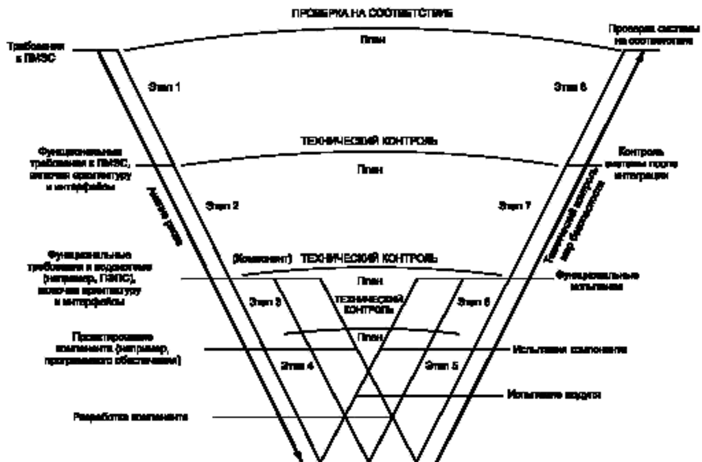
Рисунок DDD.1 — Модель ЦИКЛА РАЗРАБОТКИ для ПМЭС
