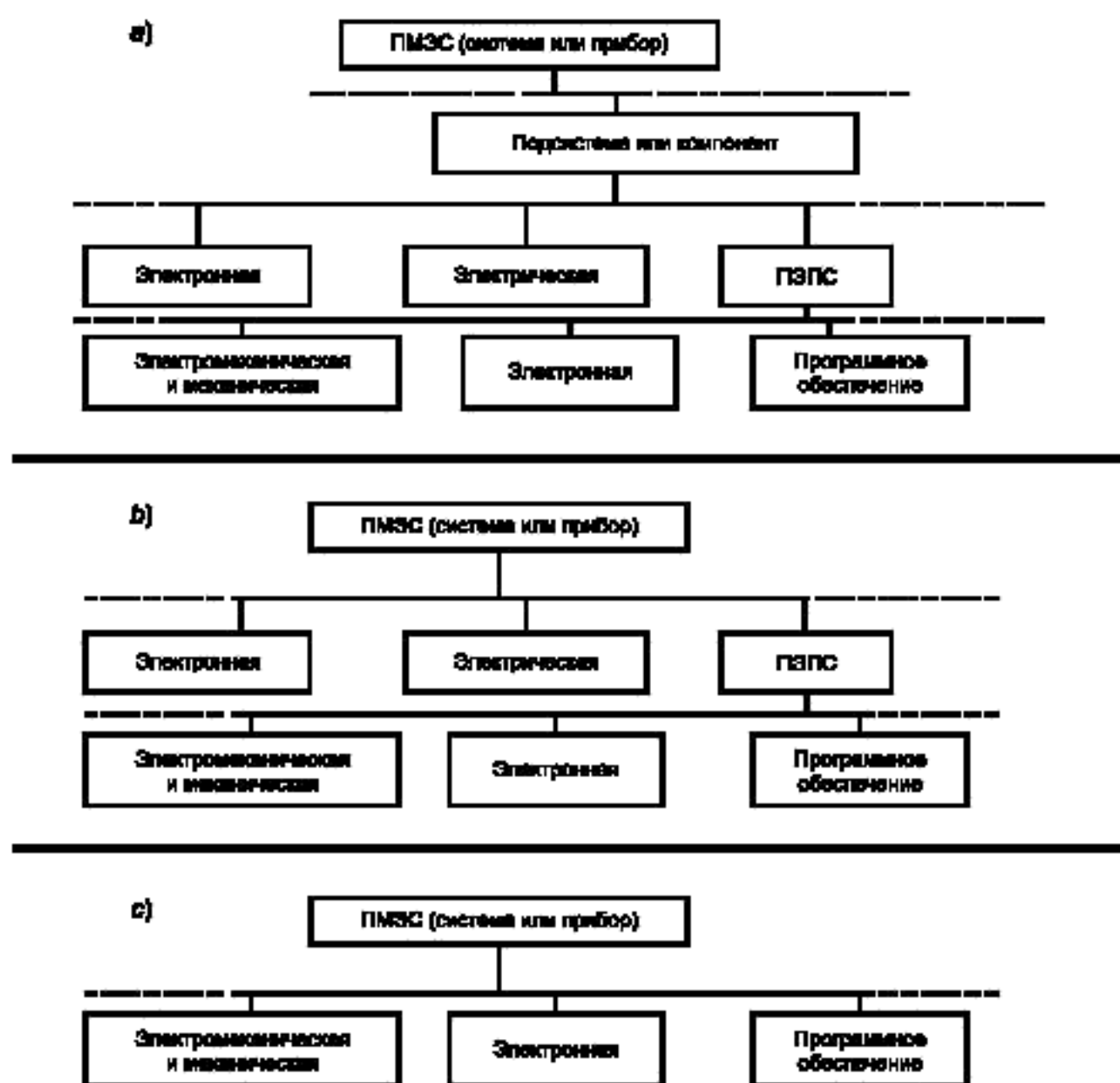
Рисунок ЕЕЕ.1 — Примеры структуры ПМЭС/ПЭПС
