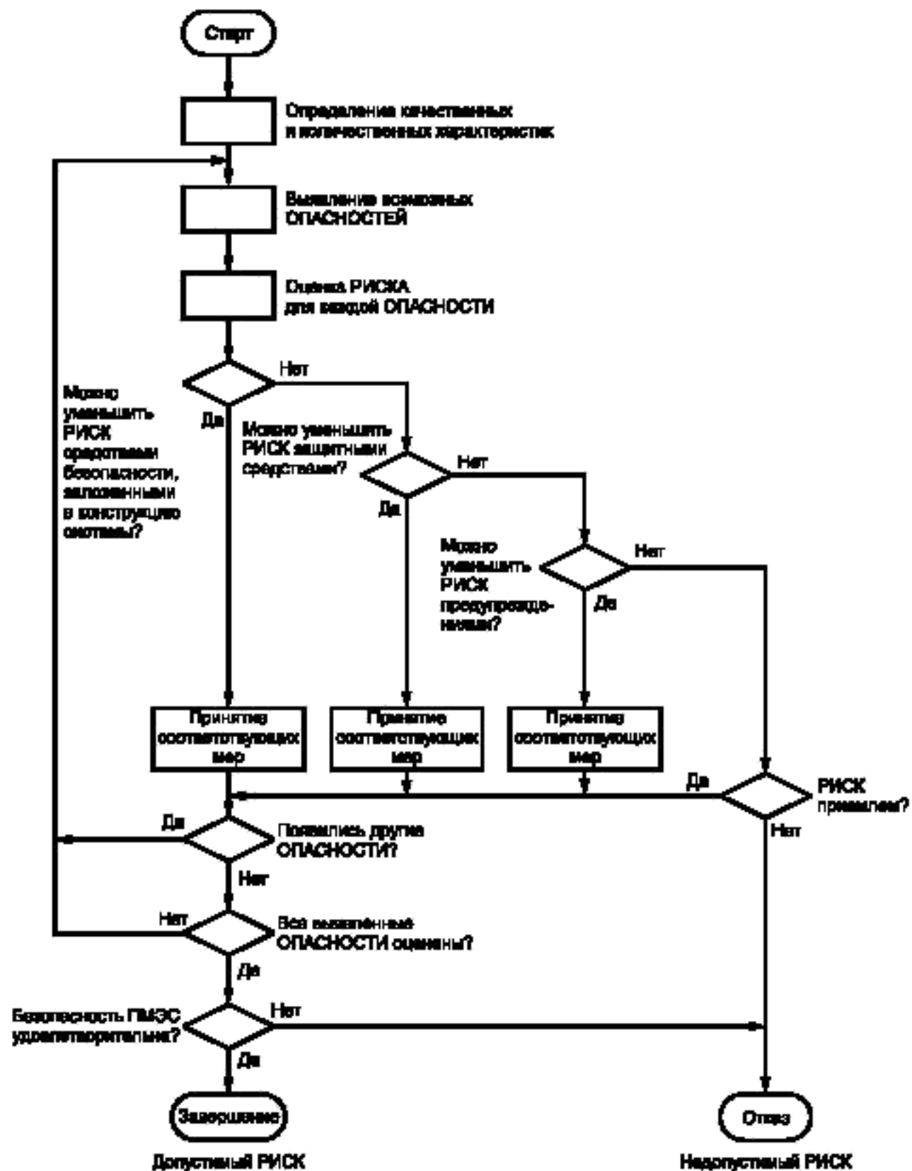
Рисунок ССС.2 — Процесс управления РИСКОМ
