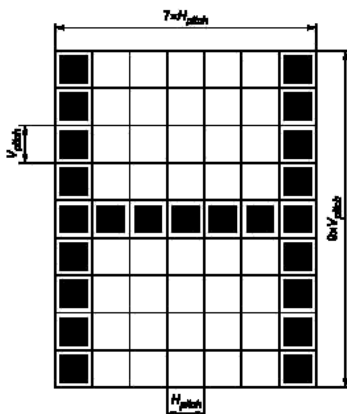
Рисунок 16 — Пример высоты знака
