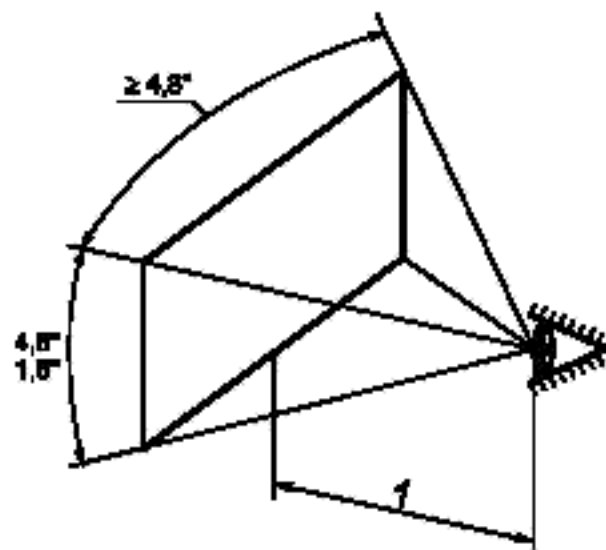
Рисунок 10 — Панель малых размеров
