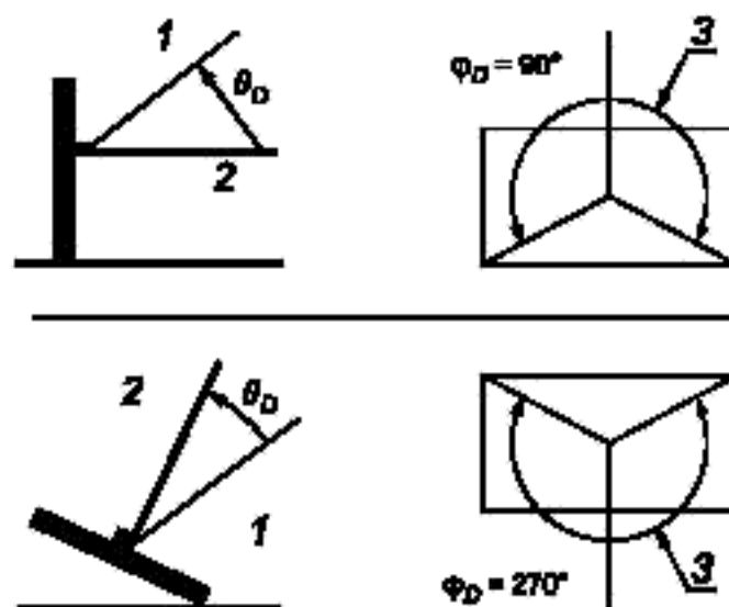
1 — линия визирования; 2 — нормаль; 3 — азимутальный диапазон.
