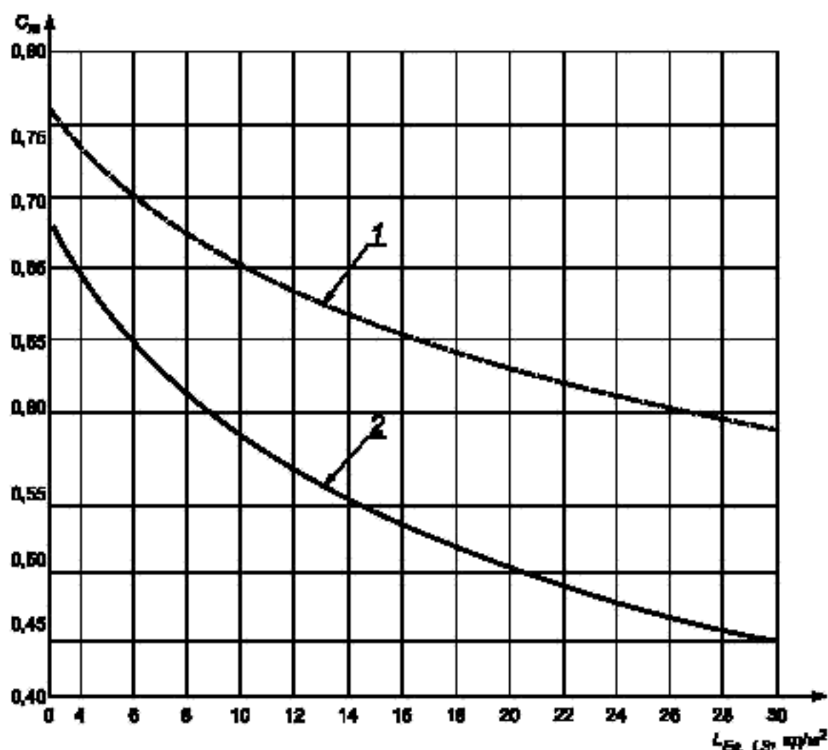
Рисунок 20 — Графическое представление уравнения (21)
