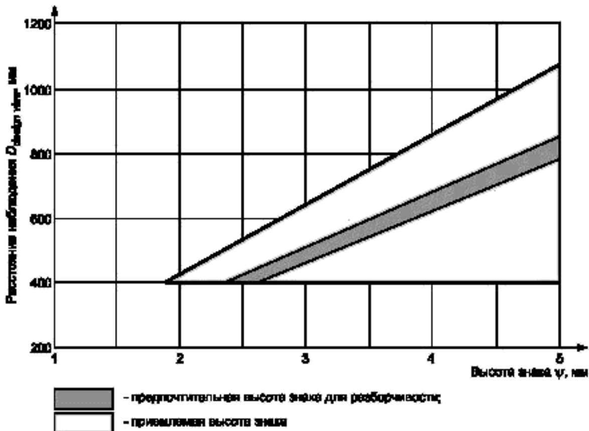
Рисунок 11 — Зависимость «расстояние наблюдения — высота знака»
