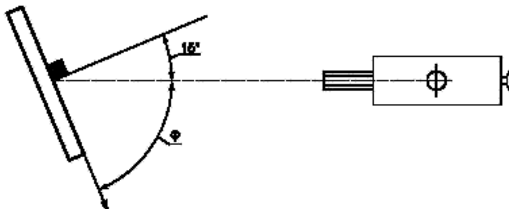
Рисунок 39 — Геометрия измерения для оценки отражения
