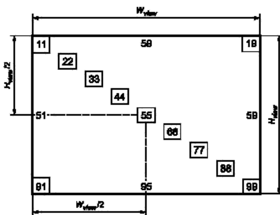
Рисунок 32 — Возможные места измерений
