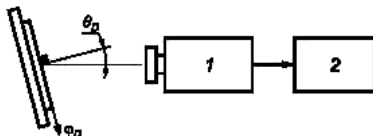
1 — фотометр; 2 — обработка данных
