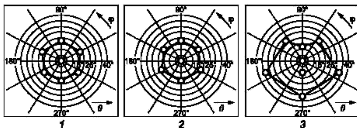
1 — альбомная ориентация, \varphi_D = 90^\circ , \theta_D = 0^\circ и \varphi_C = 63,4^\circ (таблица 33); 2 — альбомная ориентация, \varphi_D = 270^\circ , \theta_D = 0^\circ и \varphi_C = 63,4^\circ (таблица 34); 3 — портретная ориентация, \varphi_D = 270^\circ , \theta_D = 10^\circ и \varphi_C = 71,6^\circ (таблица 35)
