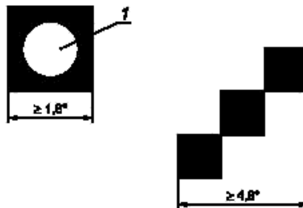
1 — фотометрируемое изображение с угловым размером 1^\circ
