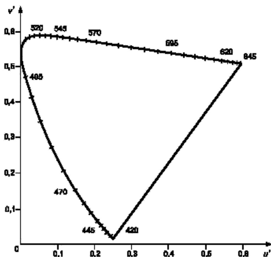
Рисунок 1 — равноконтрастный цветовой график МКО 1976
