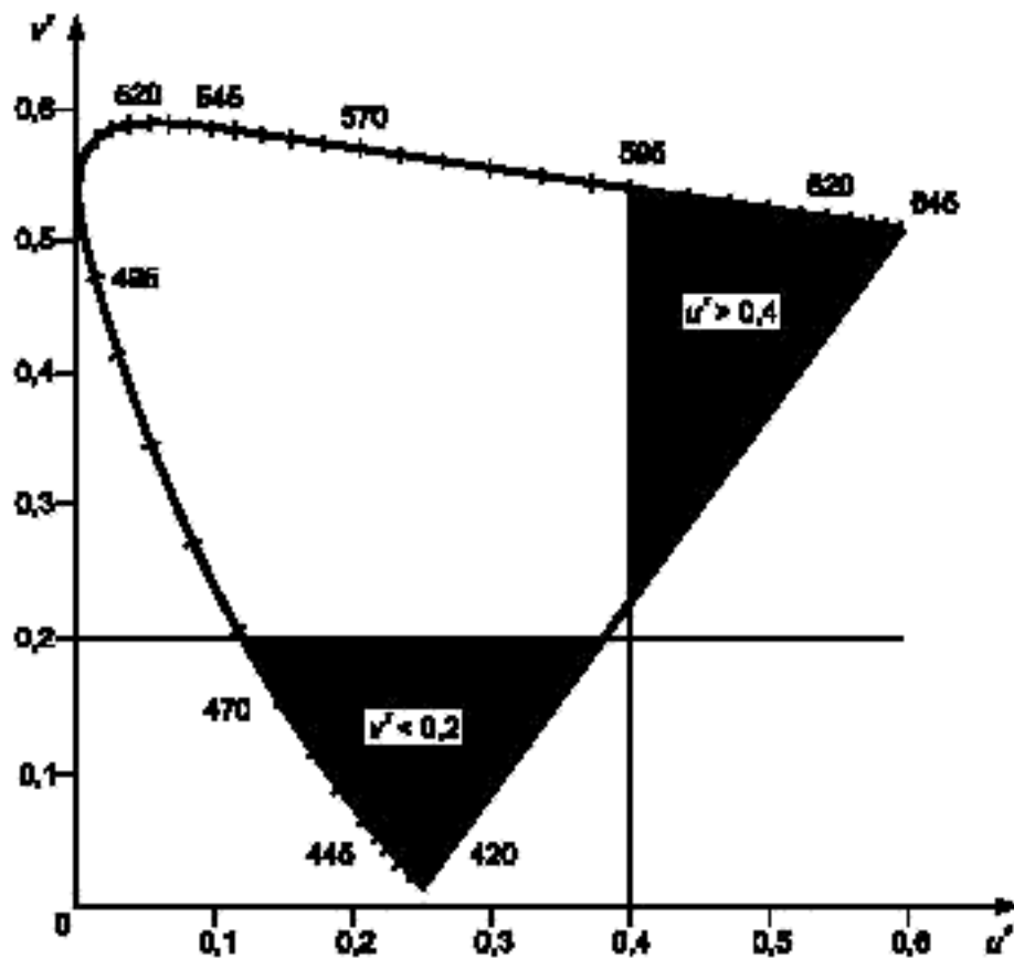
Рисунок 2 — Предельный красный и предельный синий цвета
