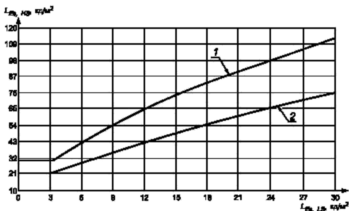
Рисунок 18 — Графическое представление уравнения (22)
